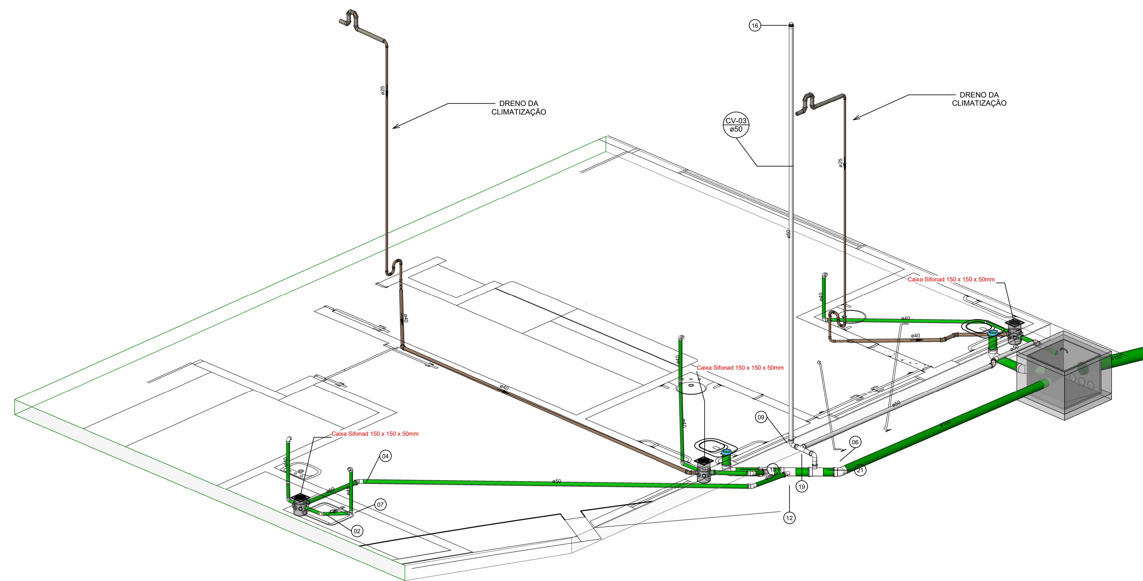
DETALHAMENTO 05 Escala
