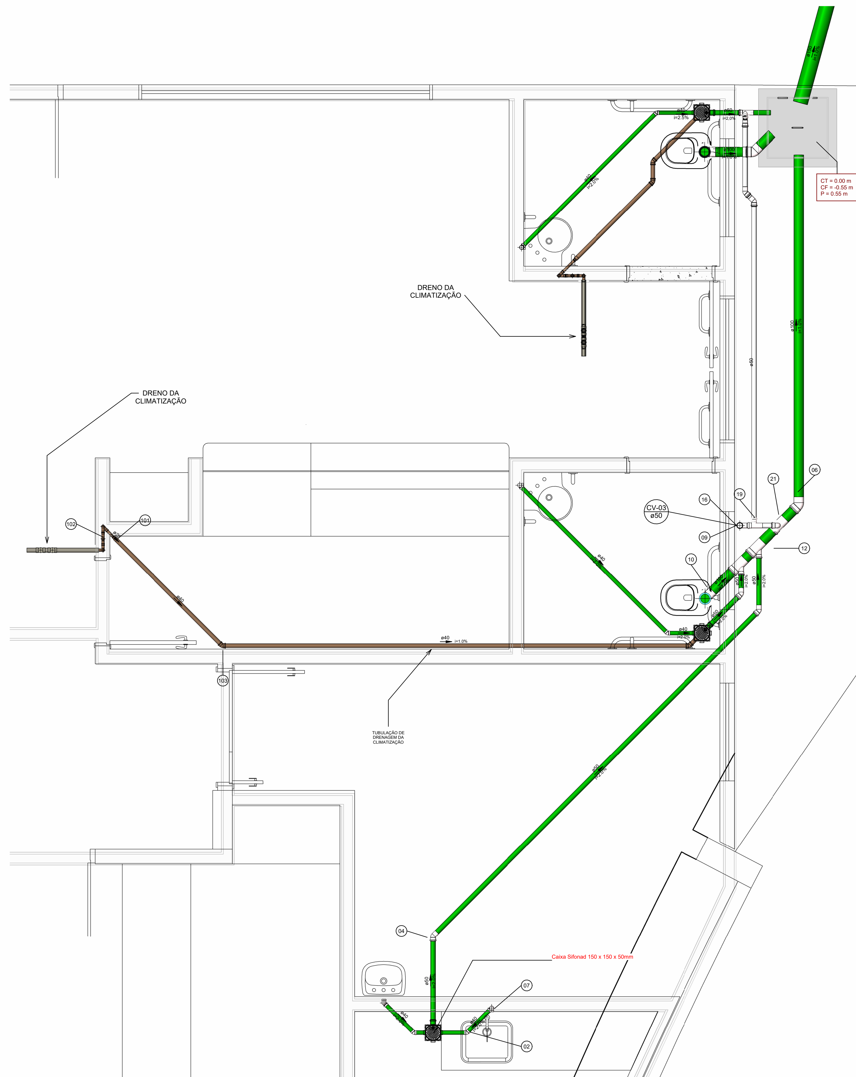
DETALHAMENTO 05 Escala 1 : 20
