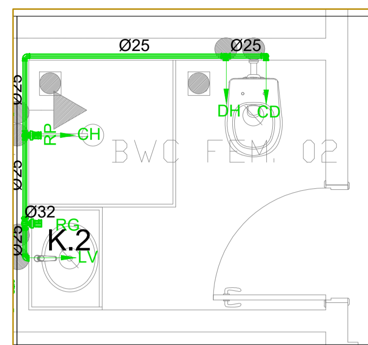
DET.04 Escala 1 : 25
