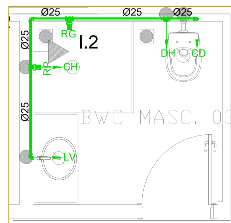
DET.08 Escala 1 : 25
