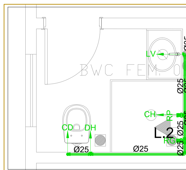
DET.03 Escala 1 : 25
