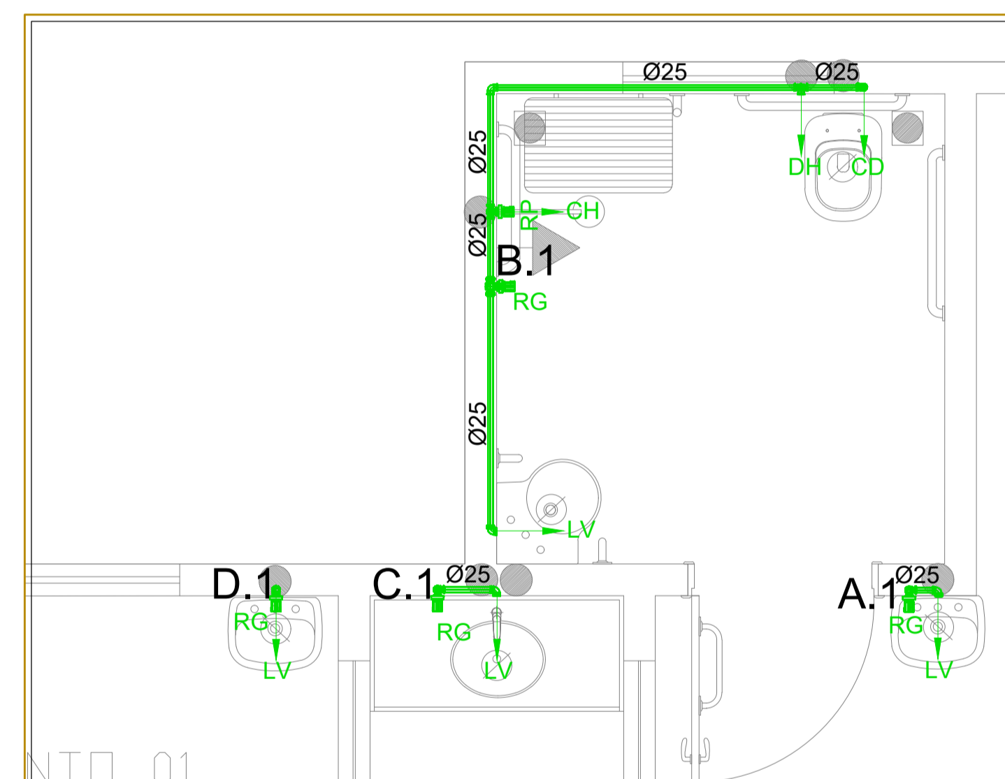
DET.09 Escala 1 : 25
