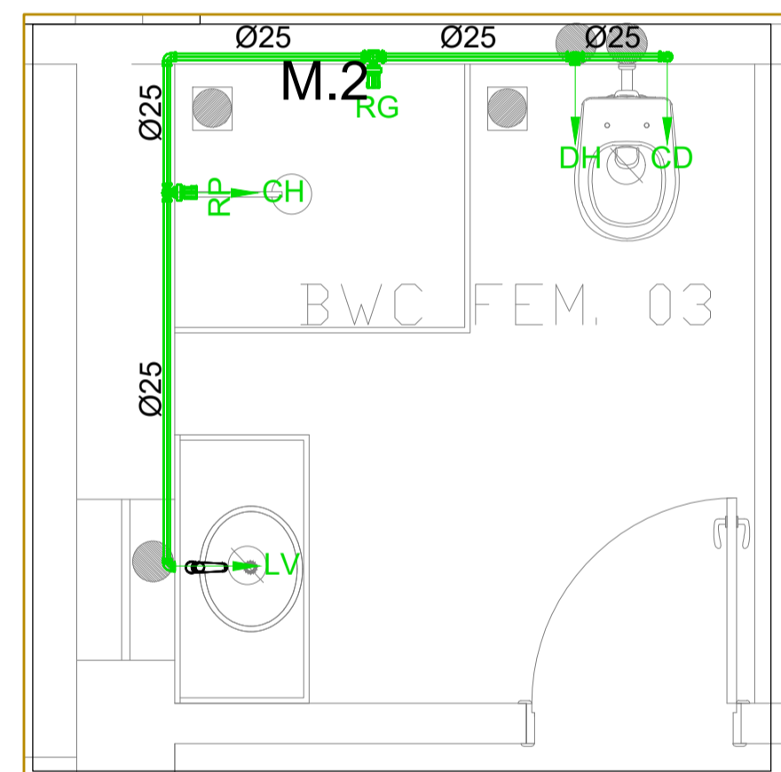
DET.06 Escala 1 : 25
