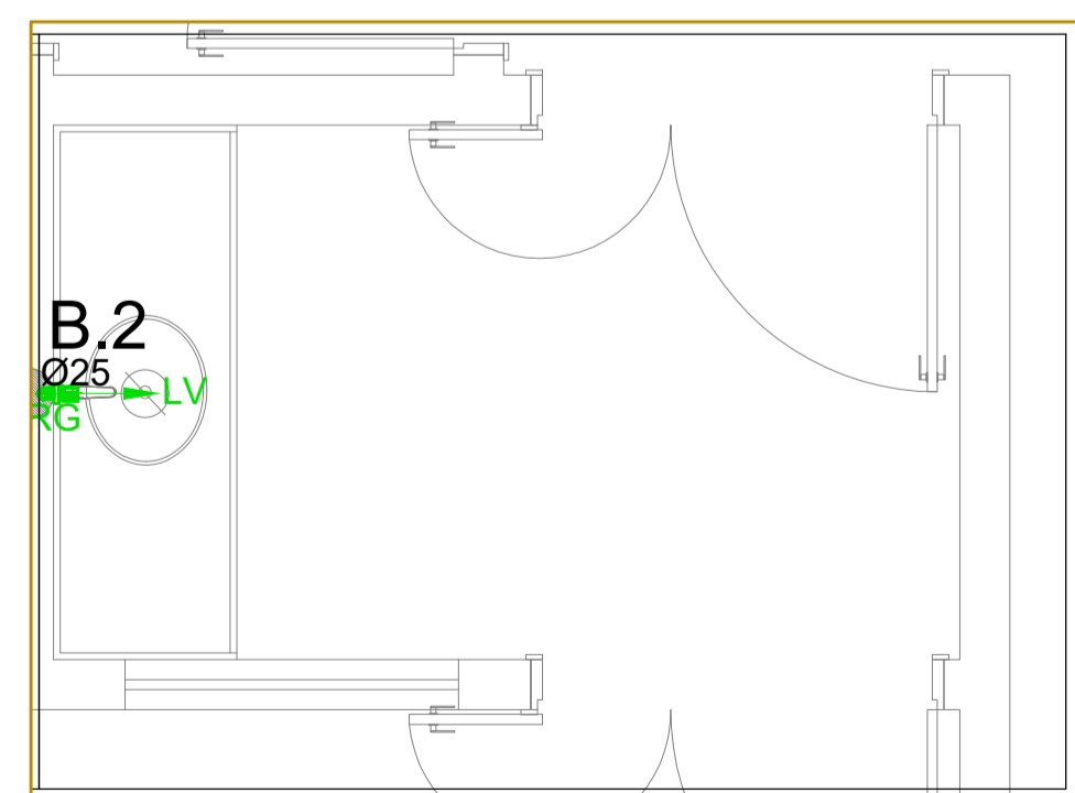
DET.11 Escala 1 : 25
