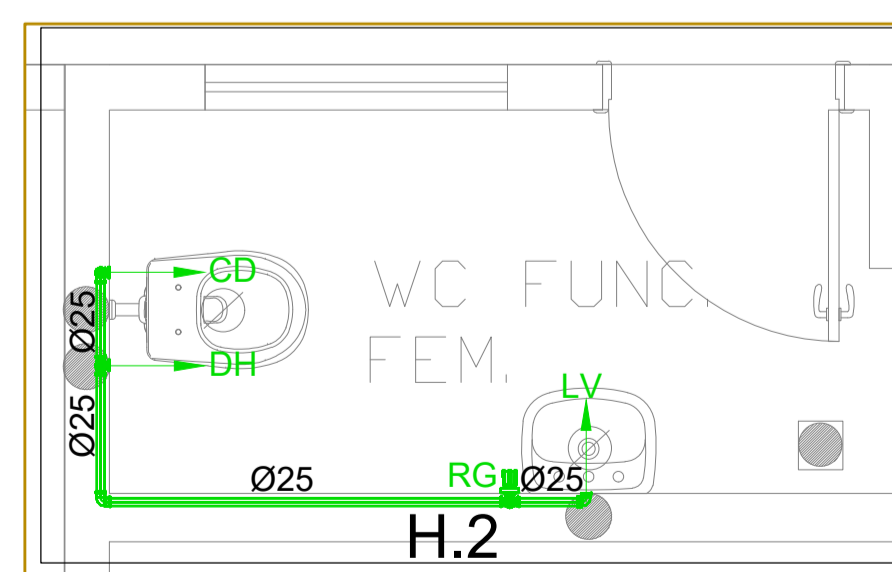
DET.12 Escala 1 : 25
