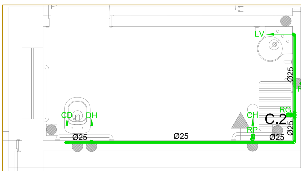
DET.10 Escala 1 : 25
