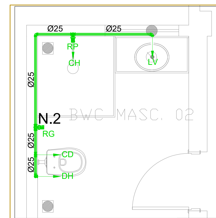
DET.05 Escala 1 : 25
