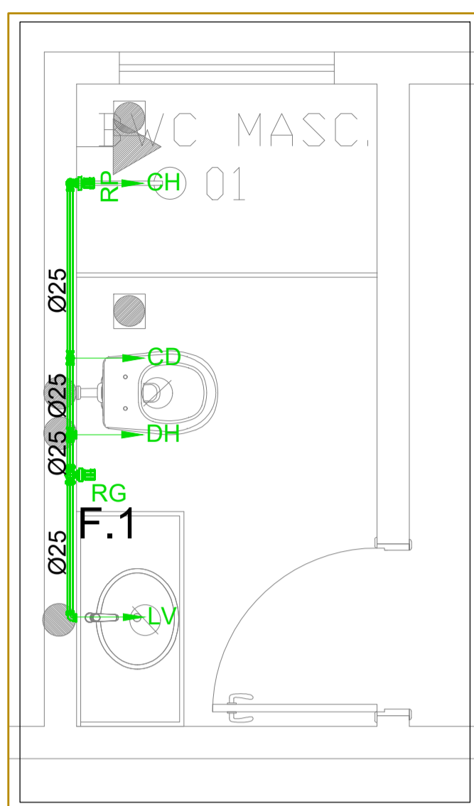
DET.01 Escala 1 : 25
