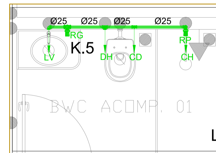
DET.21 Escala 1:25
