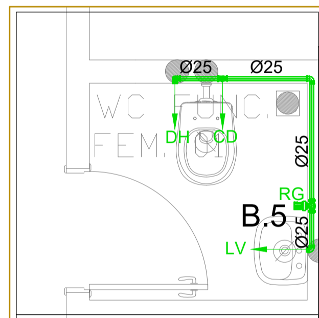
DET.18 Escala 1:25
