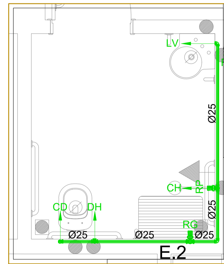
DET.14 Escala 1:25
