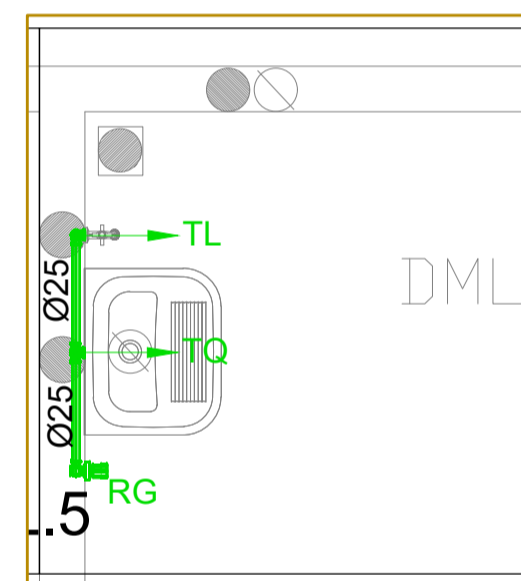
DET.22 Escala 1:25
