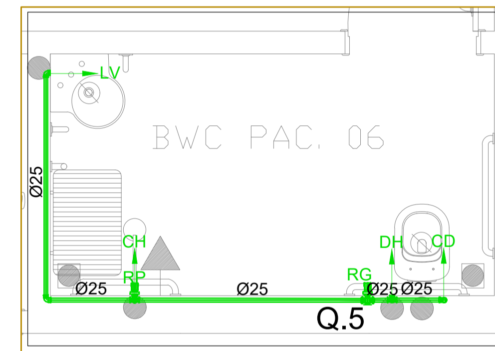
DET.23 Escala 1:25
