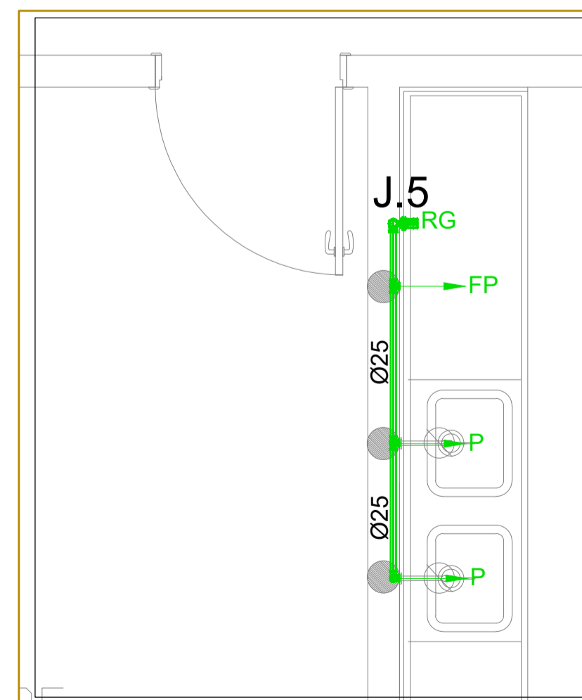
DET.25 Escala 1:25
