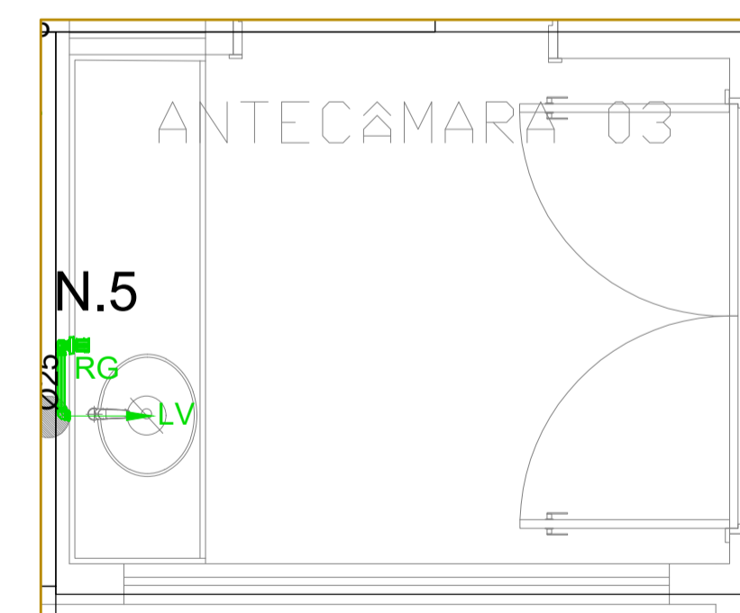
DET.28 Escala 1:25
