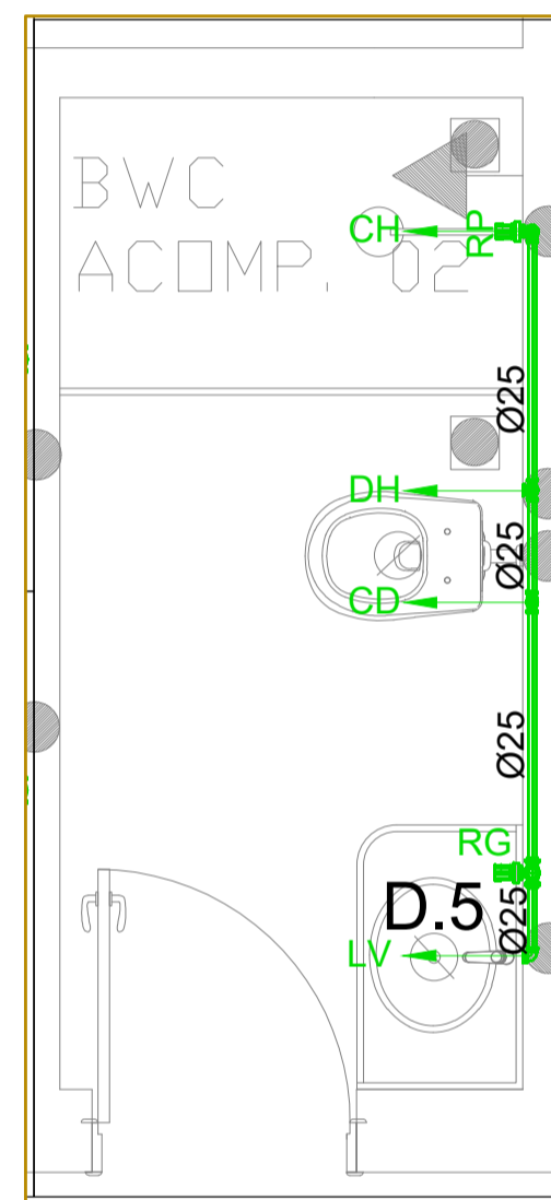
DET.19 Escala 1:25
