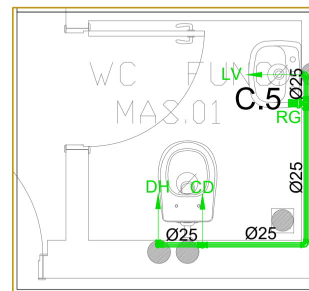
DET.20 Escala 1:25
