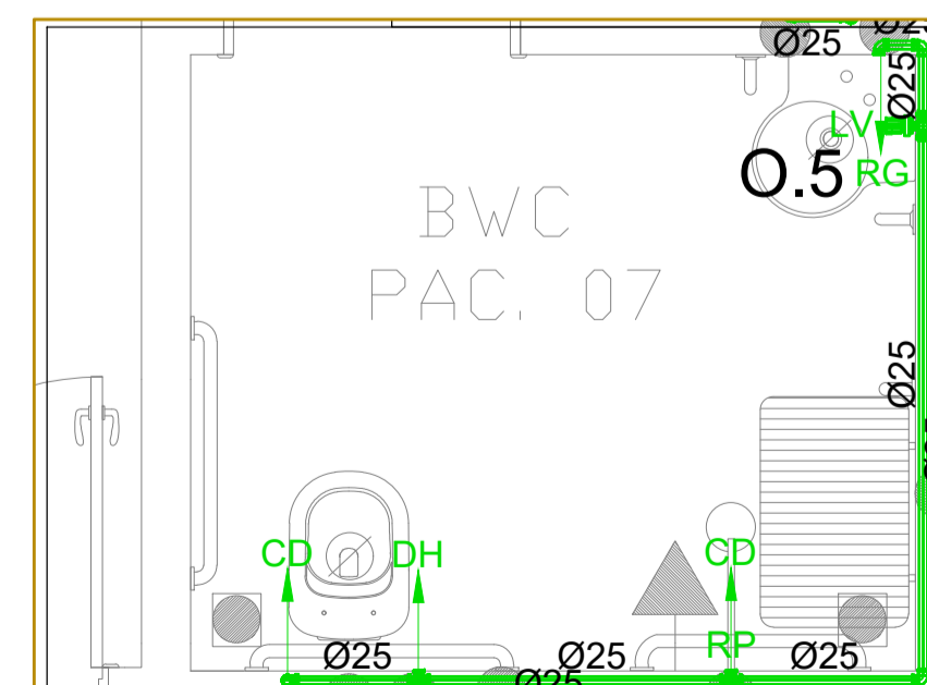
DET.27 Escala 1:25
