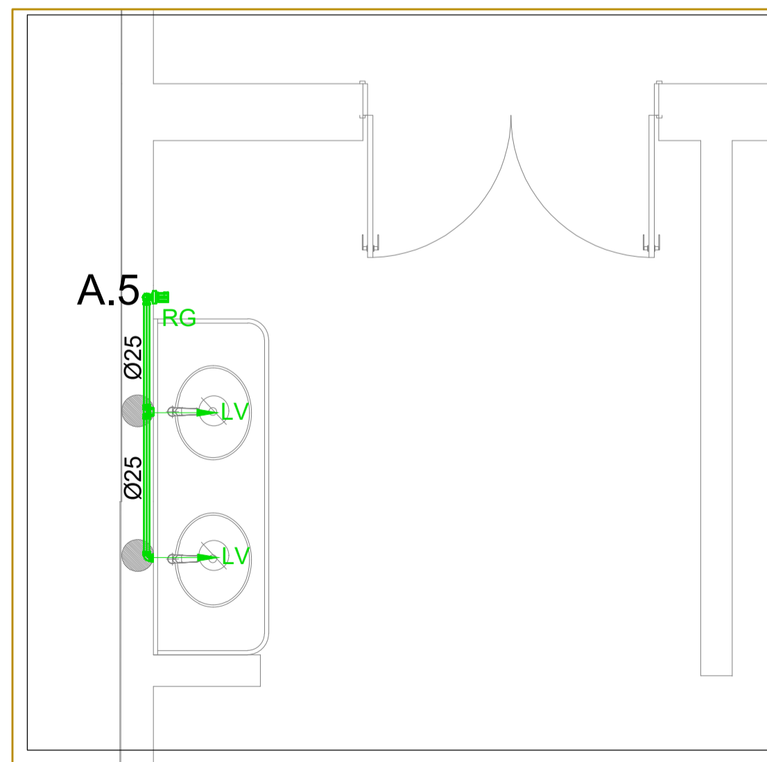
DET.24 Escala 1:25
