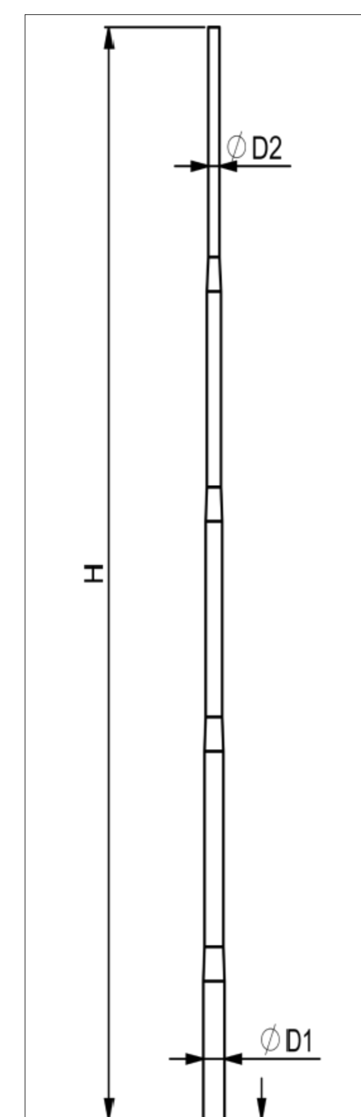
DETALHE 03 - DIMENSÕES DO POSTE CFTV
