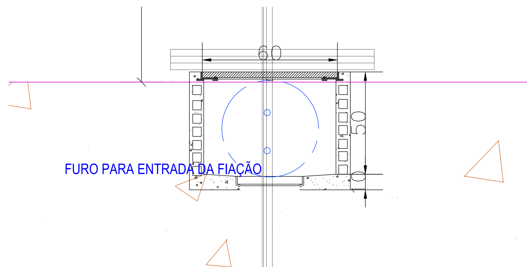
DETALHE 01 - BASE POSTE
