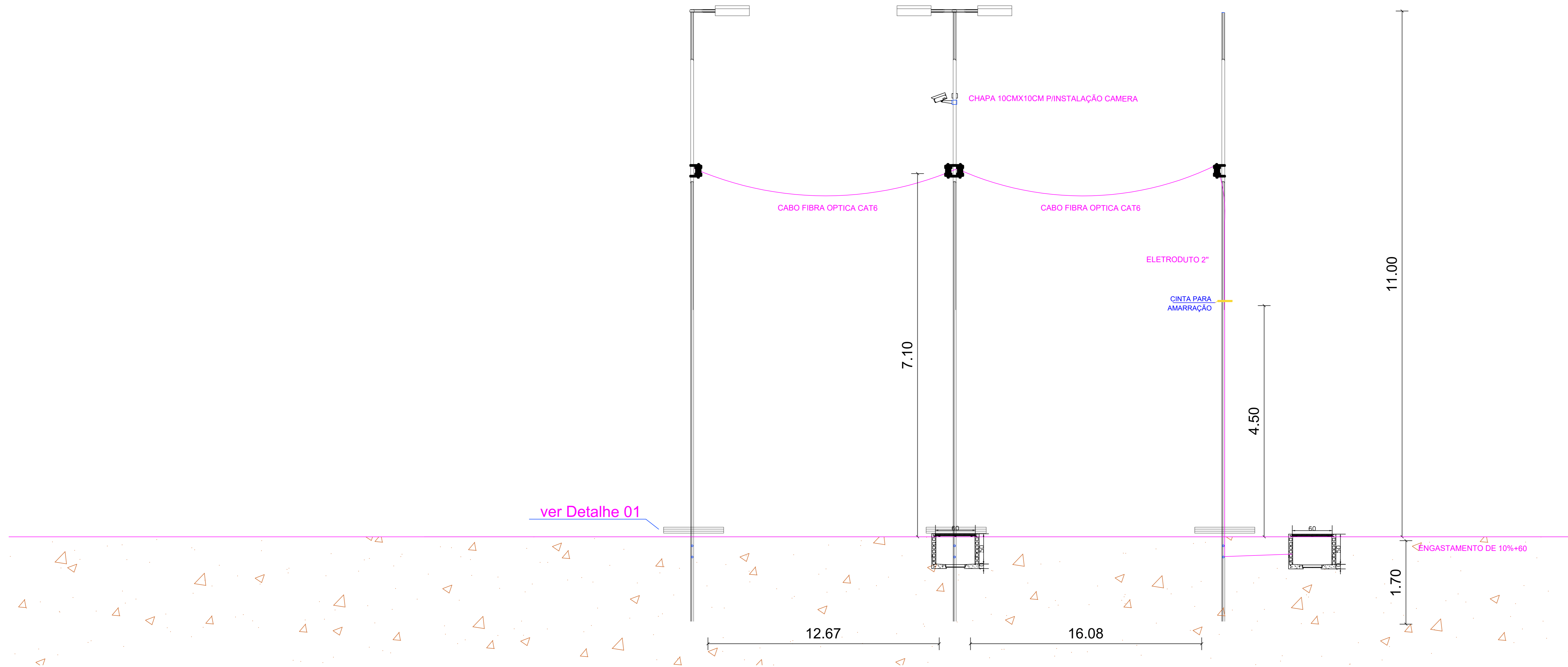
VISTA LATERAL - POSTES DE TELECOMUNICAÇÕES
