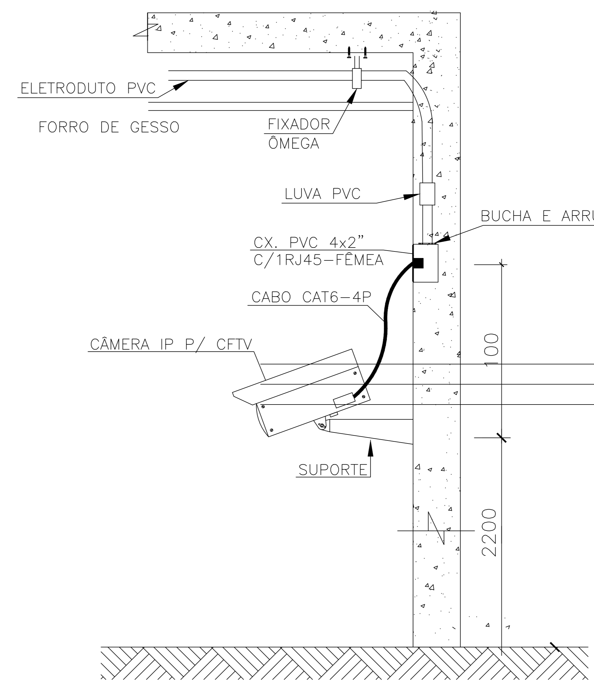
DETALHE 04 - INSTALAÇÃO CFTV EM PAREDE
