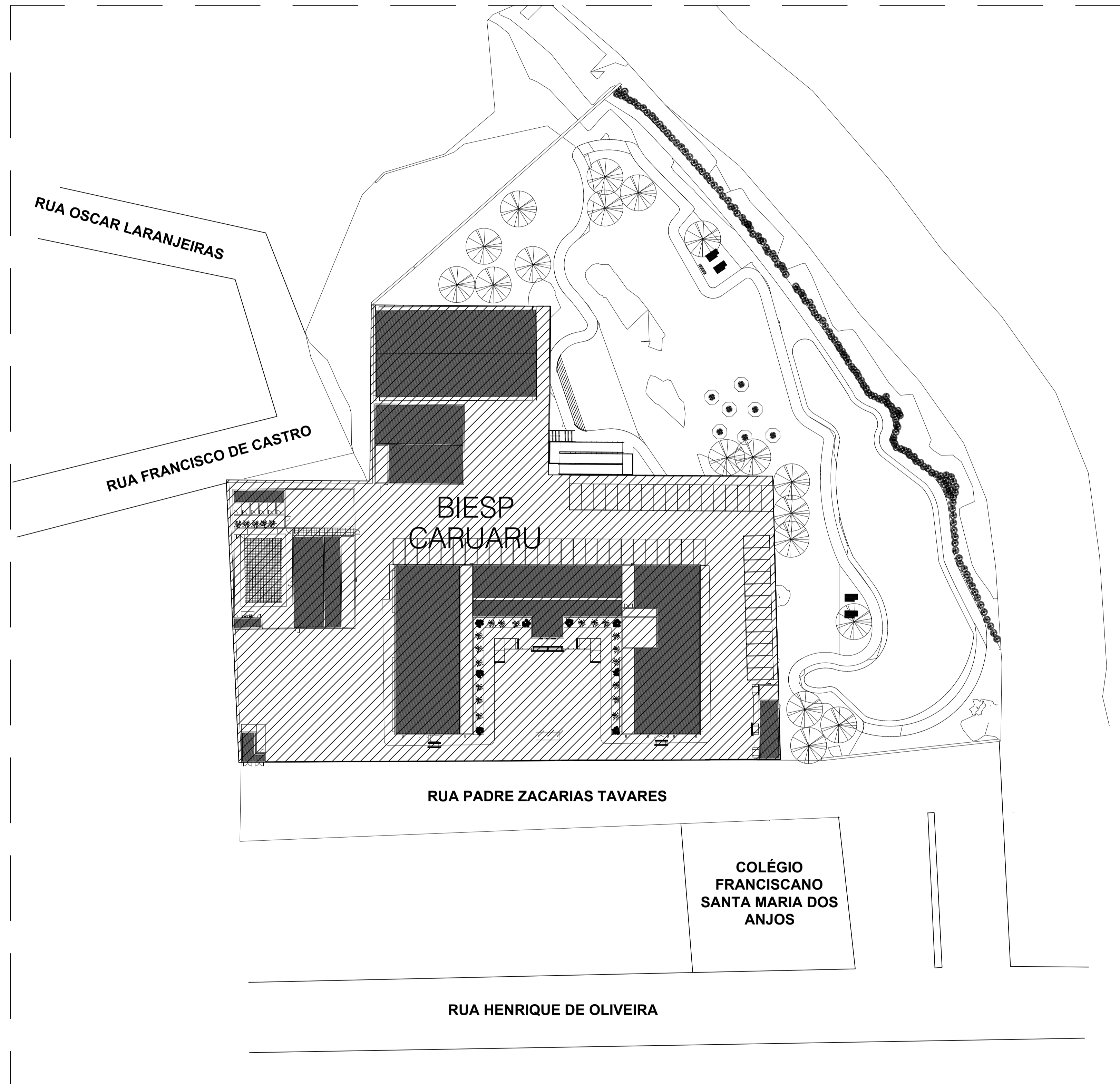
01 SUBESTAÇÃO AÉREA 13,8 kV - 300 kVA PLANTA DE SITUAÇÃO ESCALA: 1 / 500
