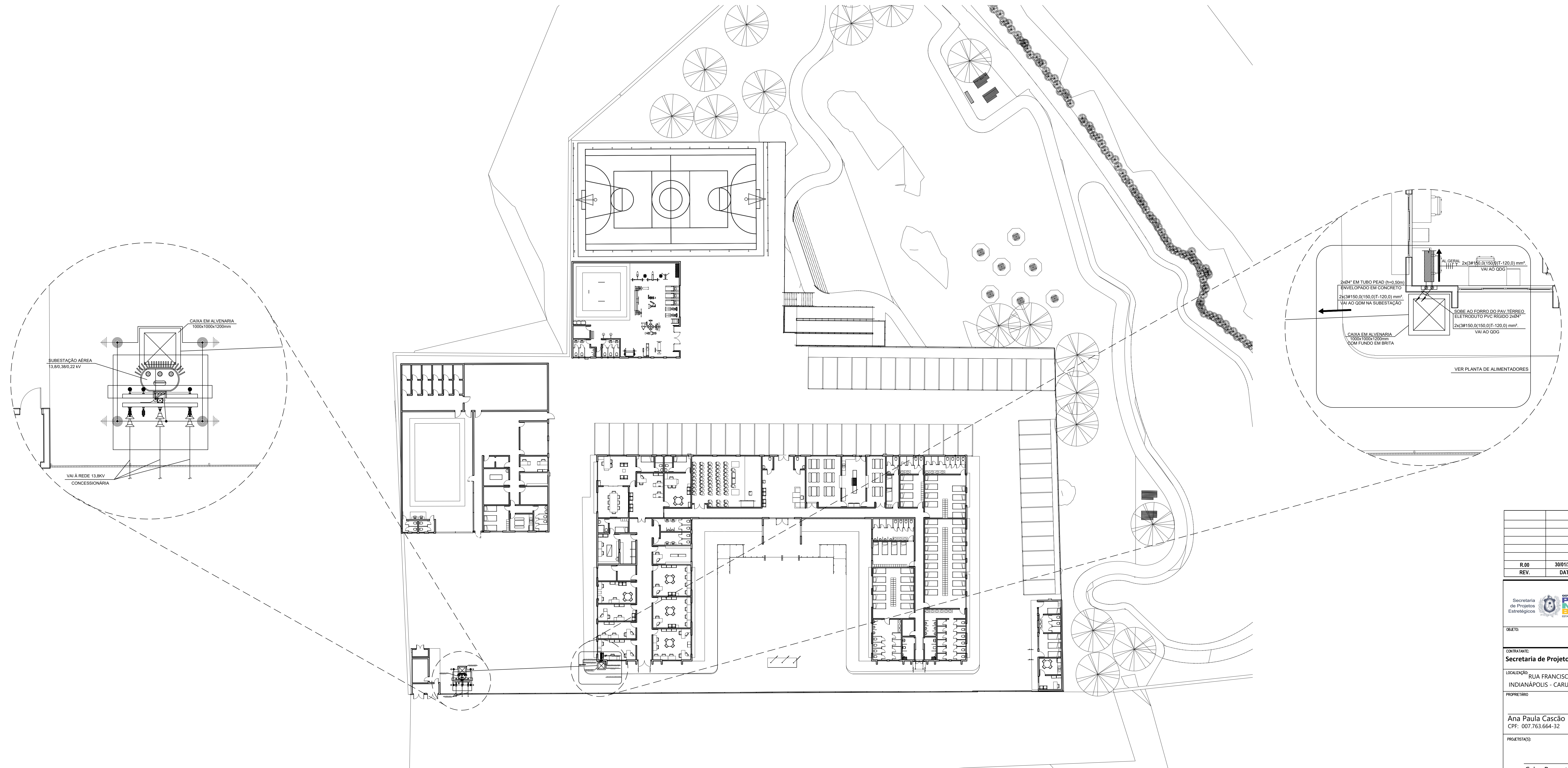
01 SUBESTAÇÃO AÉREA 13,8 kV - 300 KVA PLANTA DE LOCAÇÃO ESCALA: 1 / 500
