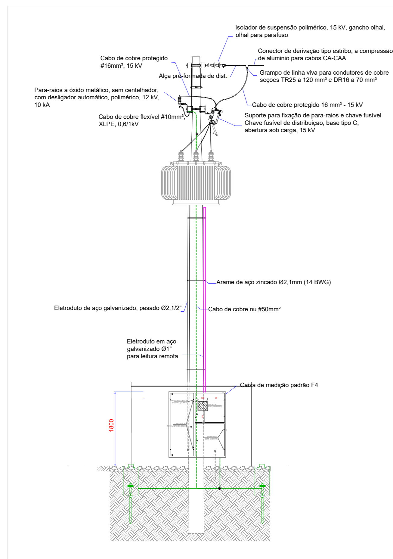
VISTA LATERAL ESCALA: 1/50
