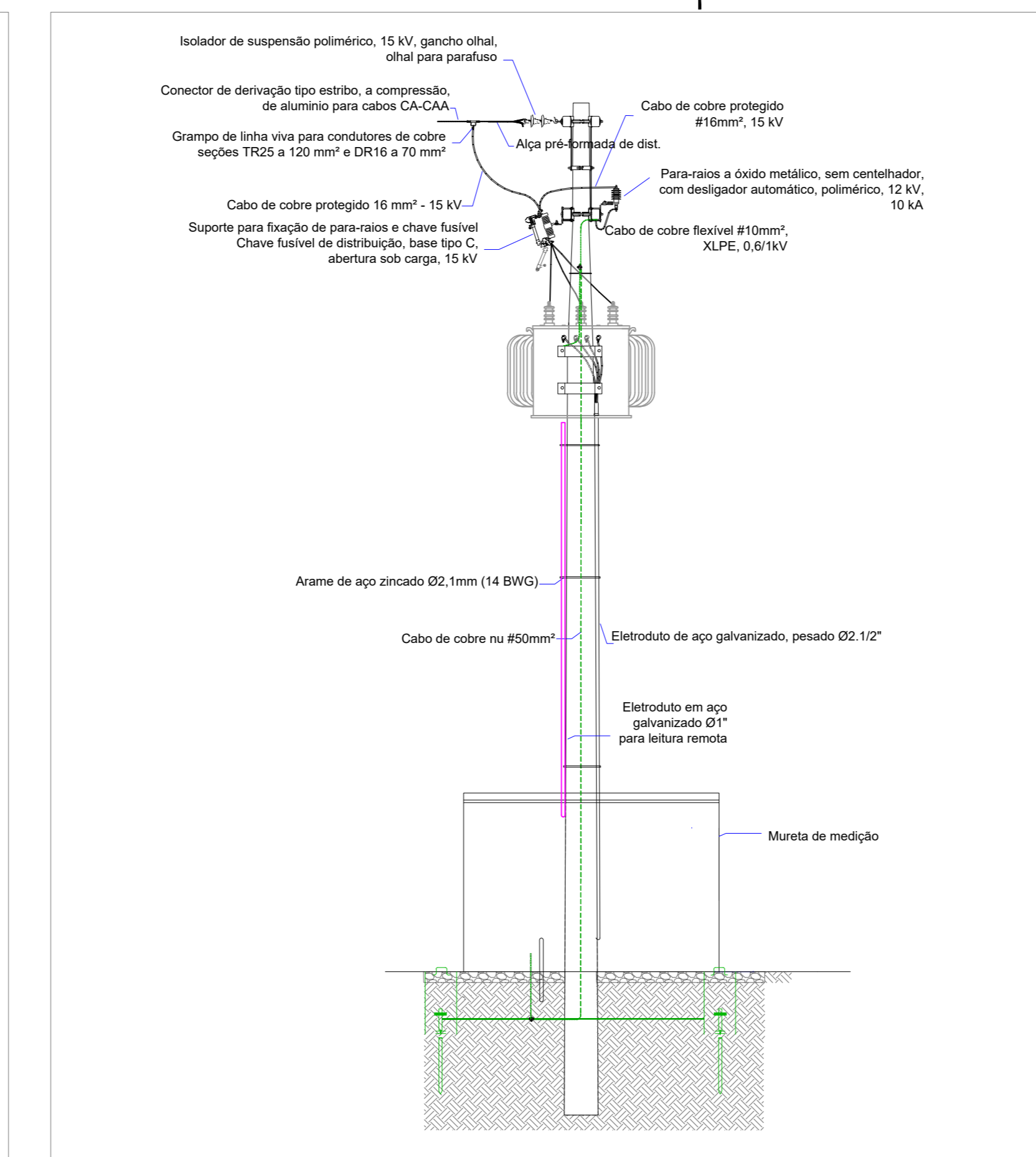
VISTA POSTERIOR ESCALA: 1/50
