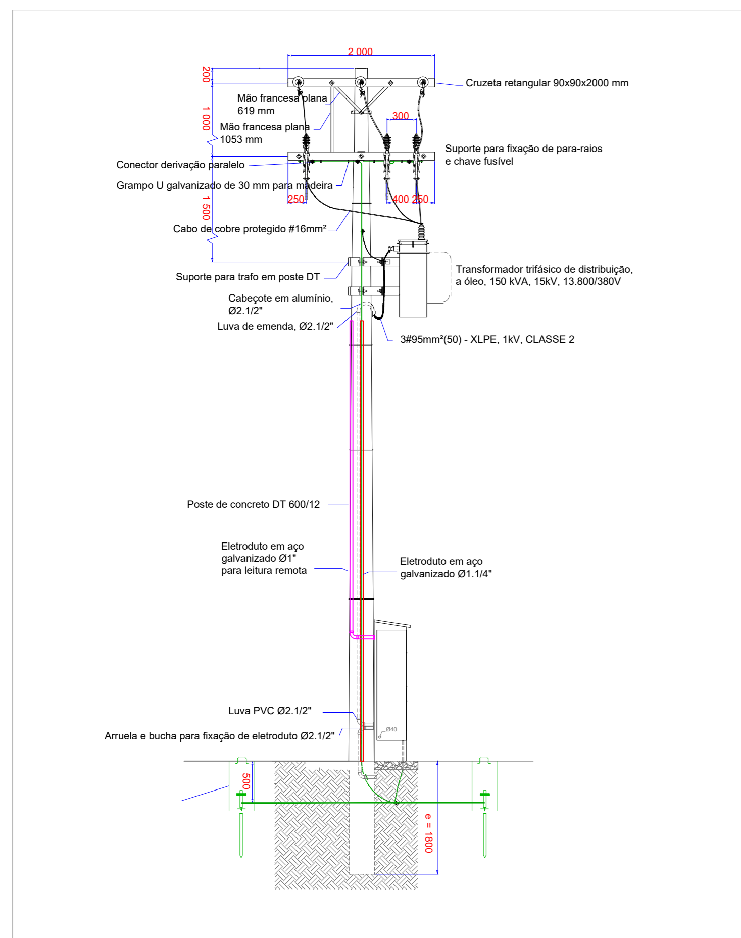
VISTA FRONTAL ESCALA: 1/50
