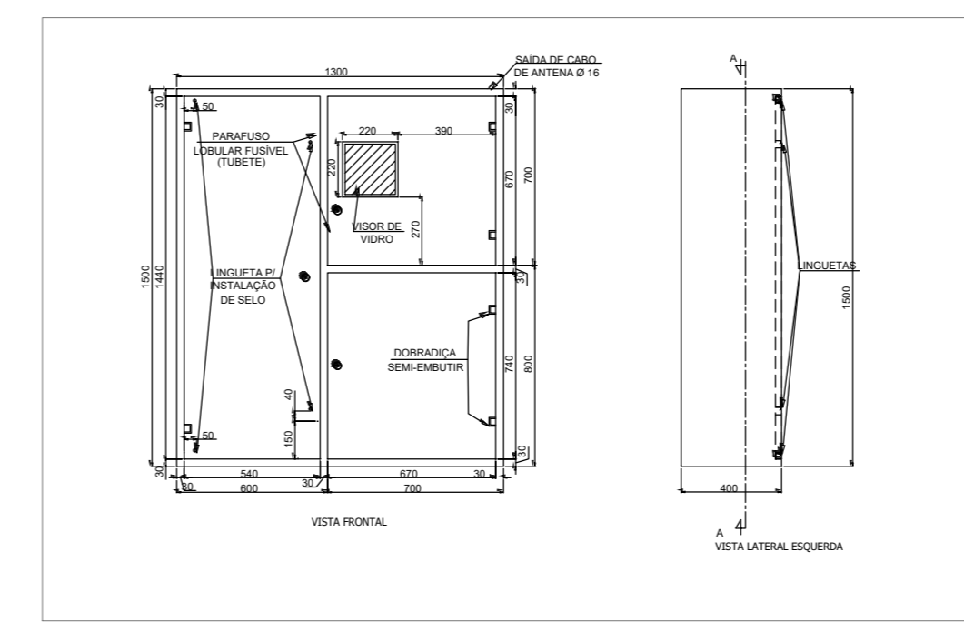
DETALHE CAIXA DE MEDIÇÃO F4 ESCALA: 1/25
