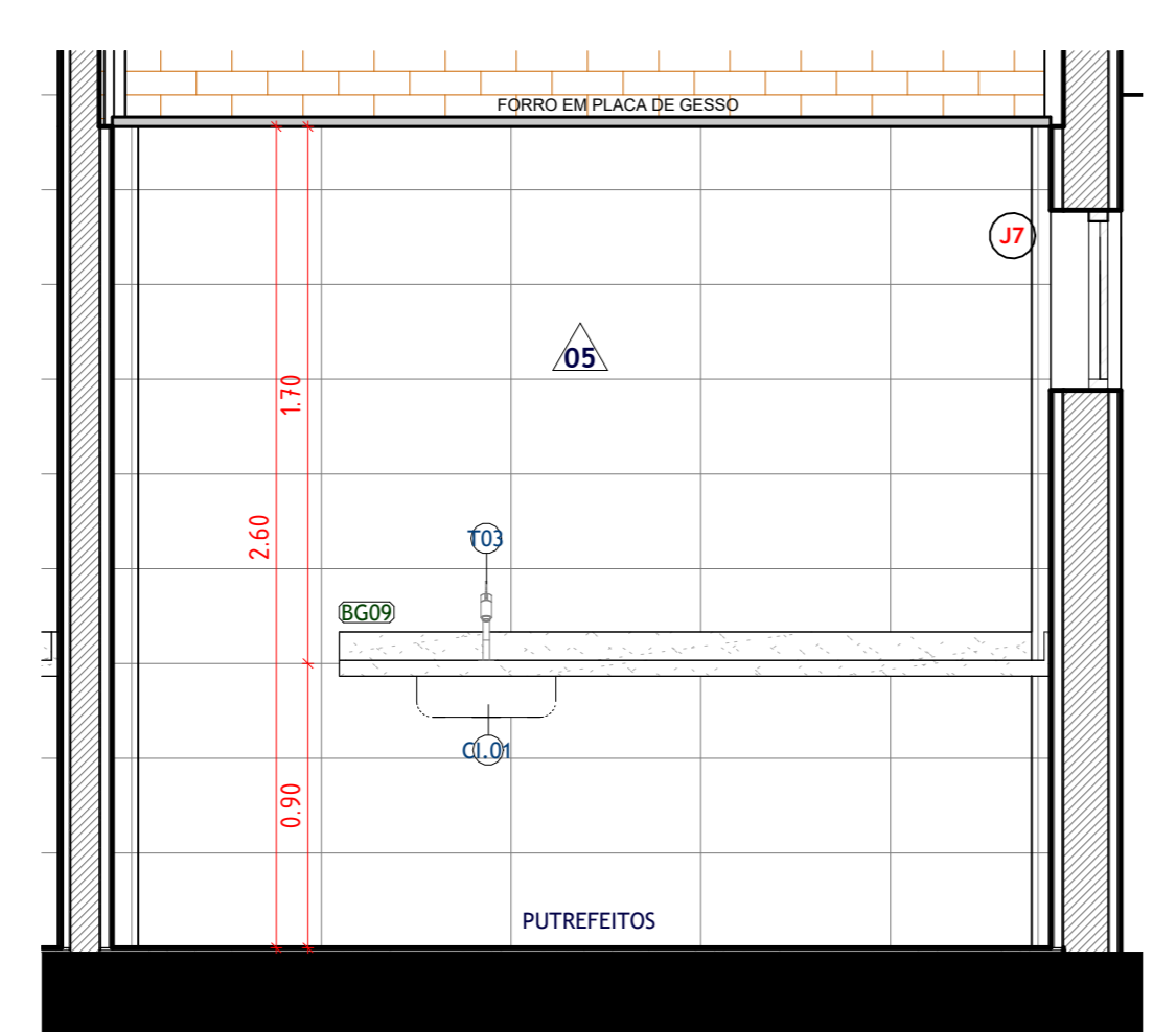
4 D13 - VISTA CC' ESCALA 1:25
