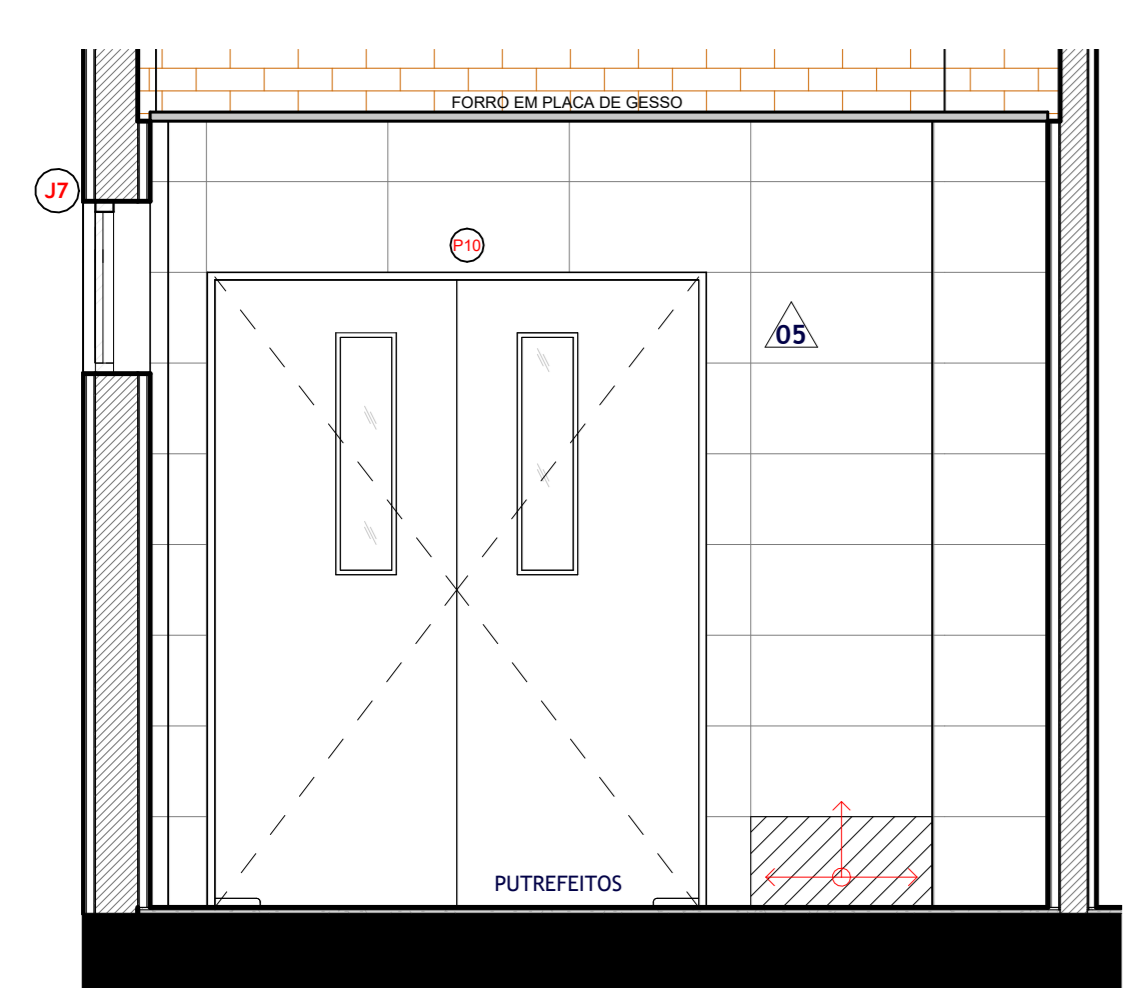
3 D13 - VISTA BB' ESCALA 1:25
