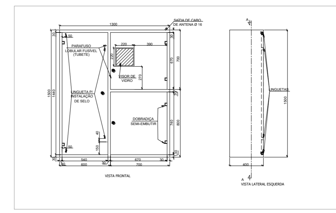
DETALHE CAIXA DE MEDIÇÃO F4 ESCALA: 1/25
