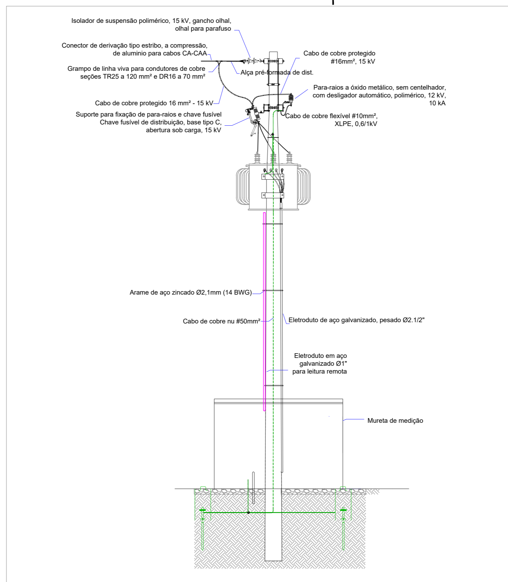
VISTA POSTERIOR ESCALA: 1/50
