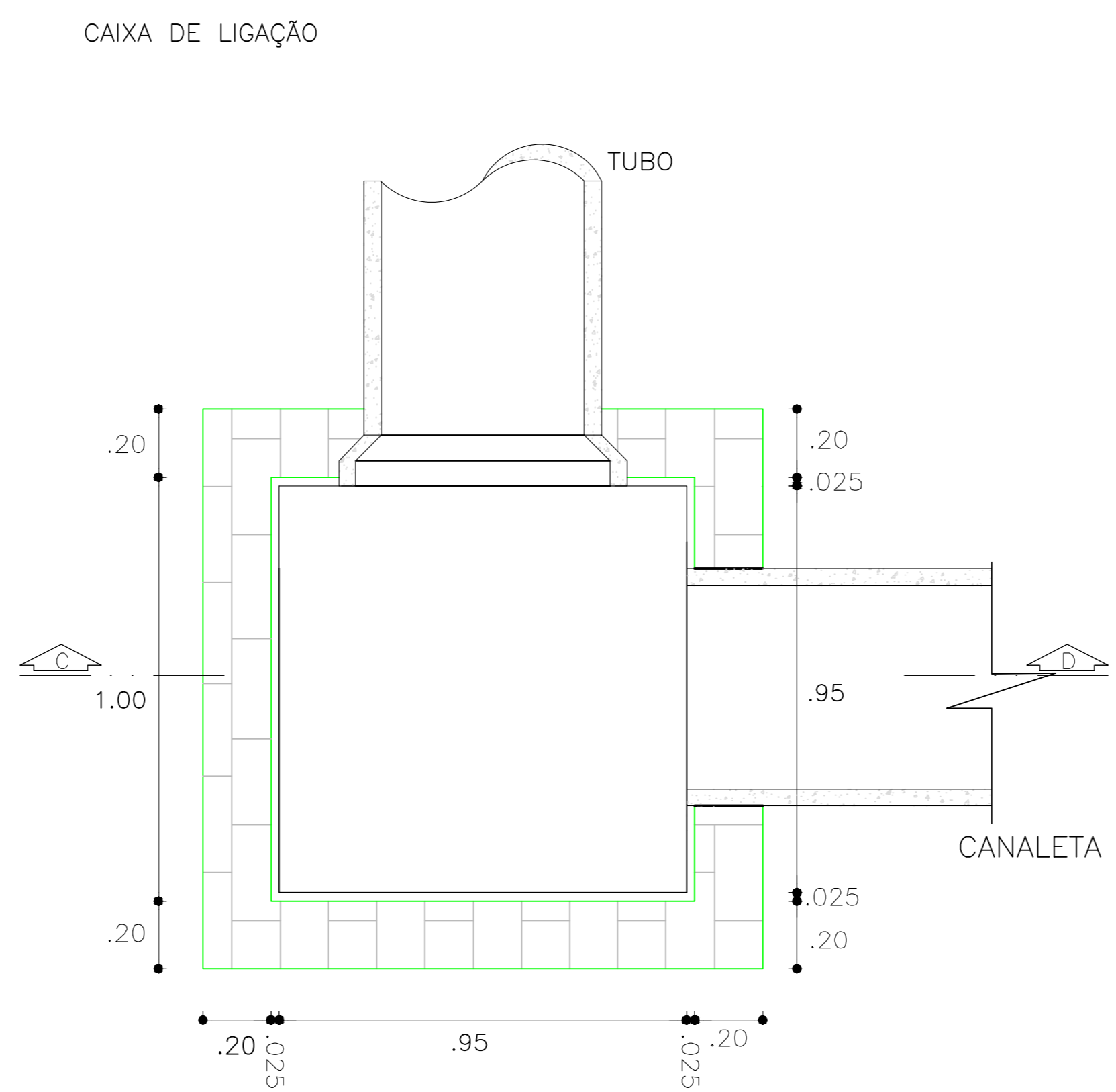
PLANTA BAIXA Sem escala
