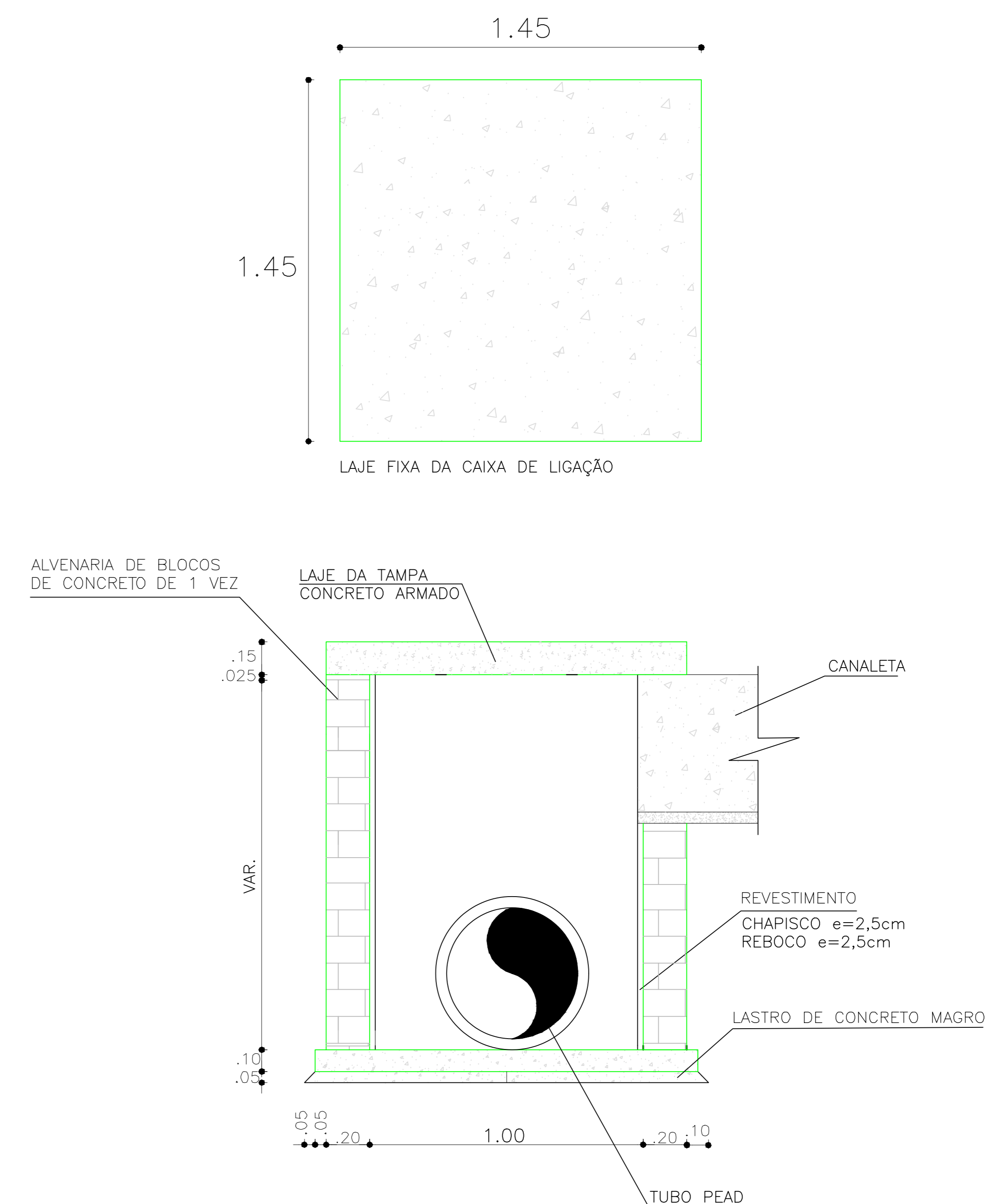
CORTE CD Sem escala
