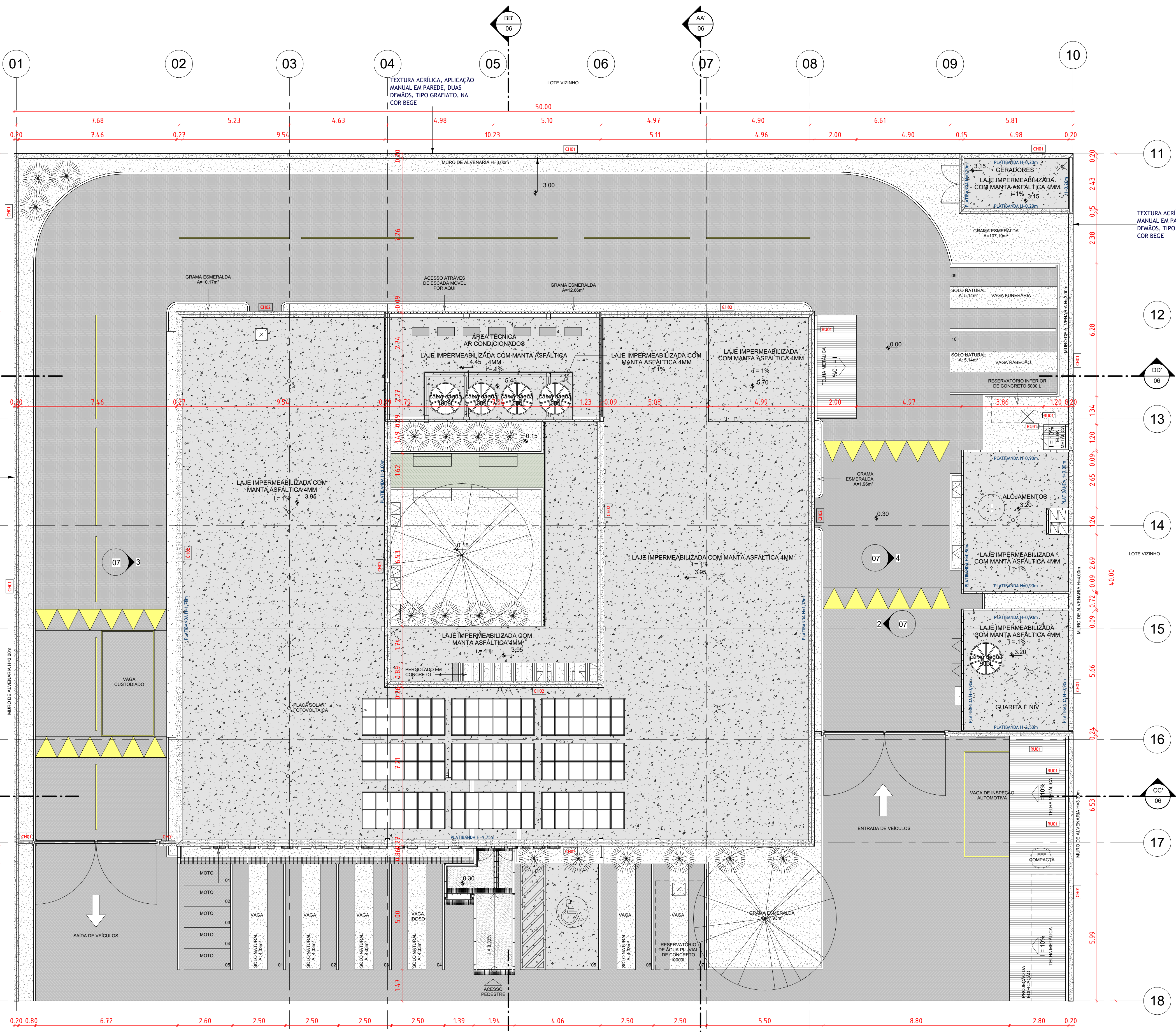
1 PLANTA DE COBERTA ESCALA 1 : 100
