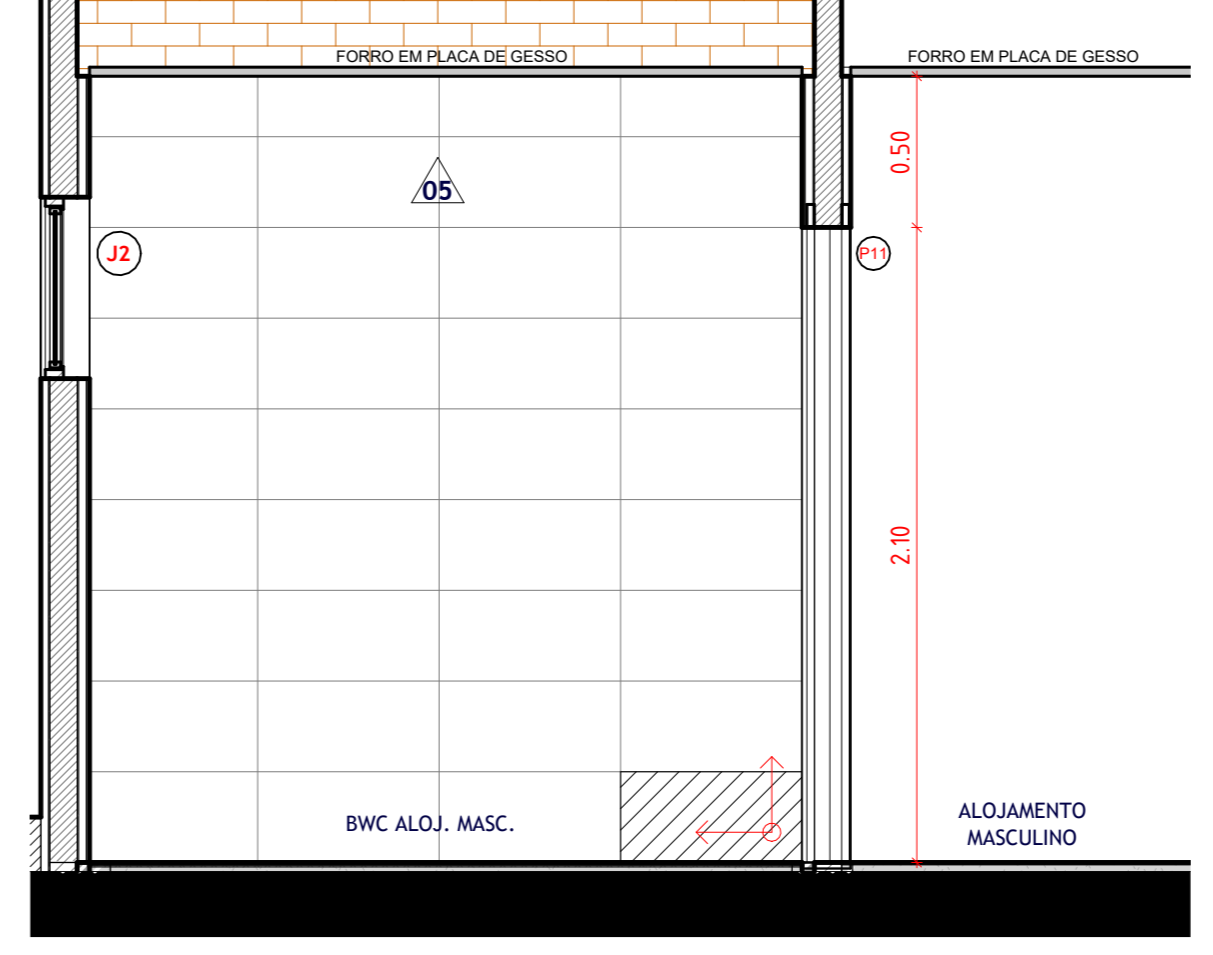
22 D04 - VISTA BB' ESCALA 1:25
