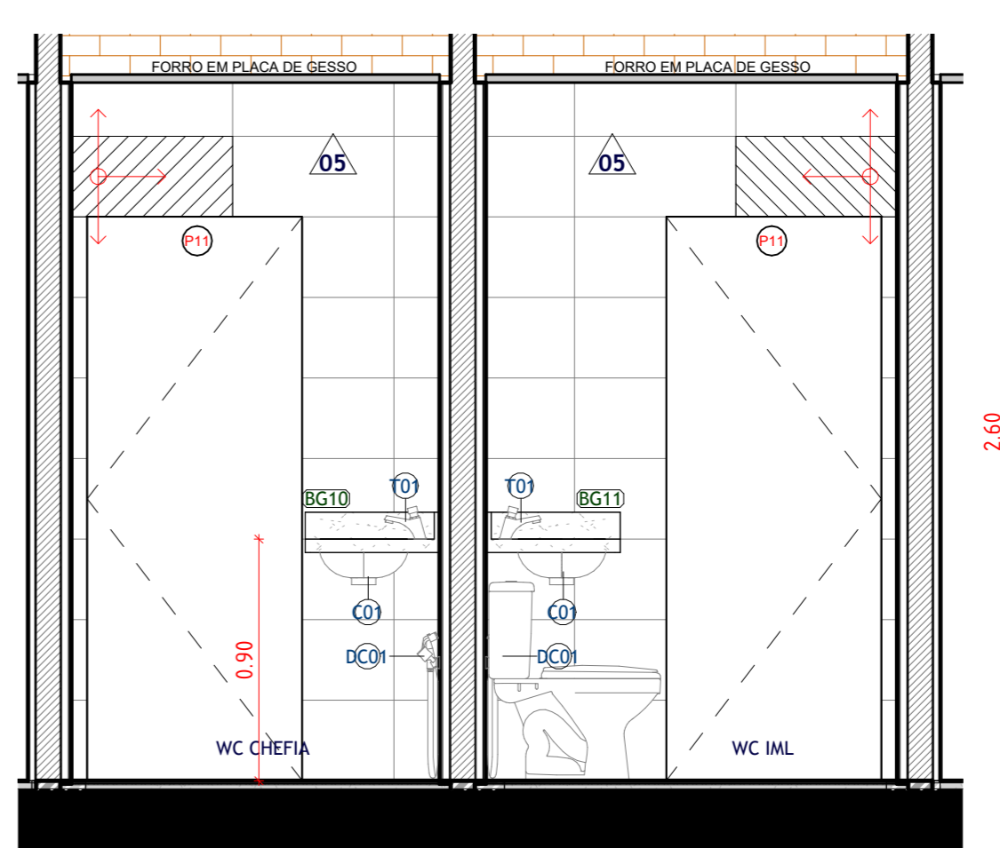
15 D03 - VISTA BB' ESCALA 1:25
