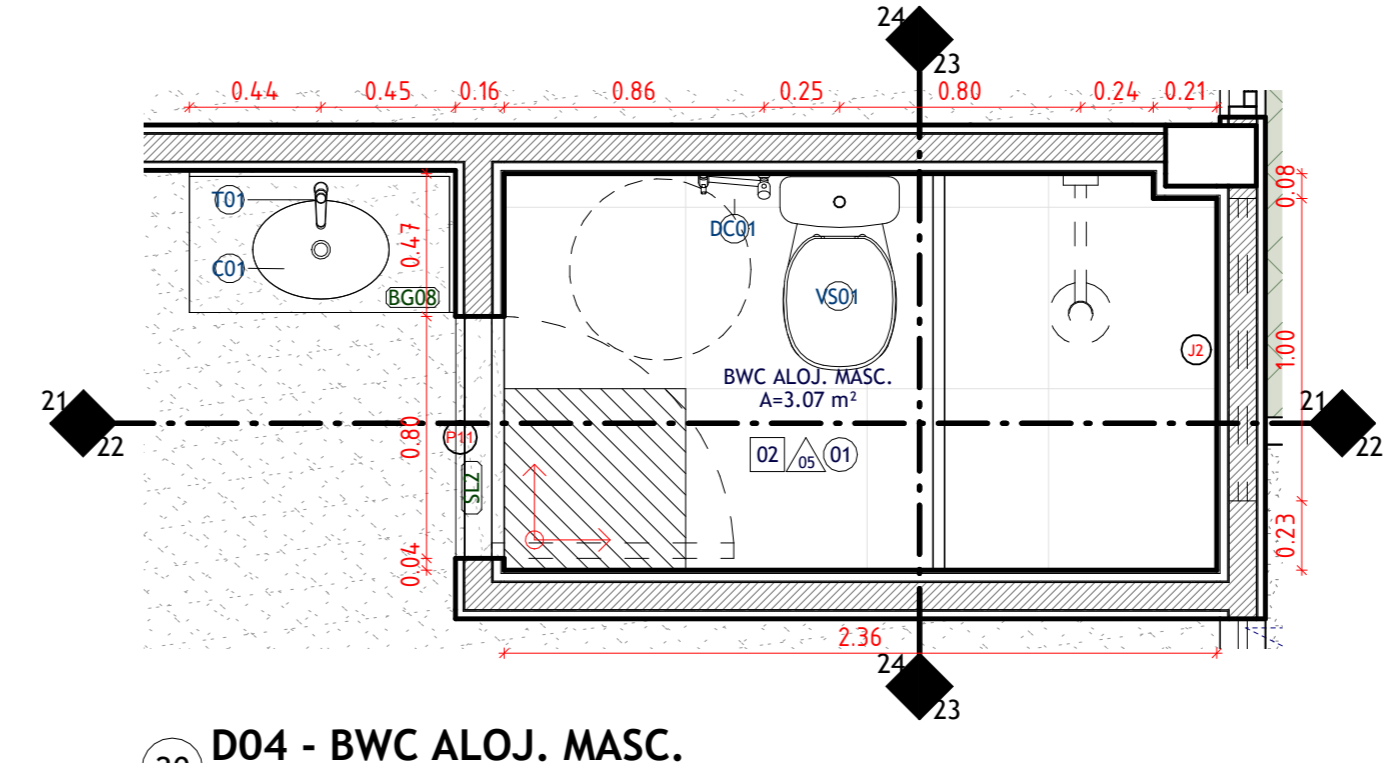
20 D04 - BWC ALOJ. MASC. ESCALA 1:25
