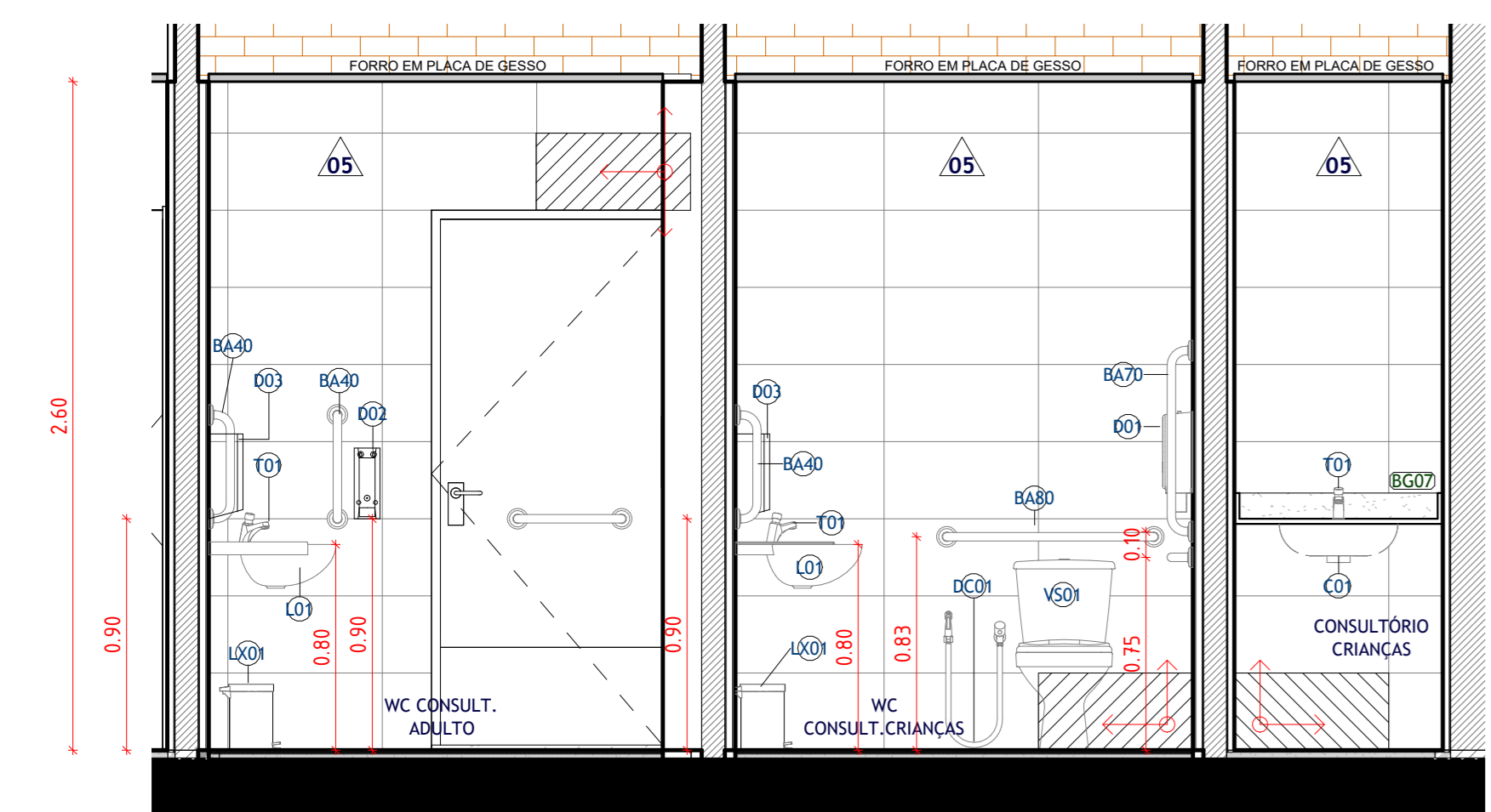
3 D01 - VISTA BB' ESCALA 1:25
