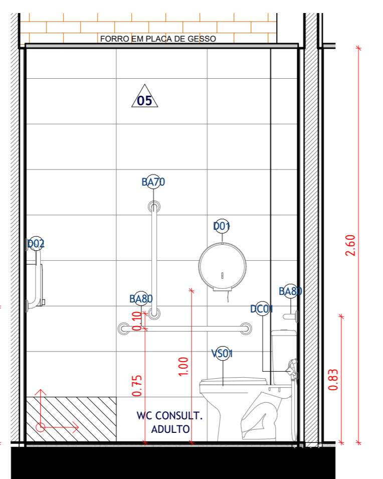
7 D01 - VISTA FF' ESCALA 1:25
