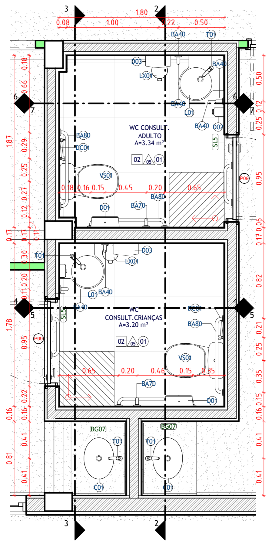
1 D01 - WC CONSULT. ADULTO/ WC CONSULT. CRIANÇA ESCALA 1:25
