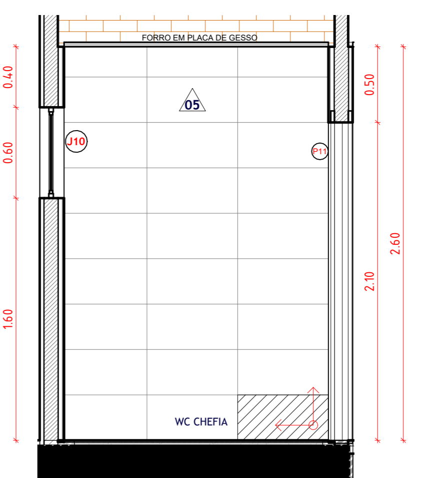
19 D03 - VISTA FF' ESCALA 1:25
