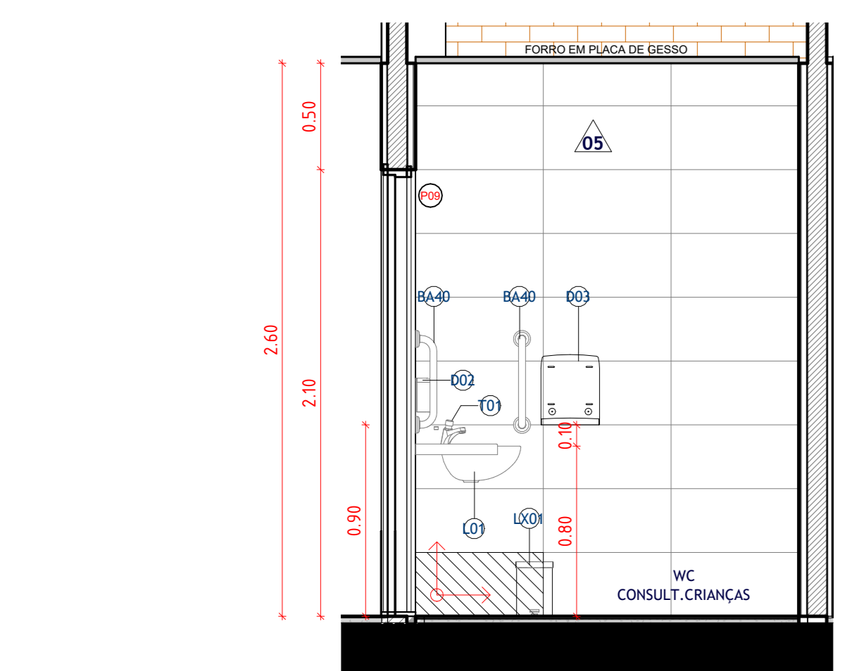
4 D01 - VISTA CC' ESCALA 1:25
