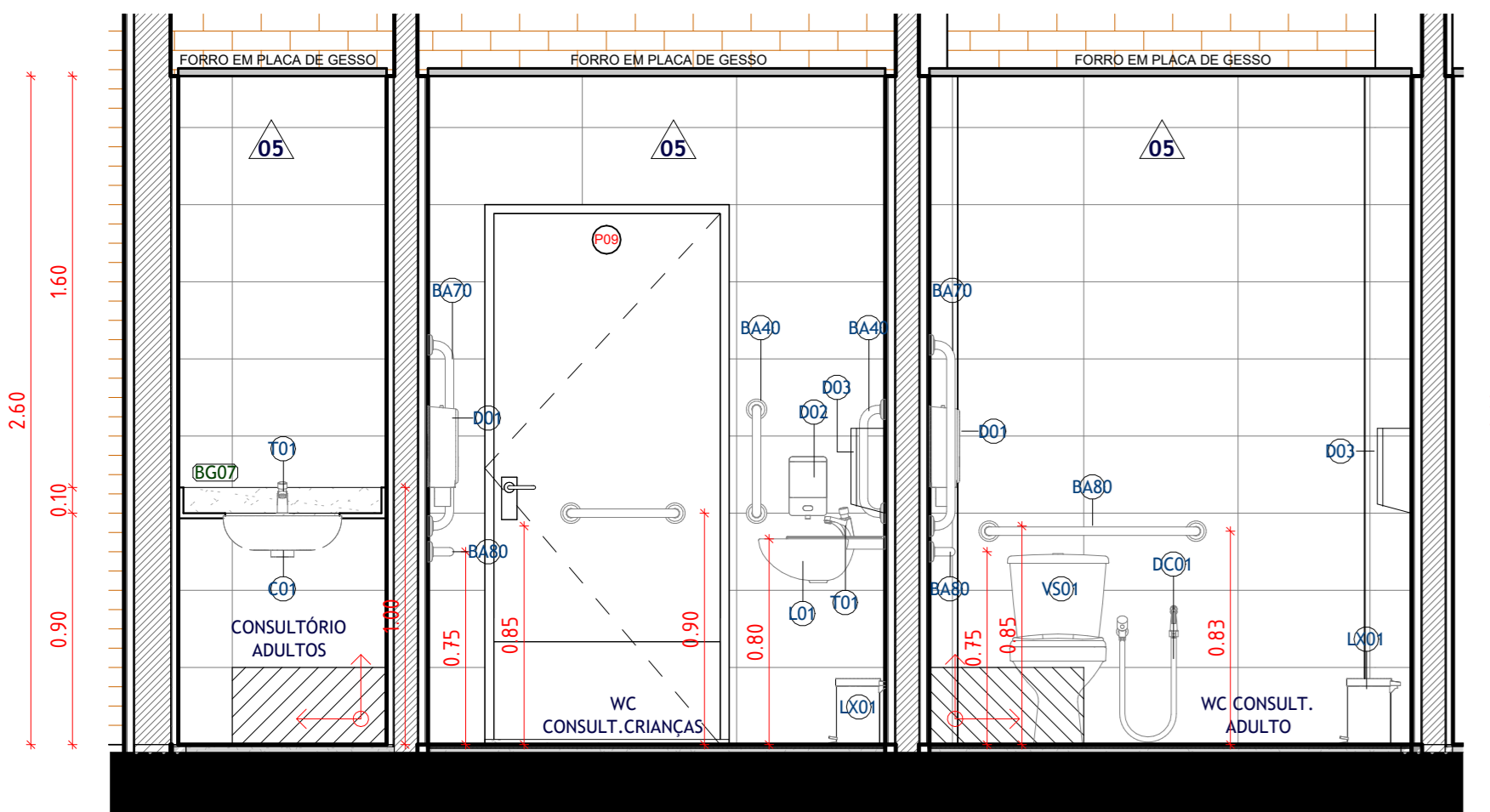
2 D01 - VISTA AA' ESCALA 1:25
