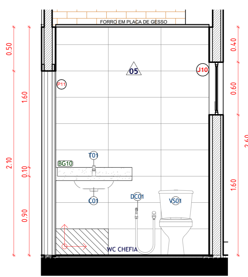
18 D03 - VISTA EE' ESCALA 1:25
