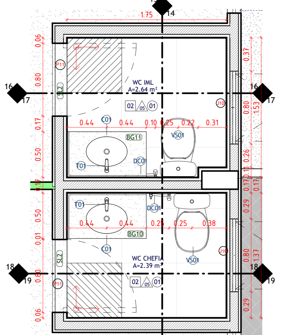
13 D03 - WC CHEFIA/ WC IML ESCALA 1:25
