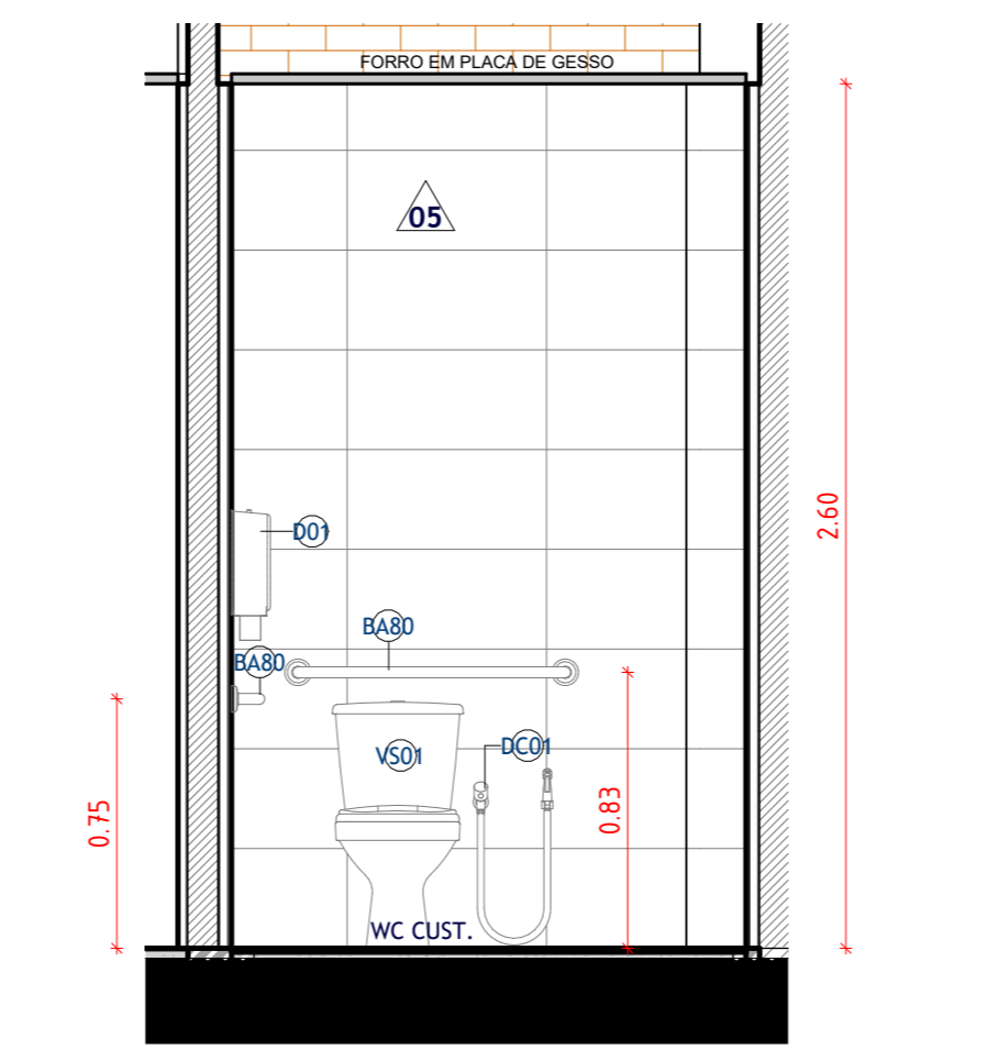
12 D02 - VISTA DD' ESCALA 1:25
