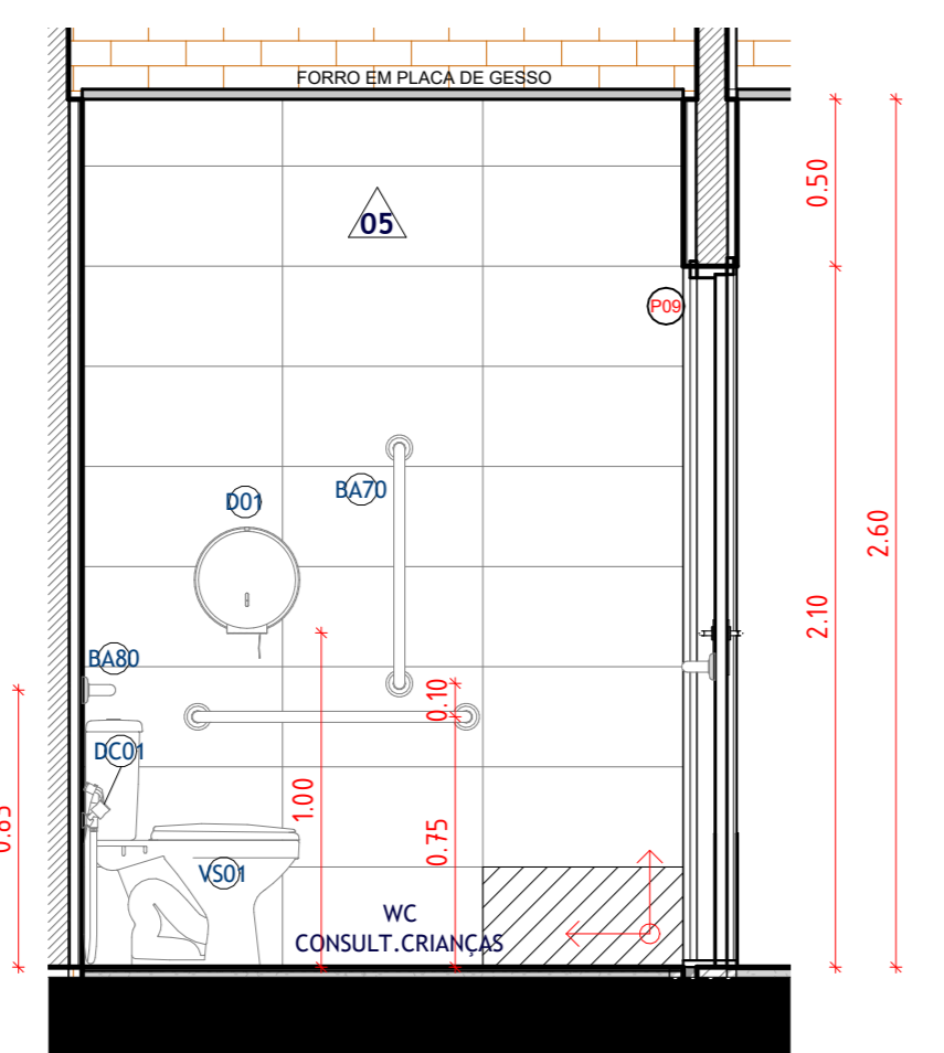
5 D01 - VISTA DD' ESCALA 1:25
