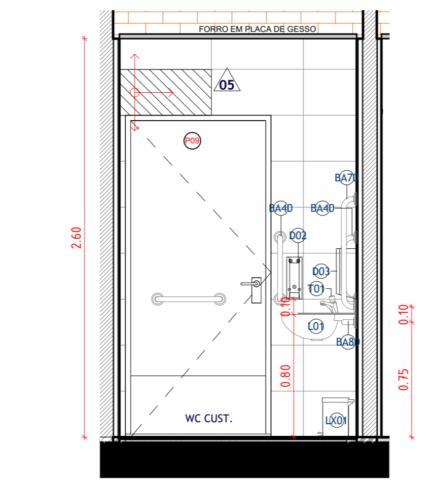
11 D02 - VISTA CC' ESCALA 1:25
