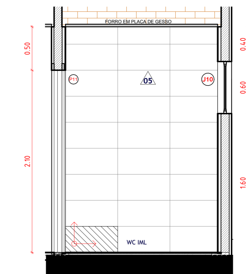
16 D03 - VISTA CC' ESCALA 1:25
