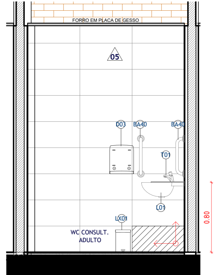
6 D01 - VISTA EE' ESCALA 1:25
