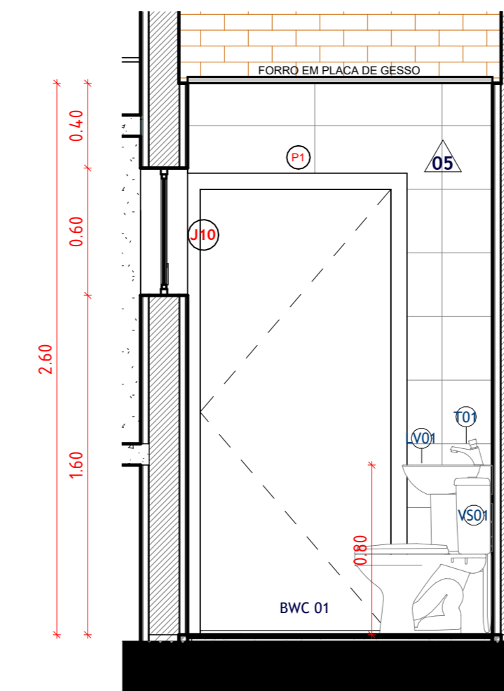
4 D05 - VISTA CC' ESCALA 1:25
