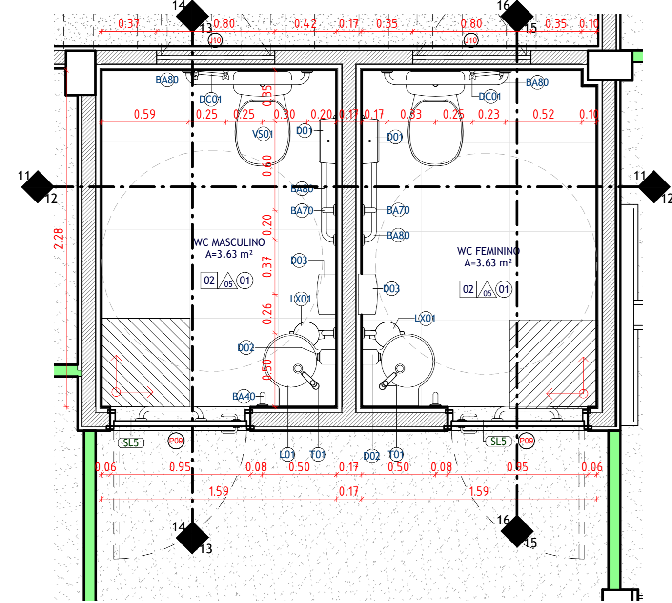
10 D06 - WC MASC/WC FEM. ESCALA 1:25
