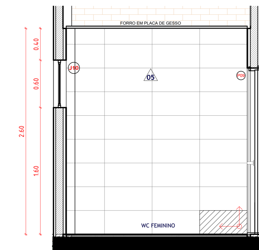
15 D06 - VISTA EE' ESCALA 1:25
