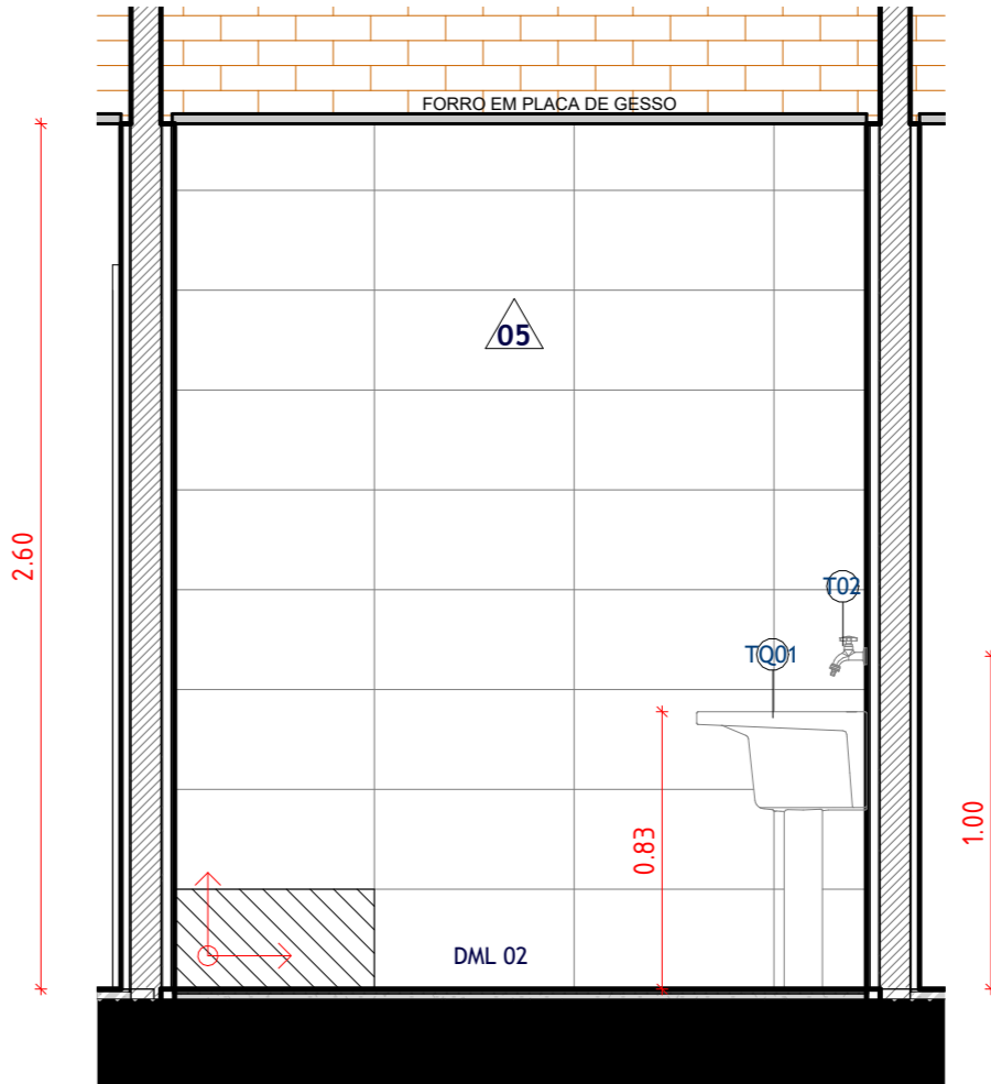
9 D05 - VISTA HH' ESCALA 1:25
