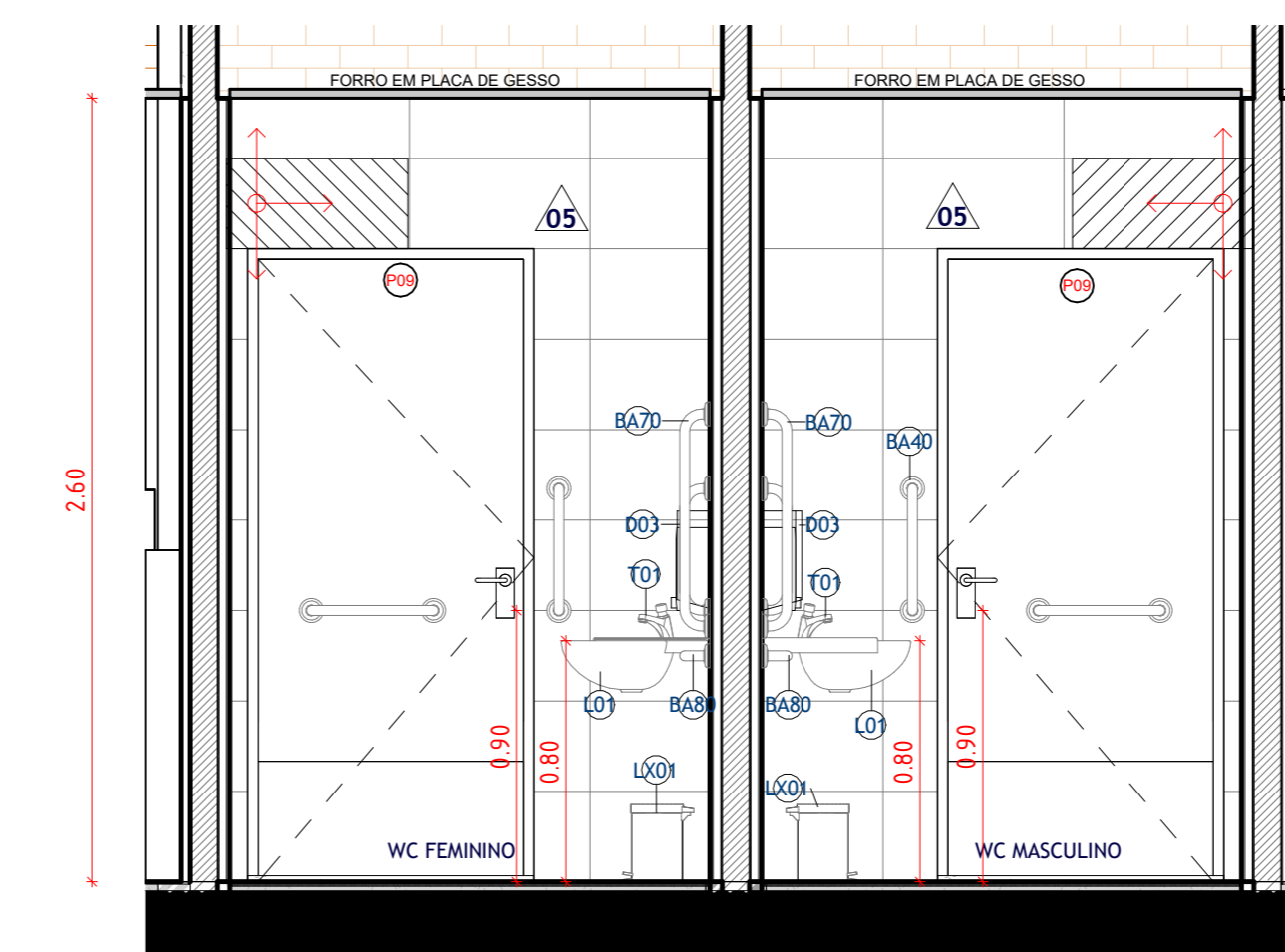
12 D06 - VISTA BB' ESCALA 1:25
