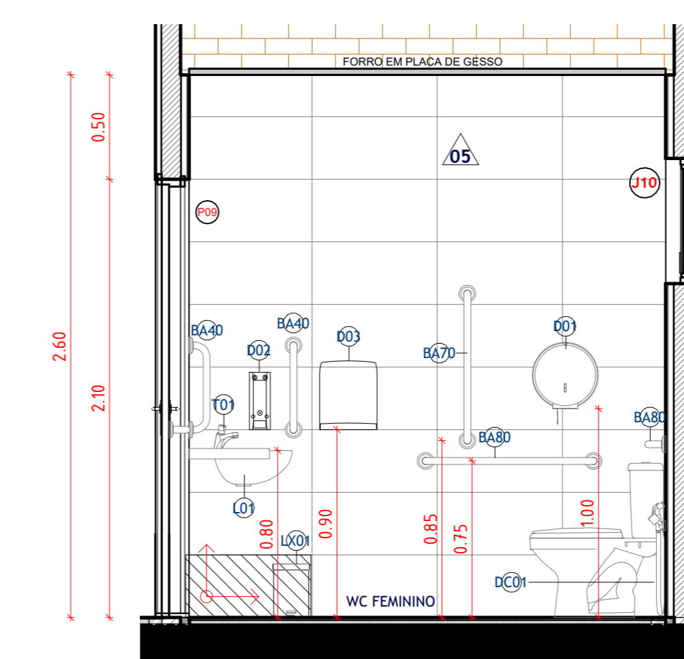
16 D06 - VISTA FF' ESCALA 1:25
