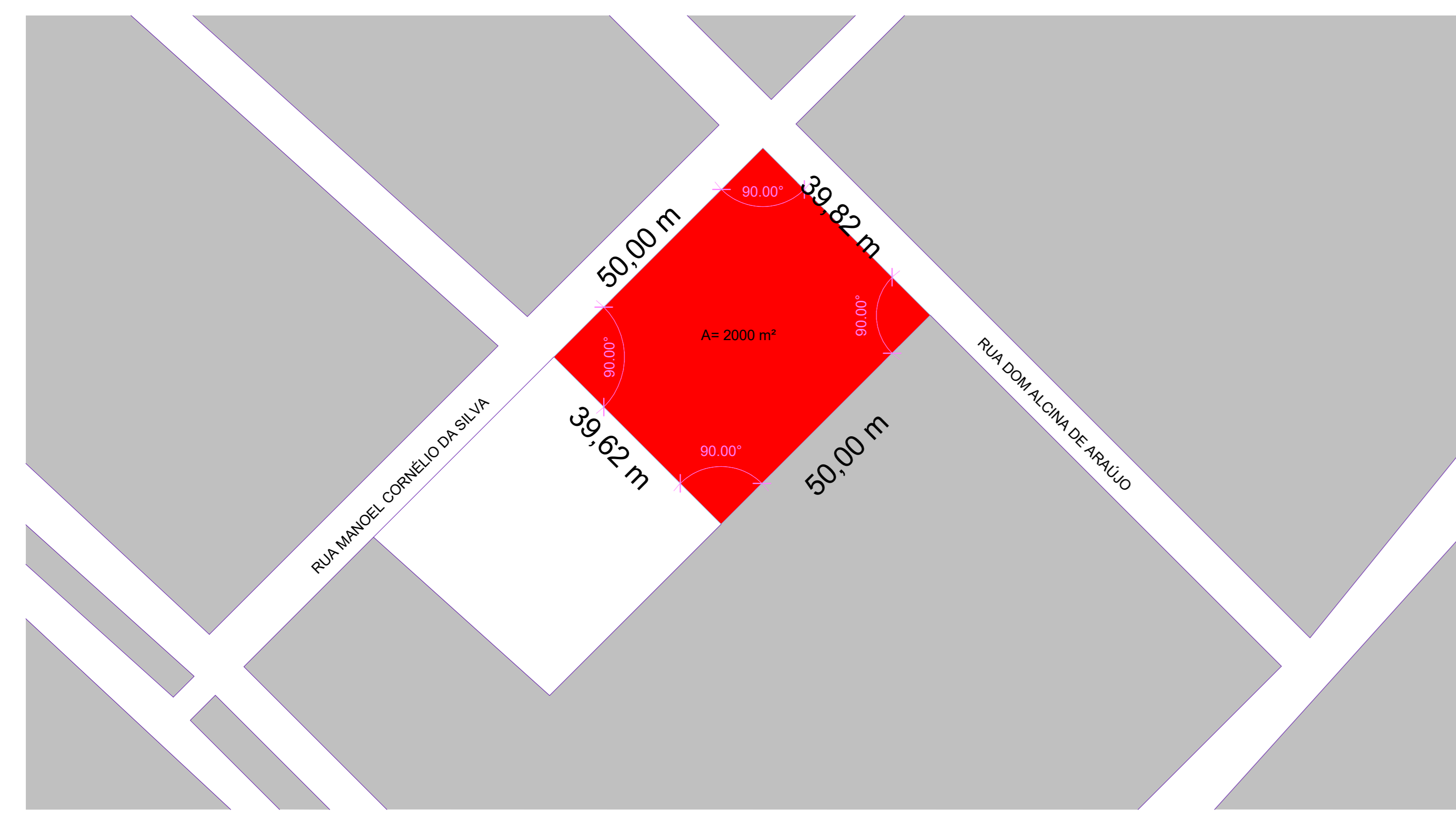
SITUAÇÃO 1:600
