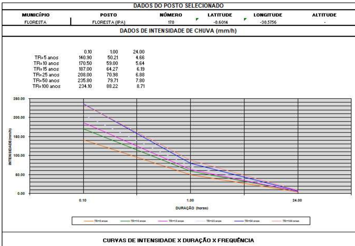
Figura EH-06: Curvas de Intensidade x Duração x Frequência
