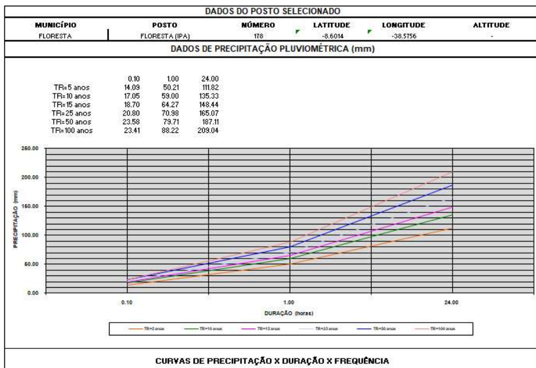
Figura EH-05: Curvas de Precipitação x Duração x Freqüência
