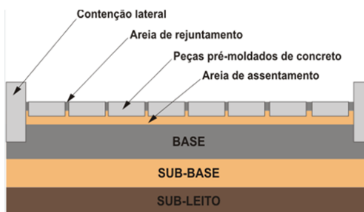
Estrutura do pavimento intertravado
