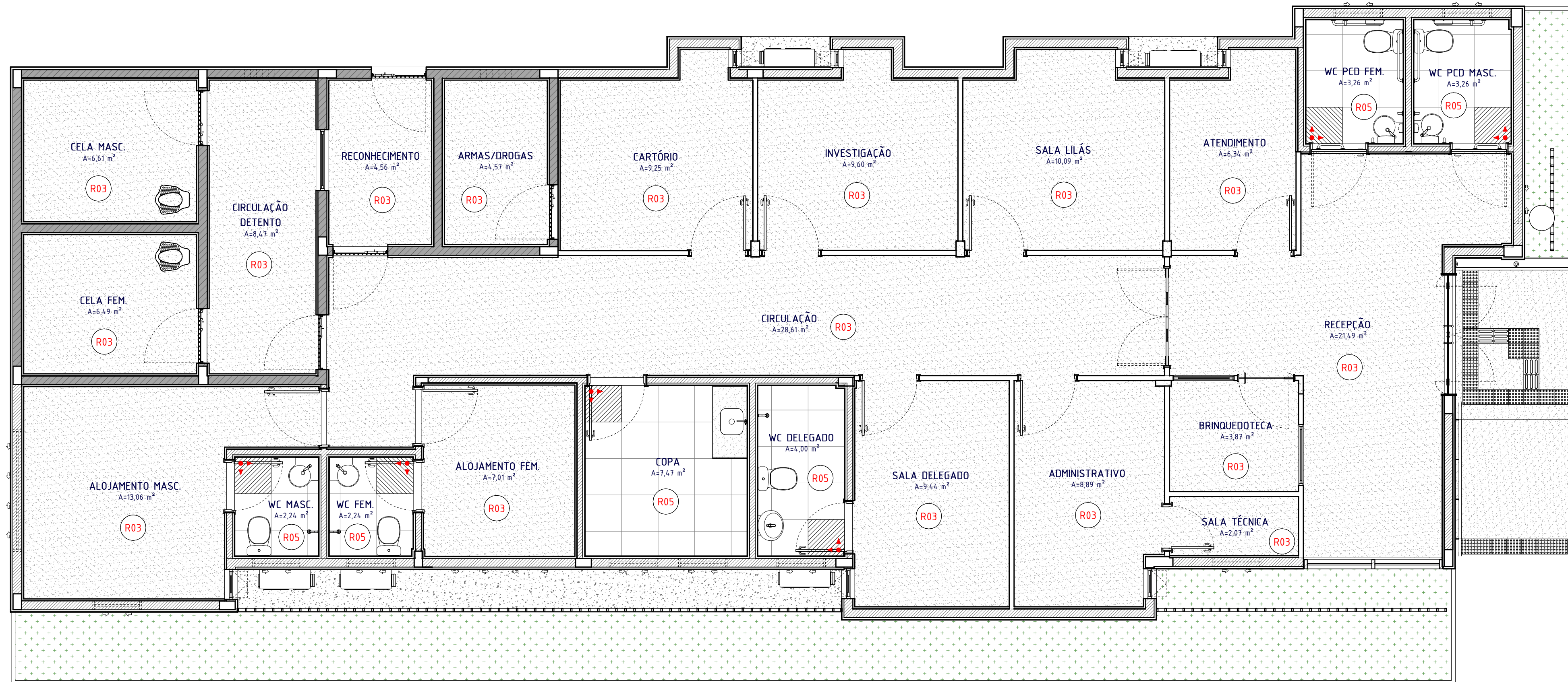
1 PAGINAÇÃO DE PISO - TÉRREO 1 : 50
