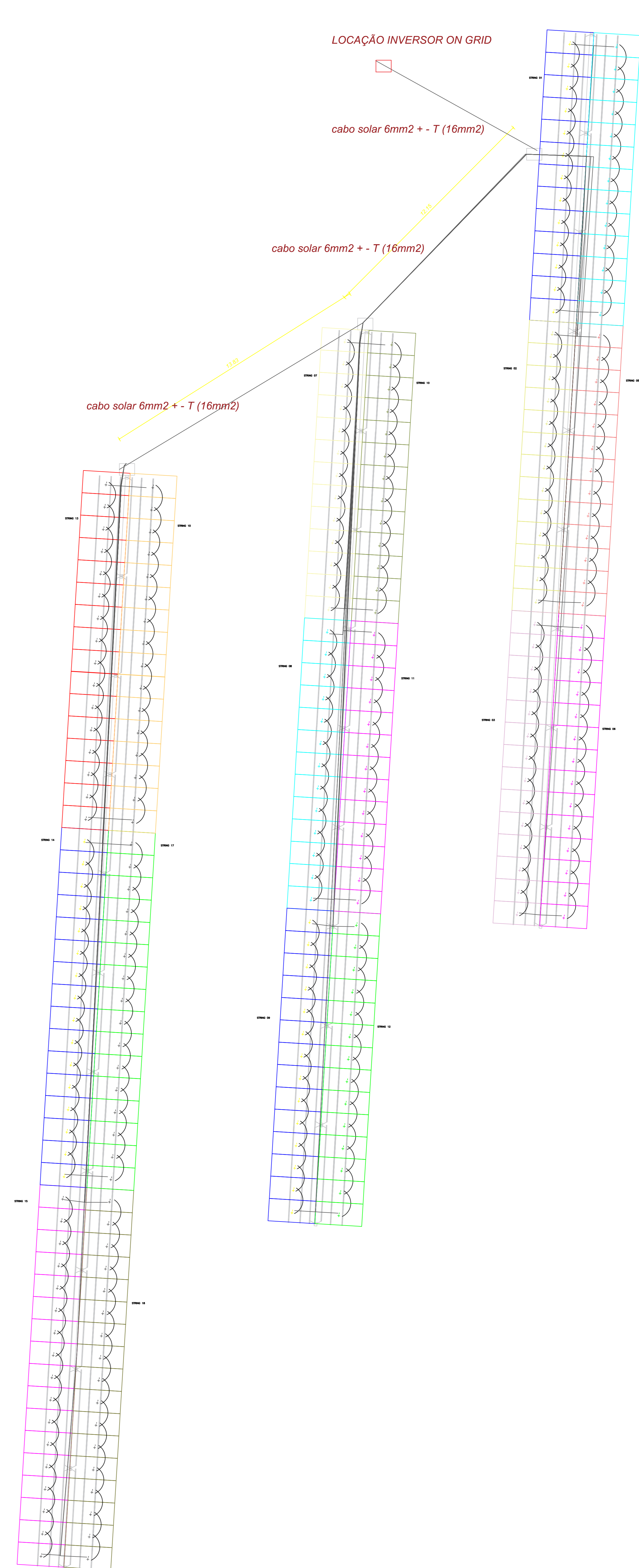
PLANTA BAIXA - DIVISÃO DAS STRINGS
