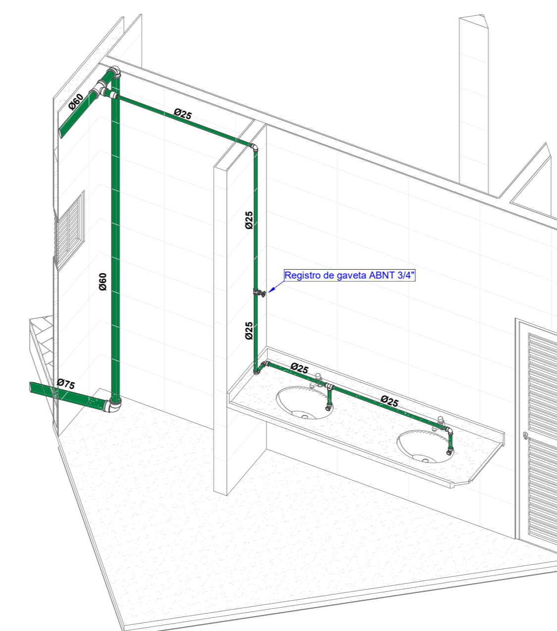
6 ISOMETRICO - VESTIÁRIO - LAVATÓRIOS ESCALA
