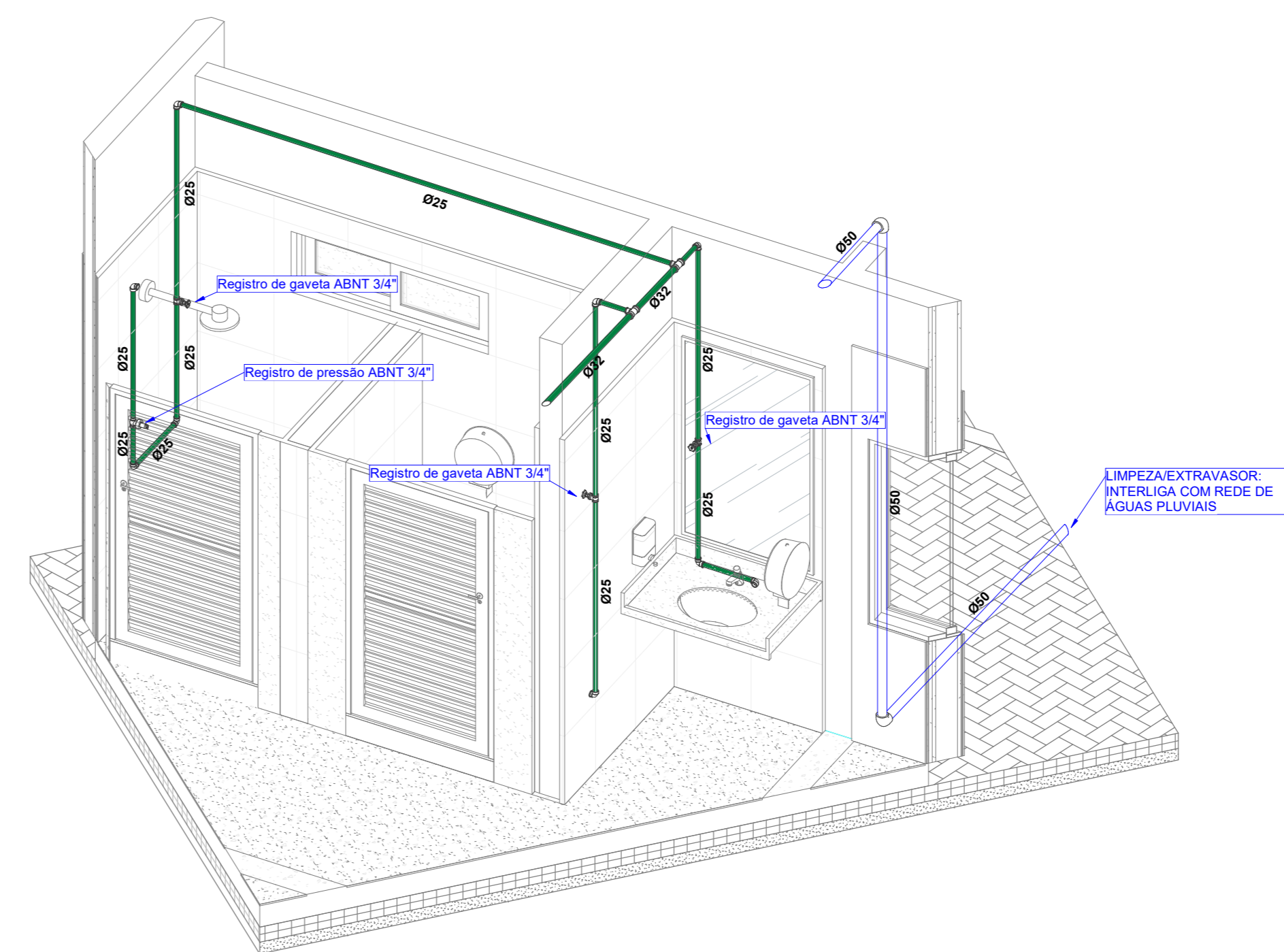
7 ISOMÉTRICO - BANHEIROS ADM ESCALA
