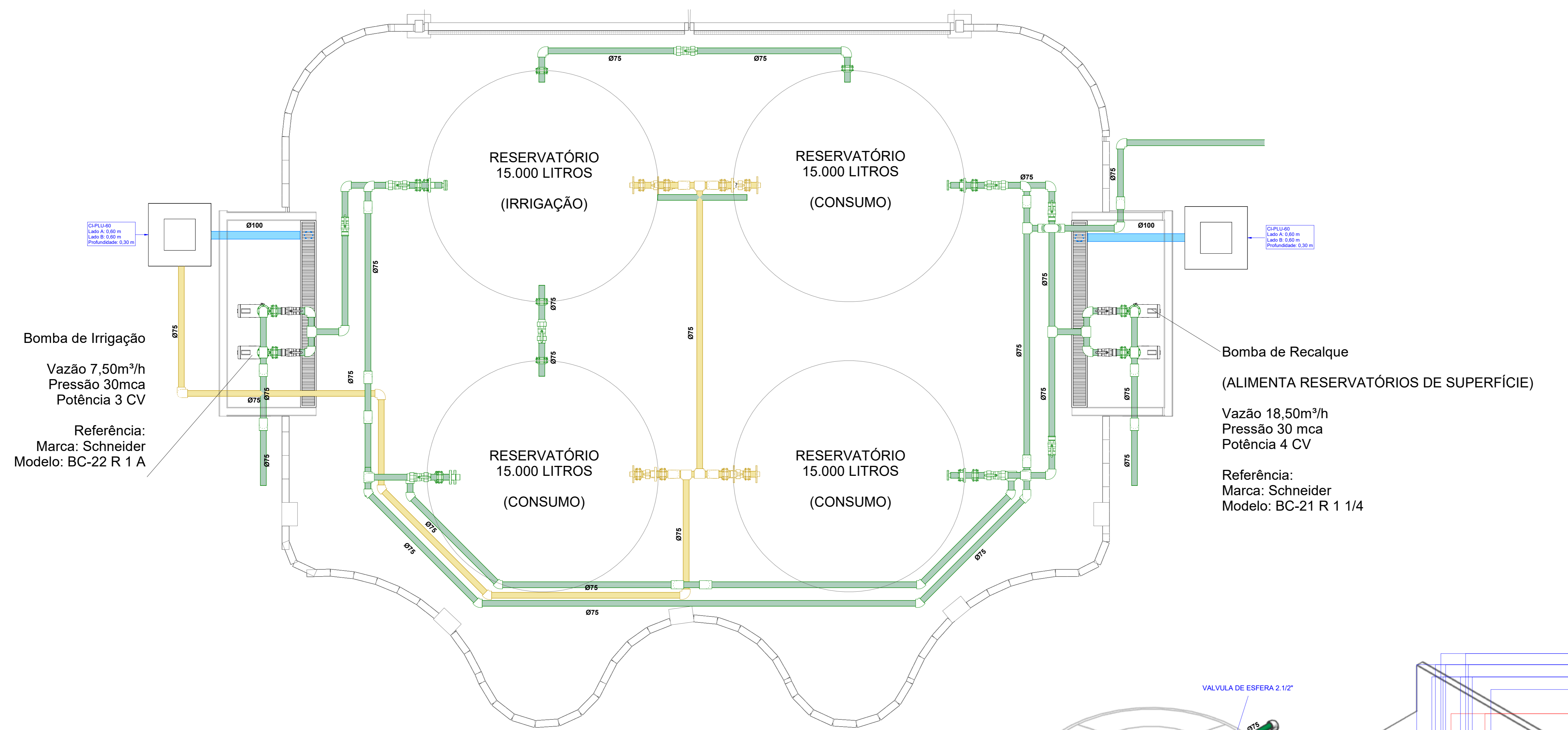
1 PLANTA BAIXA - RESERVATÓRIO DE SUPERFÍCIE (RA-01) ESCALA 1:25
