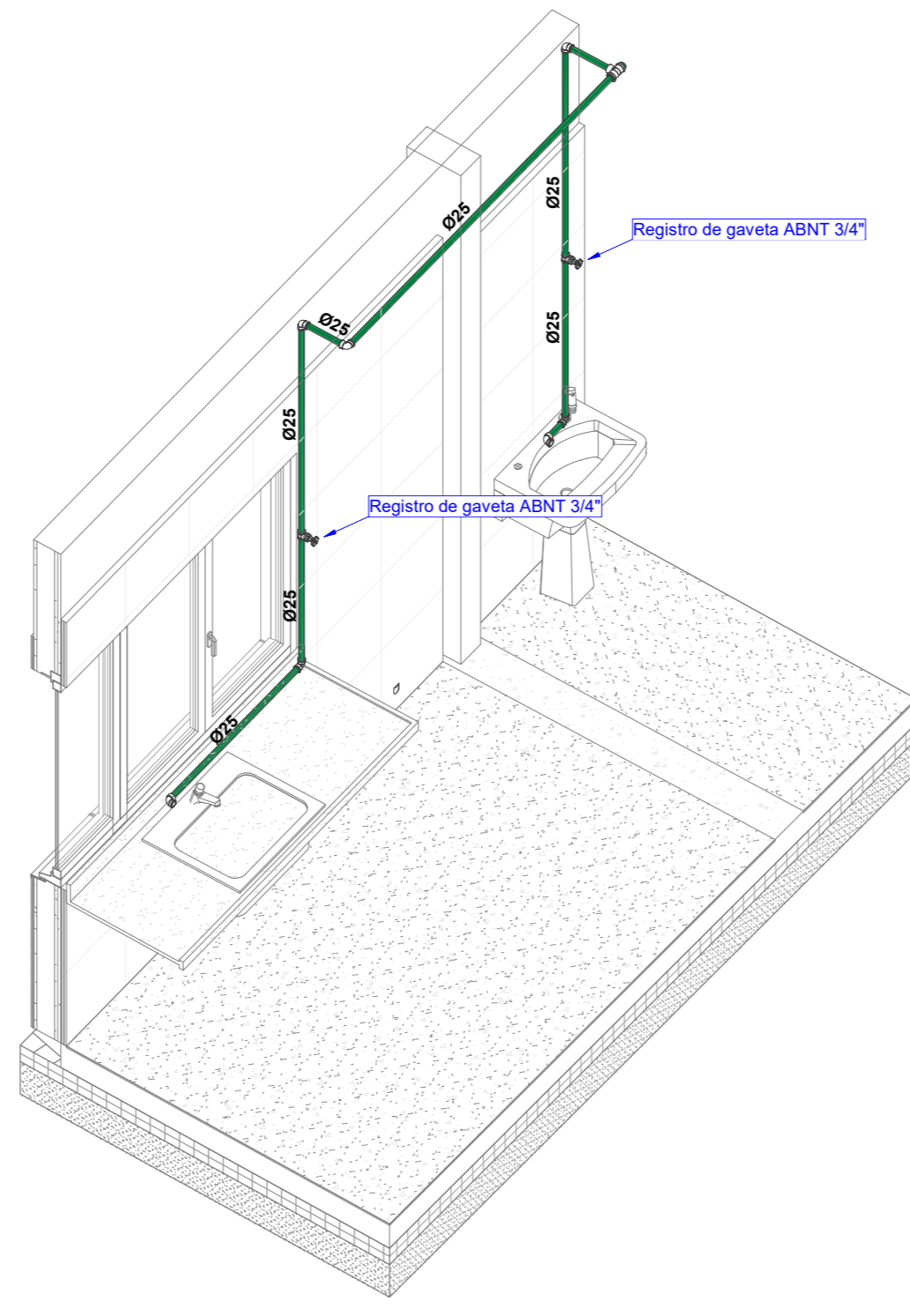
4 ISOMÉTRICO - ADM - COPA ESCALA
