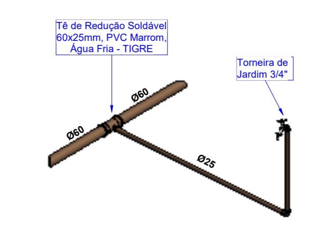
2 DETALHE LIGAÇÃO - TORNEIRA DE JARDIM ESCALA
