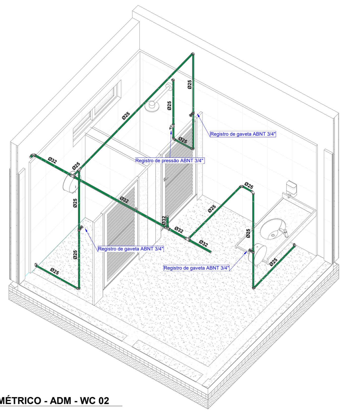
6 ISOMÉTRICO - ADM - WC 02 ESCALA
