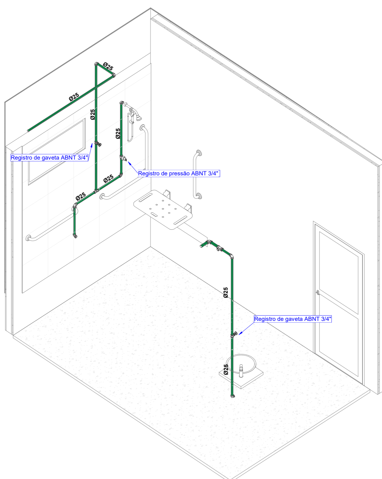
7 ISOMETRICO - SALA GUARDAS - WC 02 ESCALA
