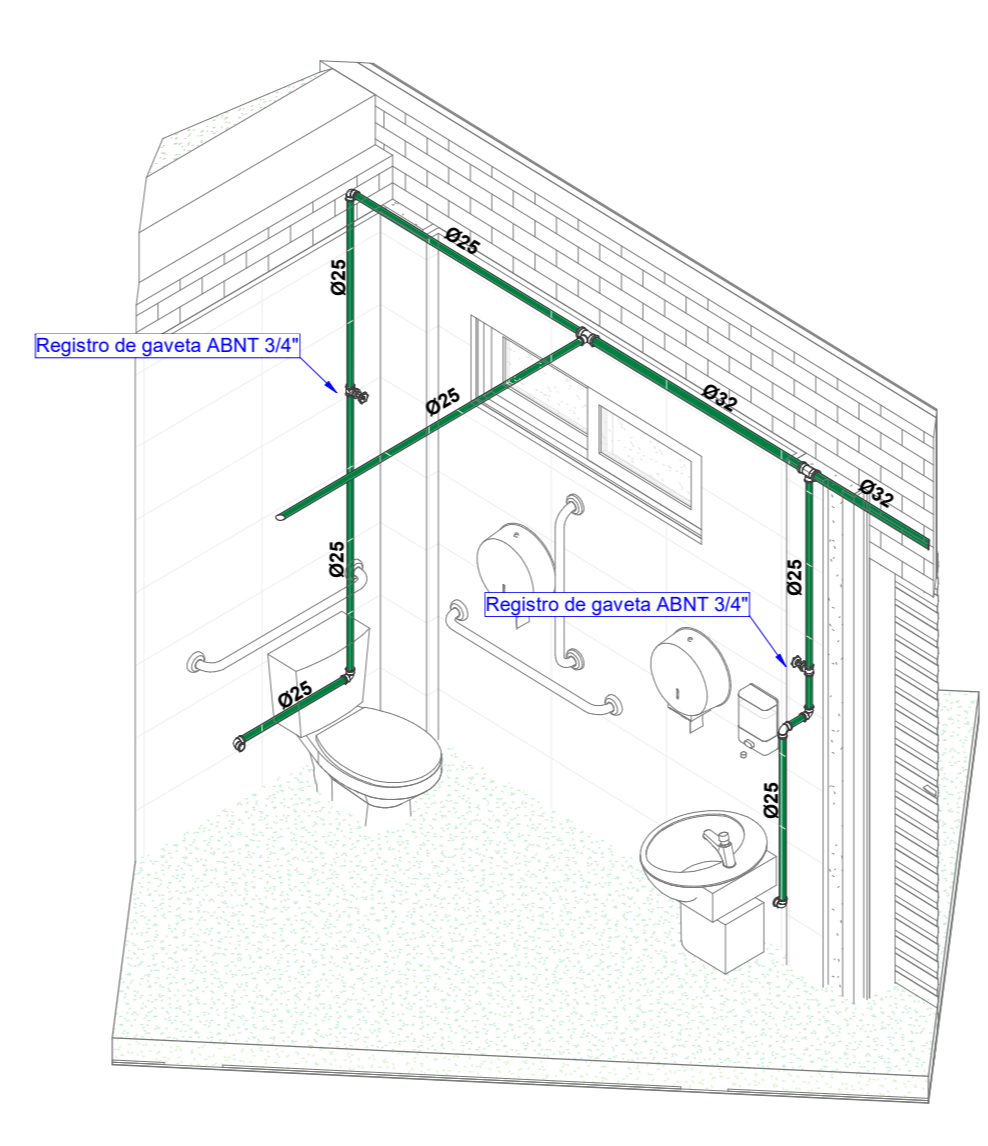
2 ISOMETRICO - BWC PCD - WC EXTERNO ESCALA
