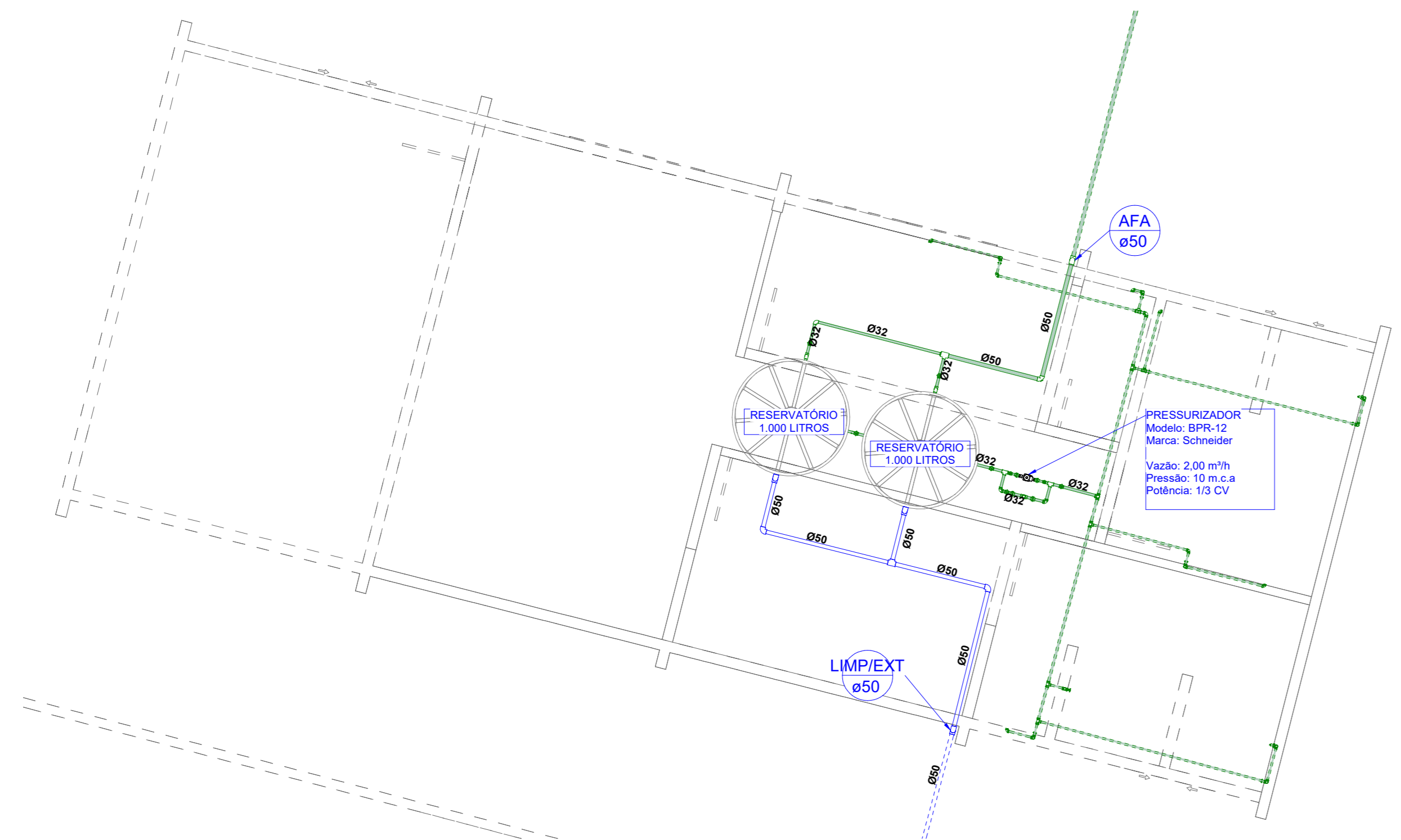
2 TÉRREO - ADM - COBERTA ESCALA 1:50
