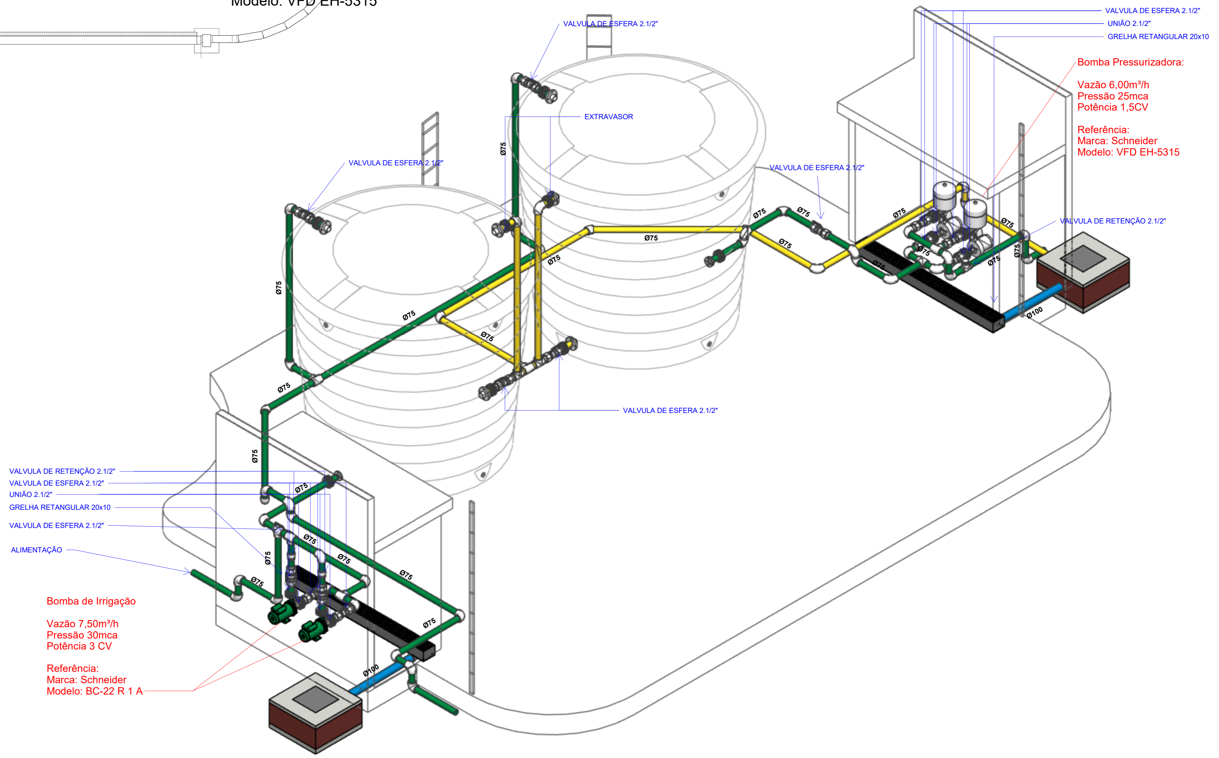
2 CASA DE BOMBAS (RA-02) ESCALA
