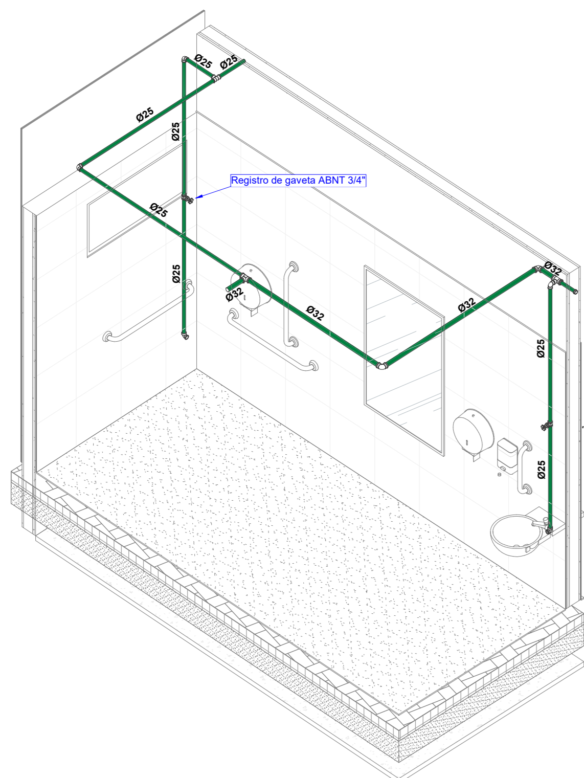
6 ISOMETRICO - SALA GUARDAS - WC 01 ESCALA
