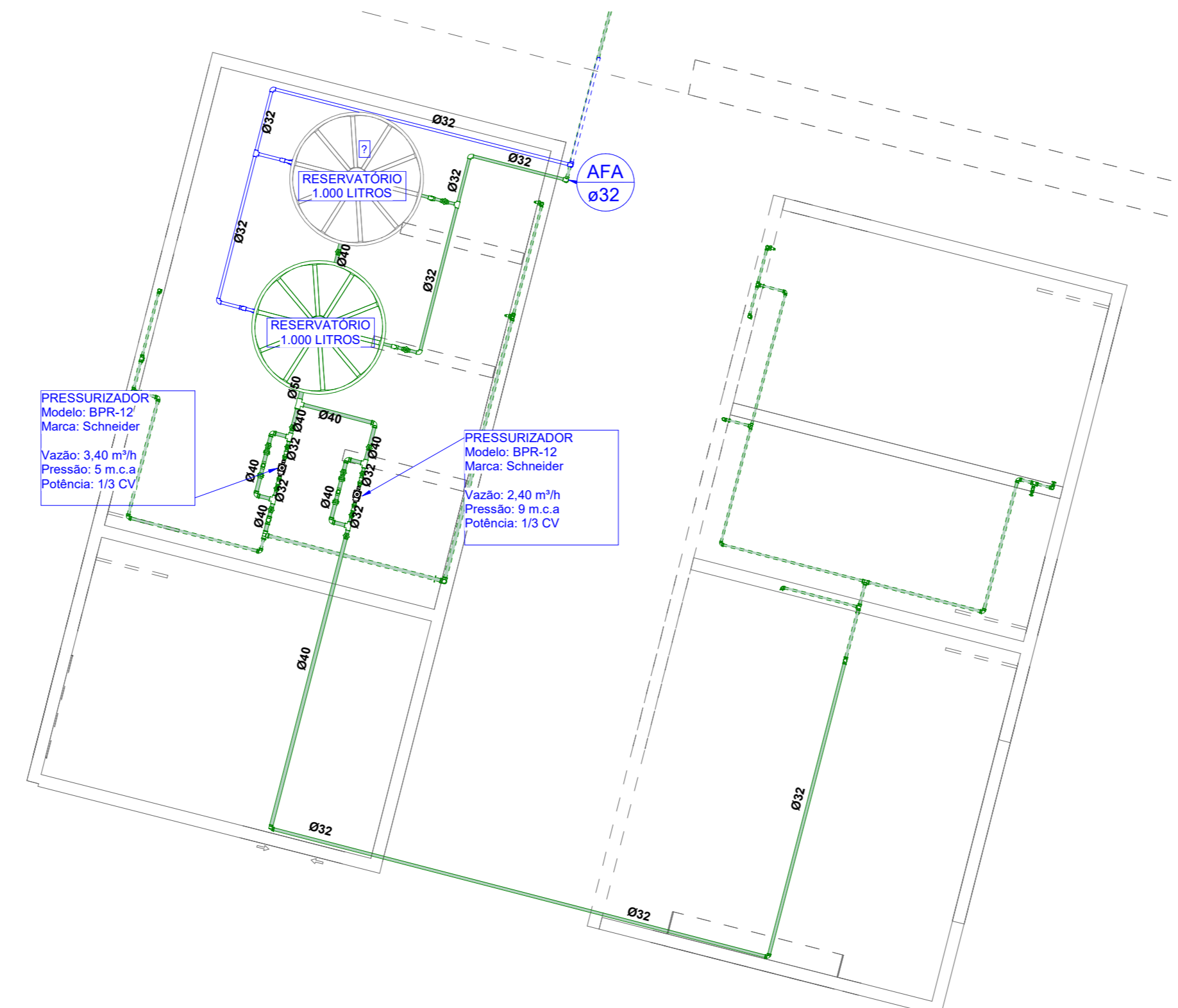
2 TÉRREO - SALA GUARDAS - COBERTA ESCALA 1:30
