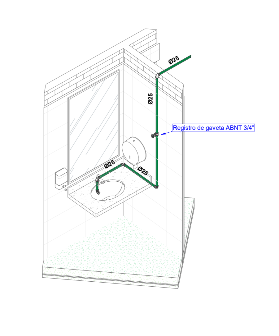
4 ISOMETRICO - LAVATÓRIO - WC EXTERNO ESCALA
