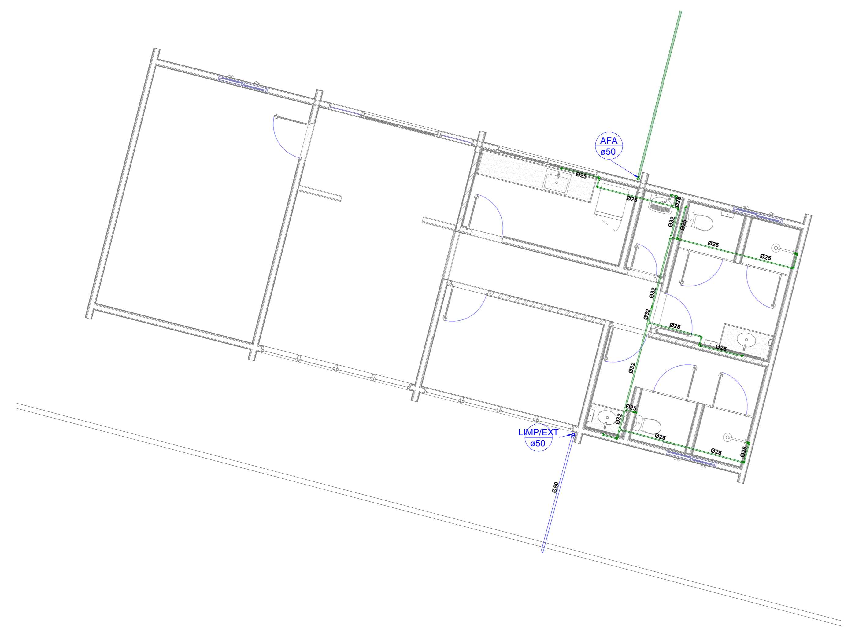
1 TÉRREO - ADM - TÉRREO ESCALA 1:50
