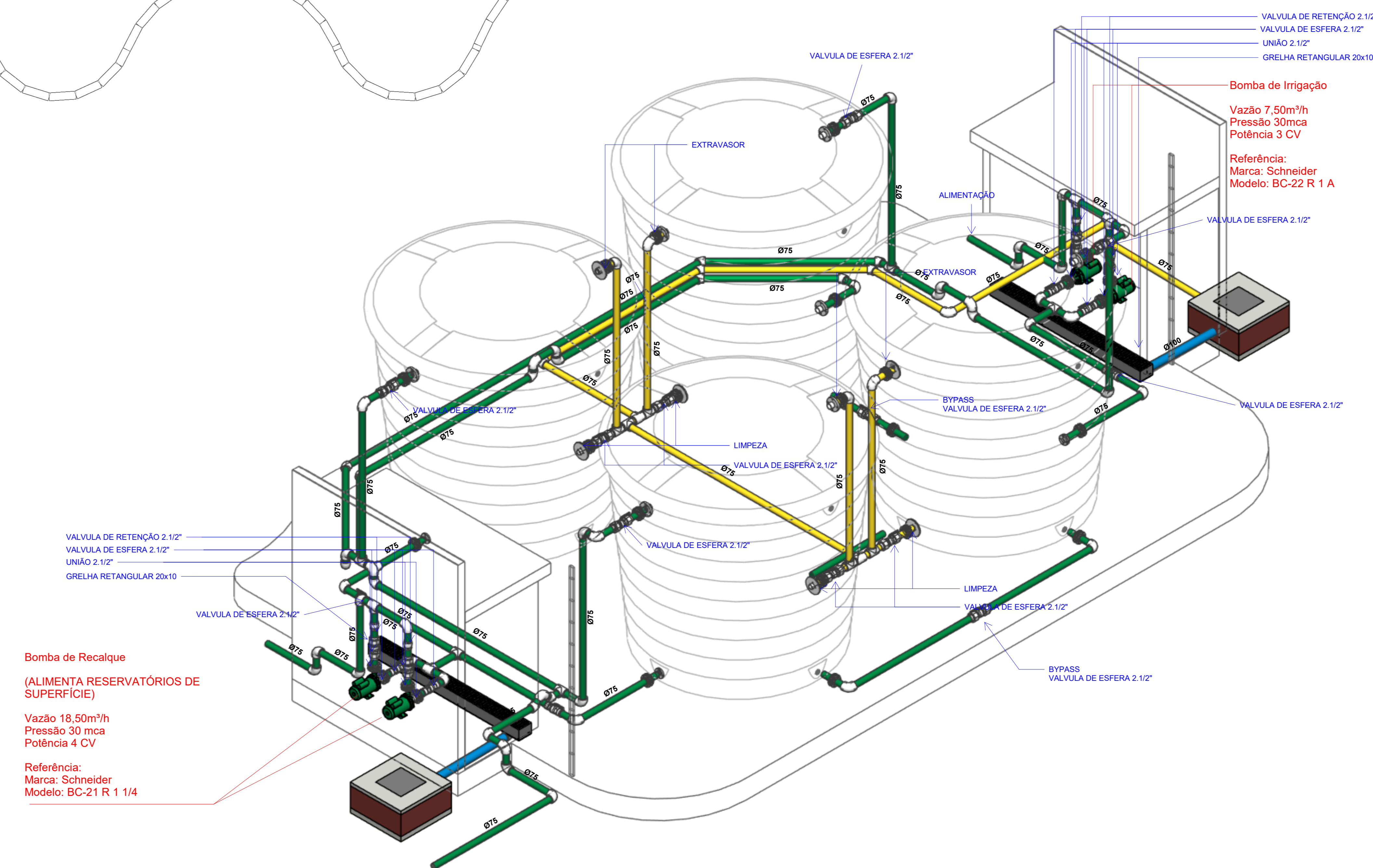
2 CASA DE BOMBAS (RA-01) ESCALA
