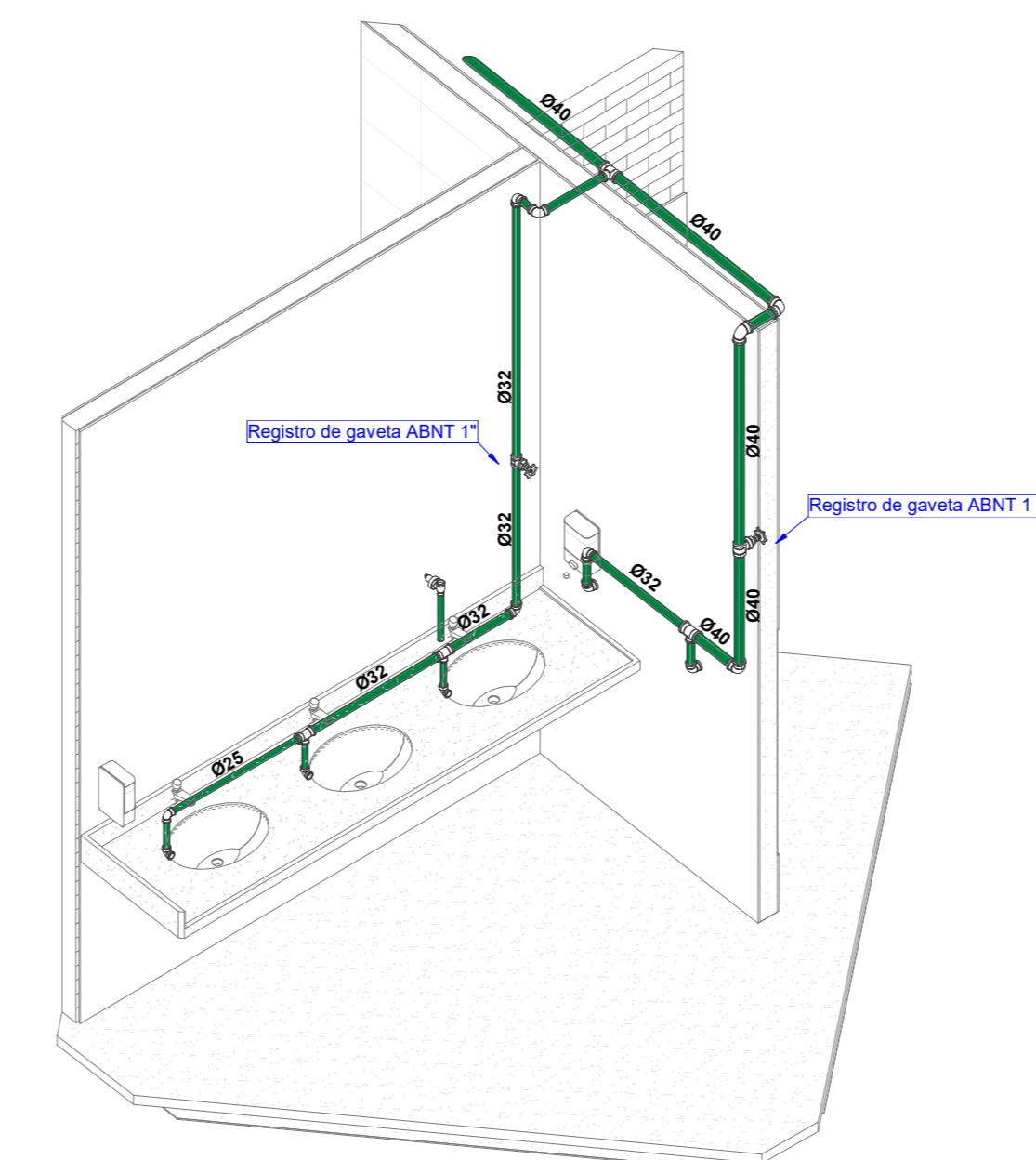
5 ISOMETRICO - VESTIÁRIO - LAVATÓRIOS E MICTÓRIOS ESCALA
