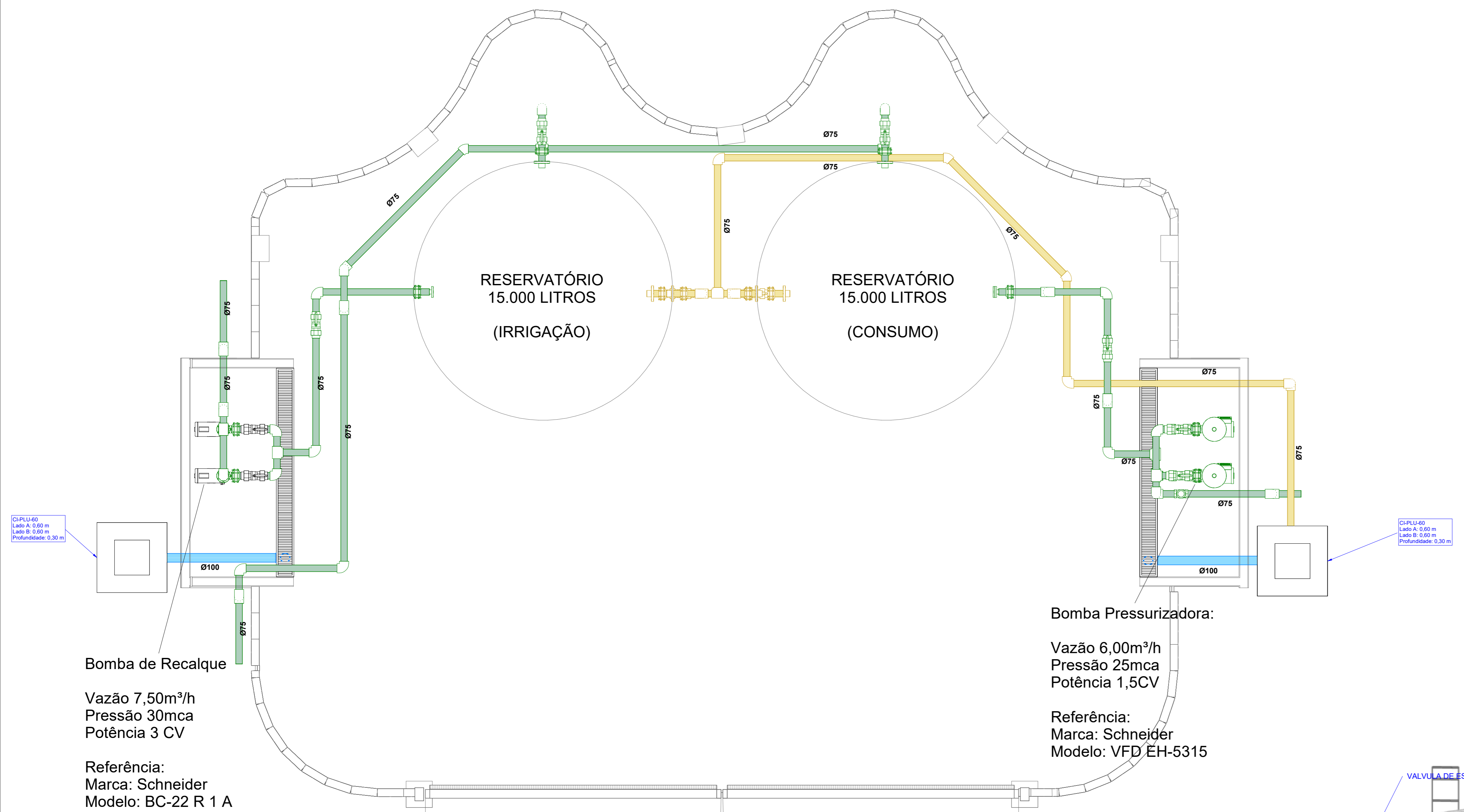
1 PLANTA BAIXA - RESERVATÓRIO DE SUPERFÍCIE (RA-02) ESCALA 1:25
