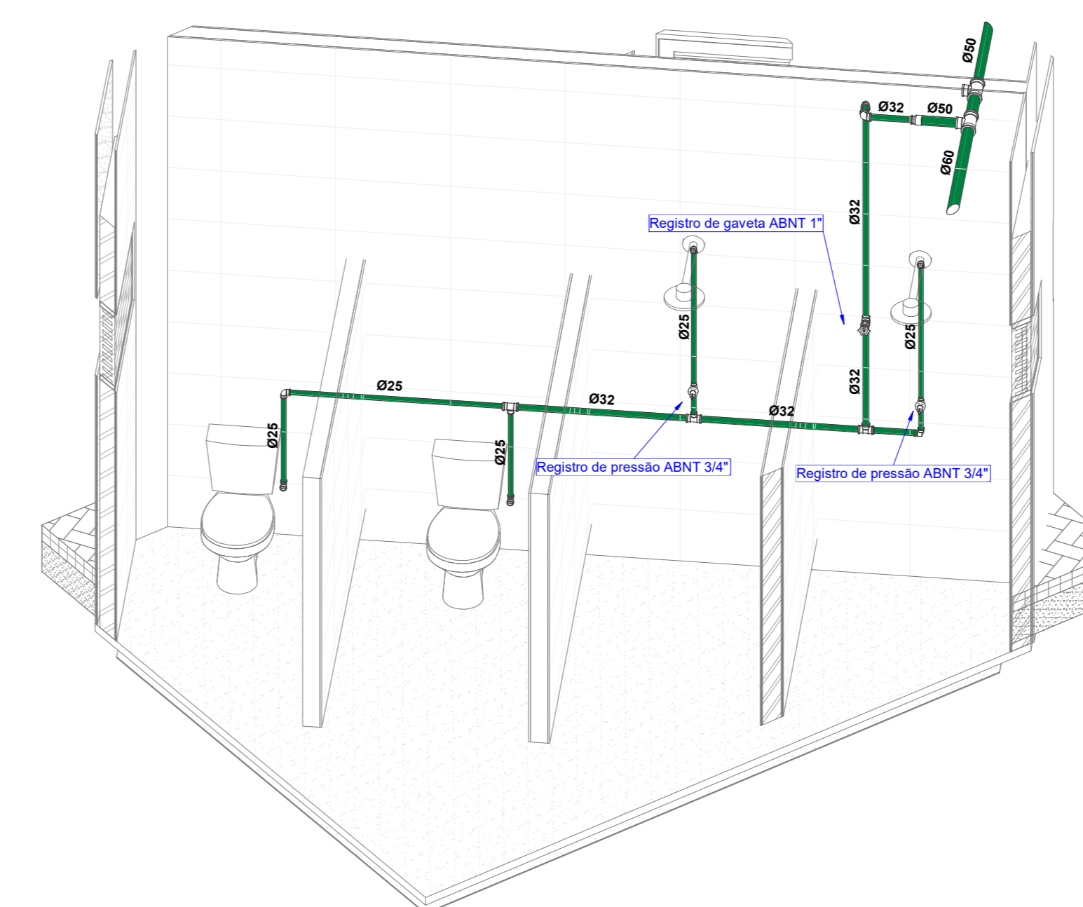
7 ISOMETRICO - WC - VESTIÁRIO ESCALA
