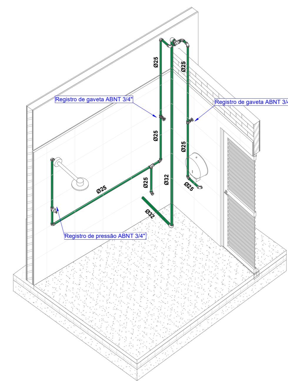
2 ISOMETRICO - WC - GUARITA ESCALA
