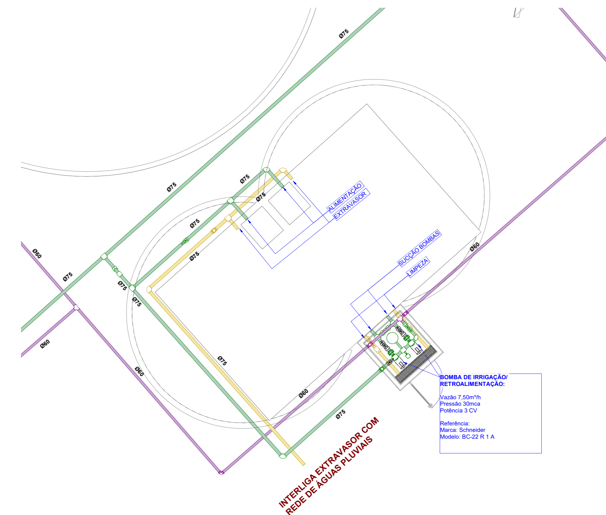
1 TÉRREO - RESERVATÓRIO VIGIAS ESCALA 1:50
