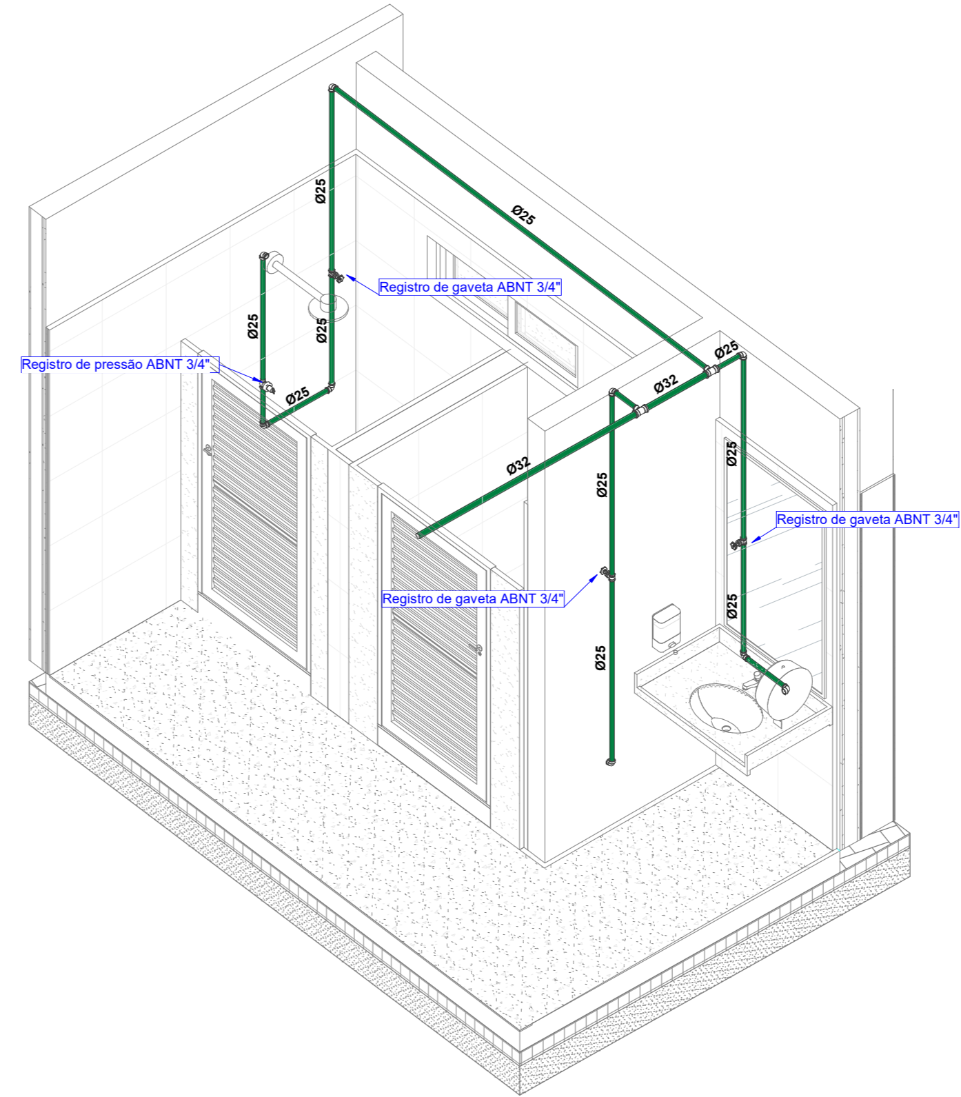
5 ISOMÉTRICO - ADM - WC 01 ESCALA
