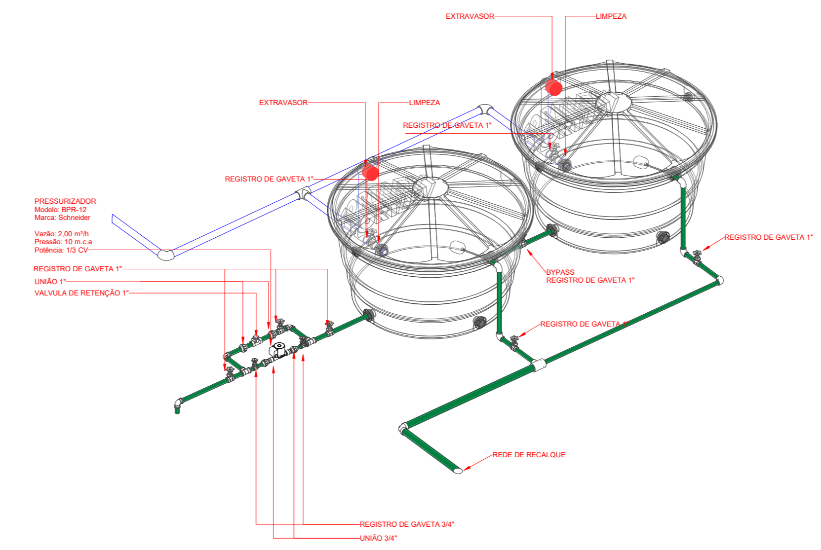
3 ISOMÉTRICO - RESERVATÓRIOS ADM - 3D ESCALA
