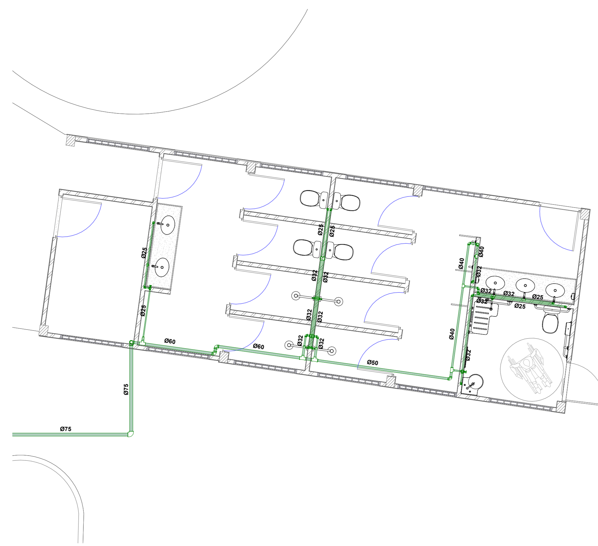
3 TÉRREO - VESTIÁRIO ESCALA 1:50
