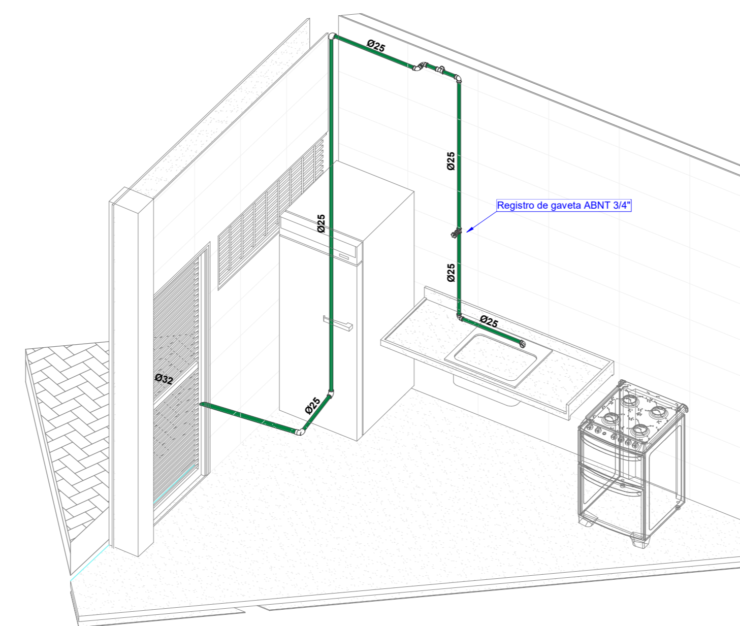
9 ISOMETRICO - QUADRAS - COPA ESCALA
