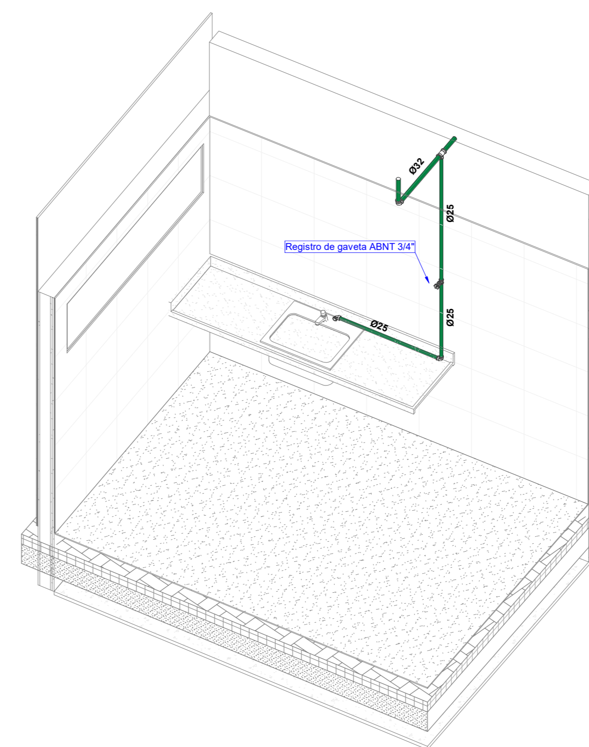
4 ISOMETRICO - SALA GUARDAS - COPA ESCALA
