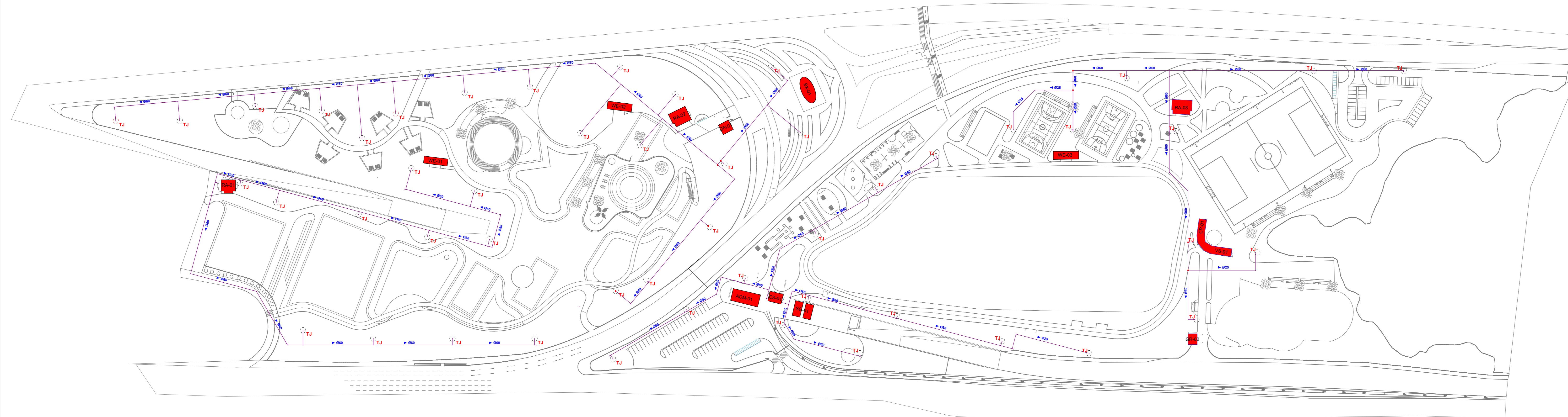
TÉRREO - REDE DE DISTRIBUIÇÃO DE IRRIGAÇÃO 1:1000
