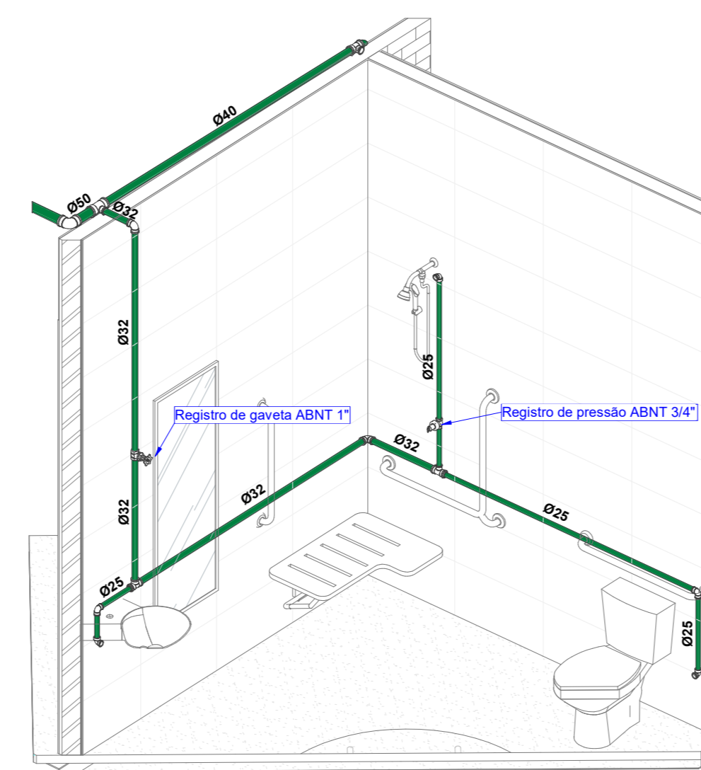
4 ISOMETRICO - VESTIÁRIO - BWC PCD ESCALA
