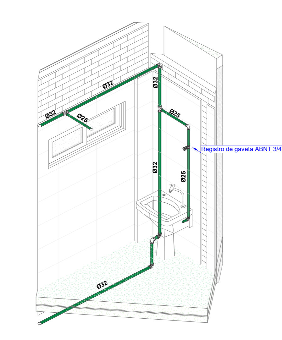
3 ISOMETRICO - DML - WC EXTERNO ESCALA
