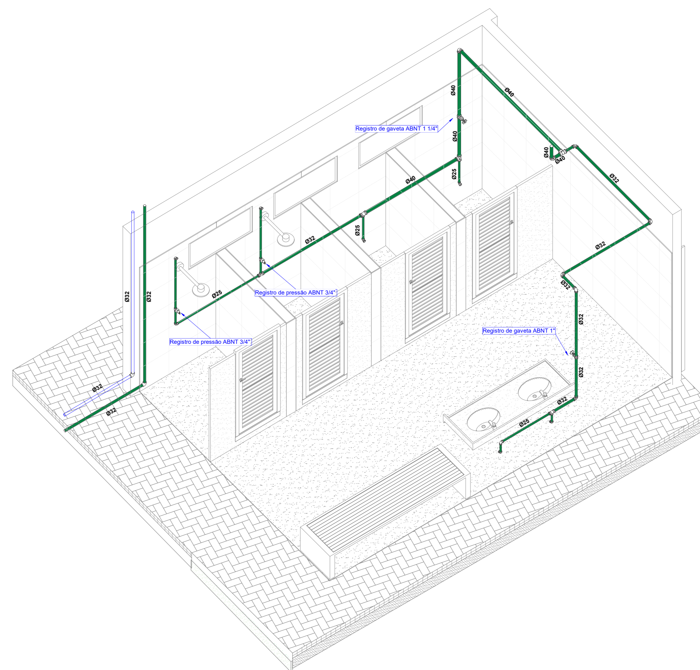
5 ISOMETRICO - SALA GUARDAS - VESTIÁRIO ESCALA
