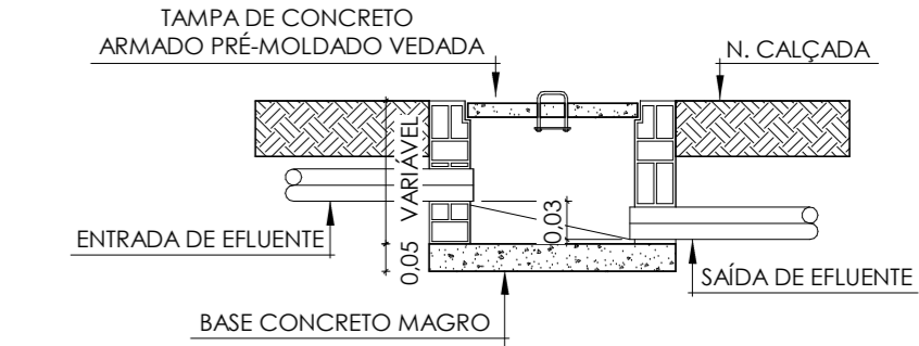
DETALHE CX. DE INSPEÇÃO E PLUVIAL (C.I./C.P.) ESCALA SEM ESCALA
