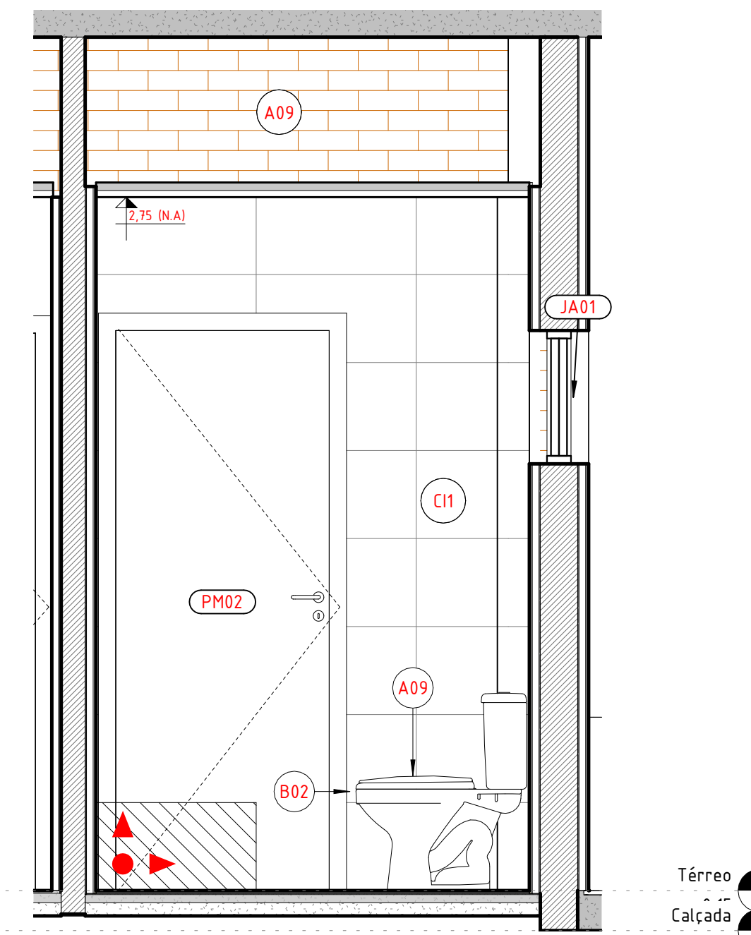
8 ELEV. ALOJ. FEM. C 1 : 20
