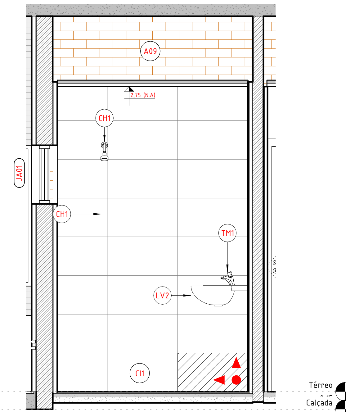
6 ELEV. ALOJ. FEM. A 1 : 20
