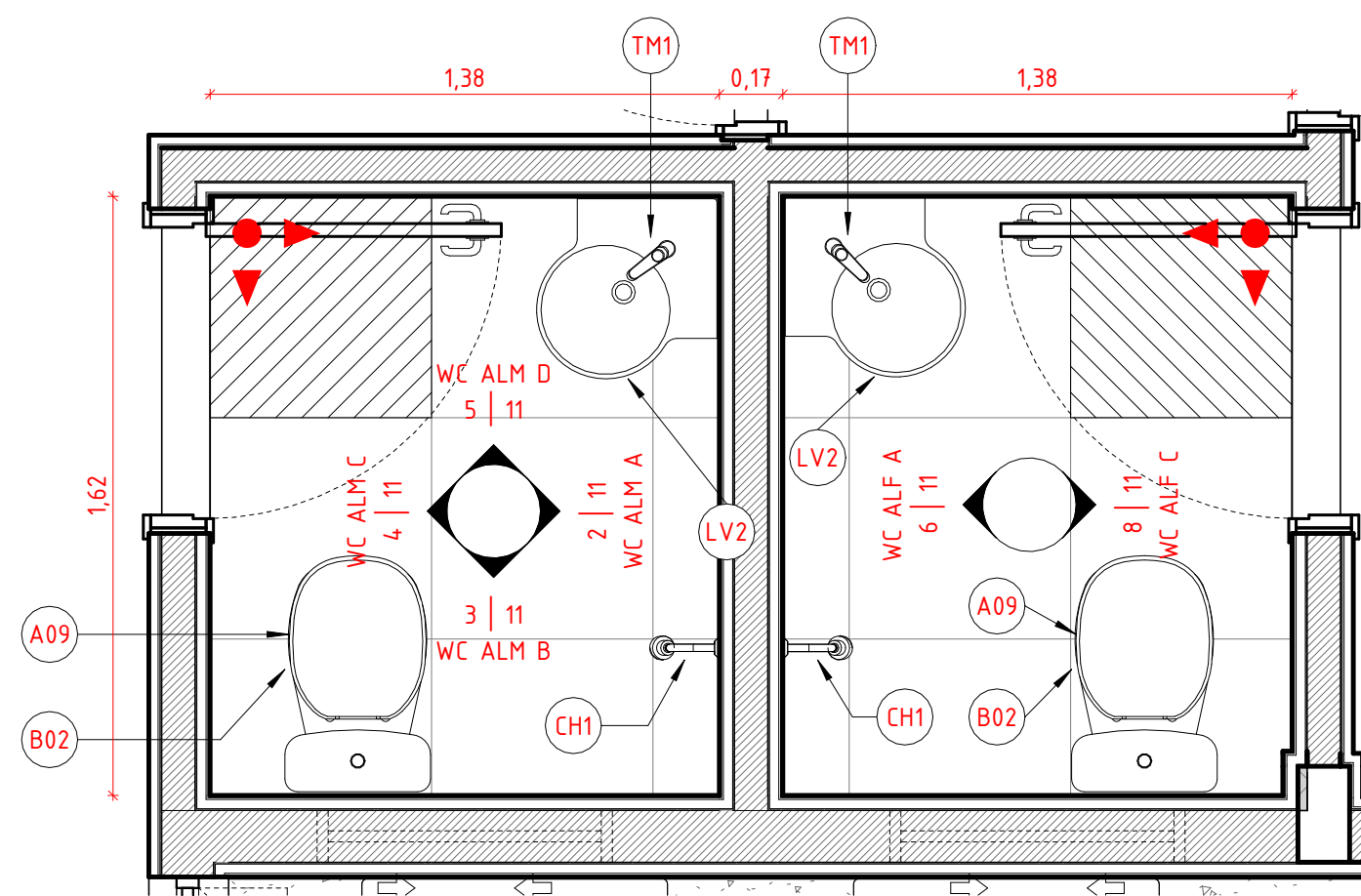
1 PLANTA BAIXA - WC ALOJAMENTO 1 : 20
