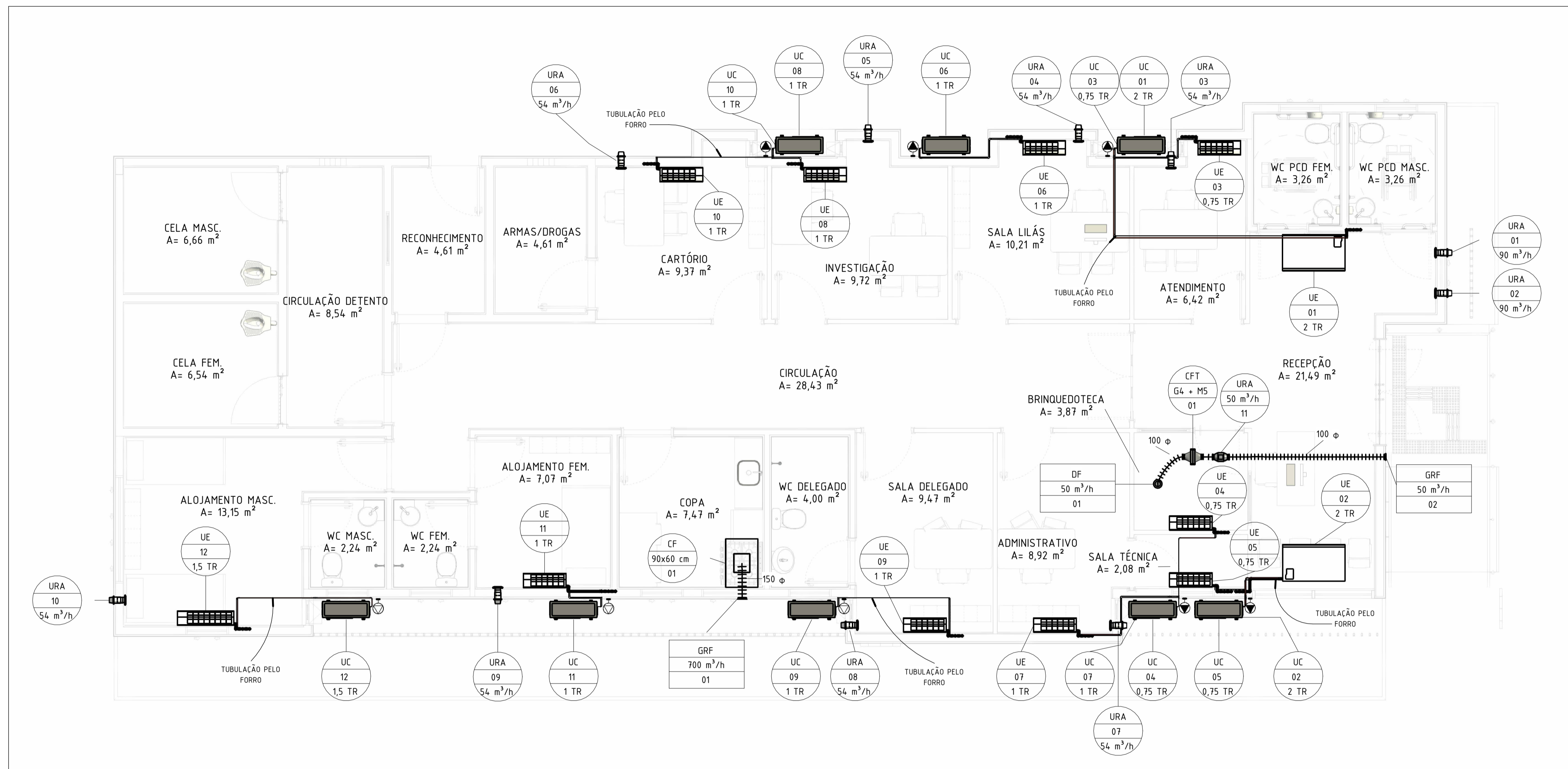
1 PLANTA BAIXA - TÉRREO 1 : 50
