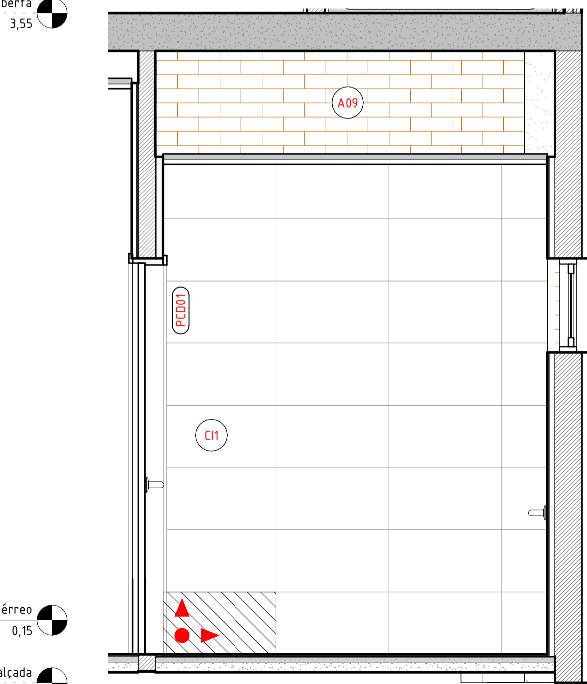
5 ELEV. WC PCD FEM. D 1 : 20
