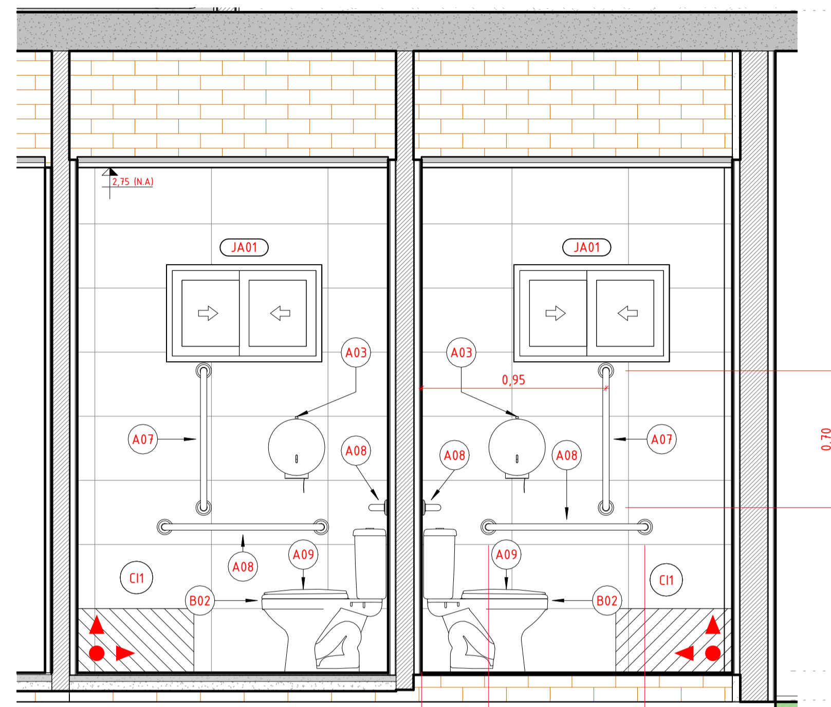
2 ELEV. WC PCD FEM. A 1 : 20
