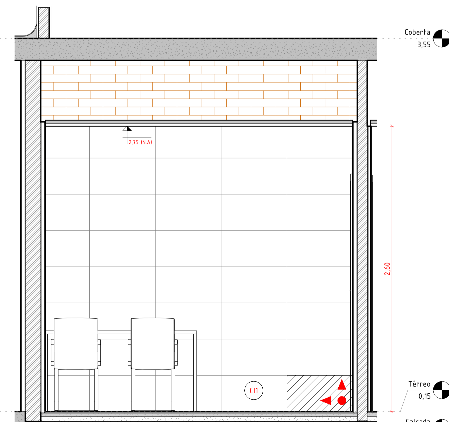
05 ELEVAÇÃO INTERNA - COPA B 1 : 20
