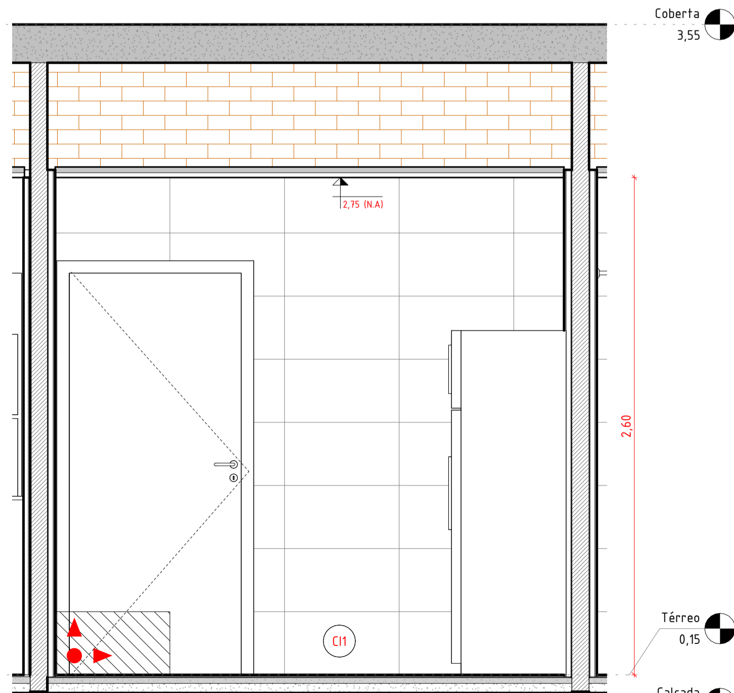
04 ELEVAÇÃO INTERNA - COPA C 1 : 20
