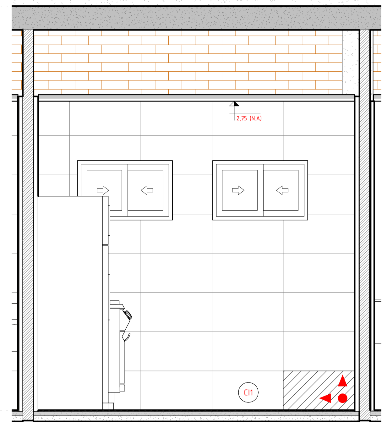
02 ELEVAÇÃO INTERNA - COPA A 1 : 20
