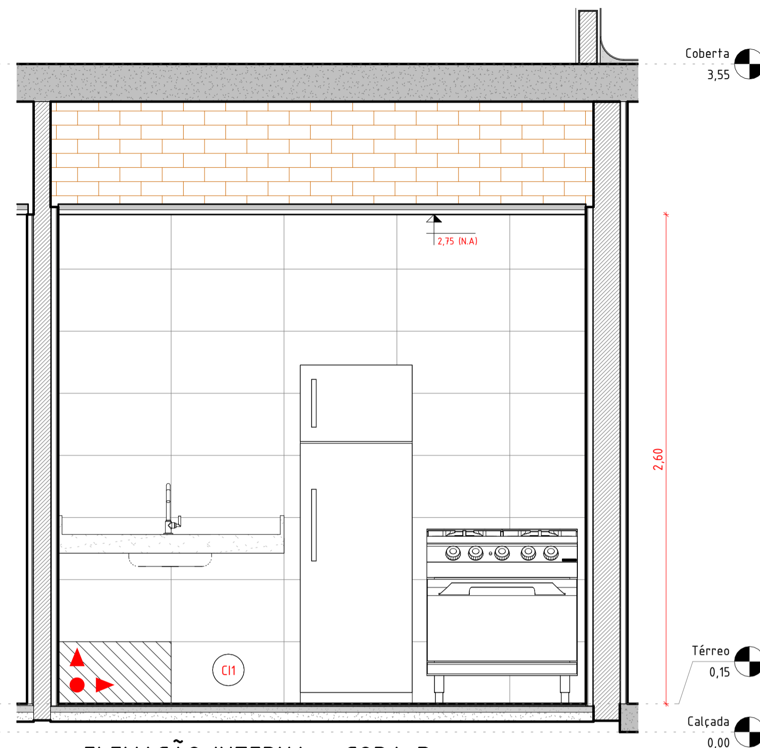
03 ELEVAÇÃO INTERNA - COPA D 1 : 20
