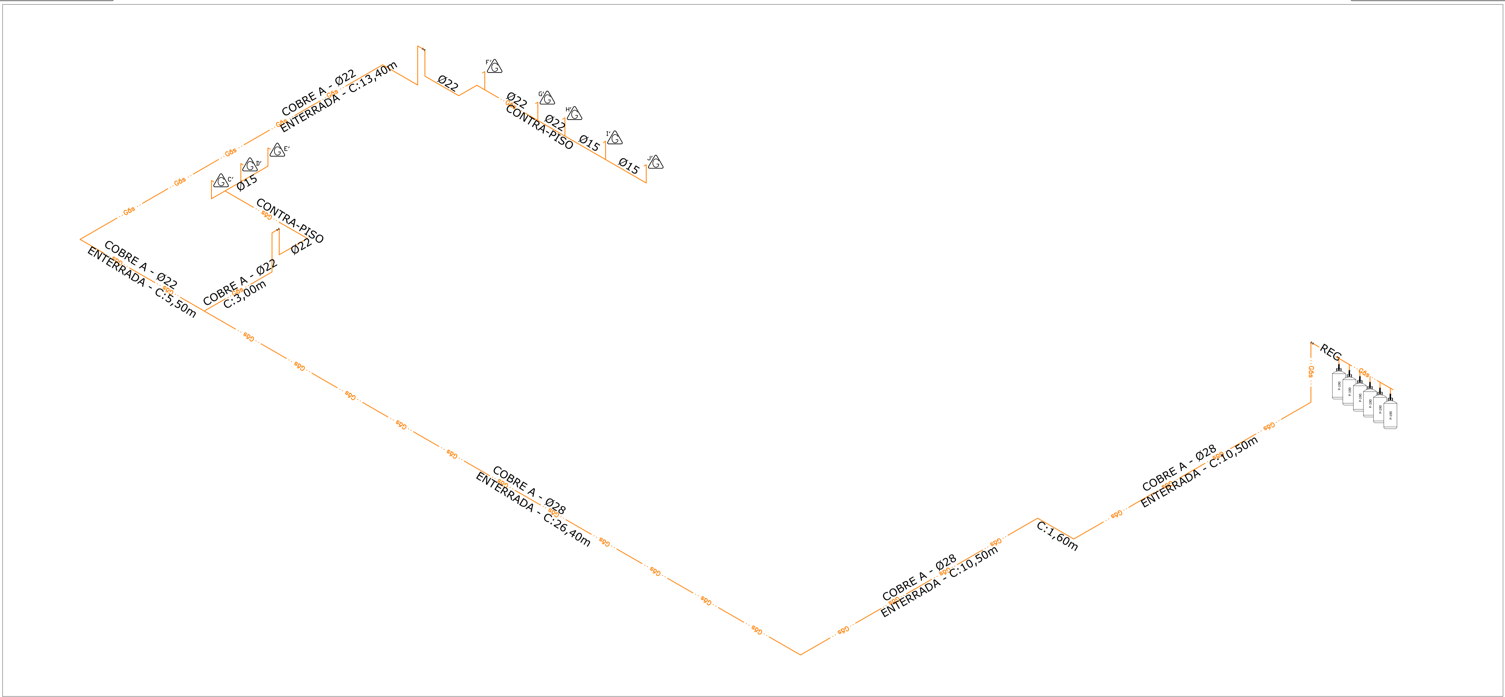
01 Representação Isométrica ESC.: 1:75
