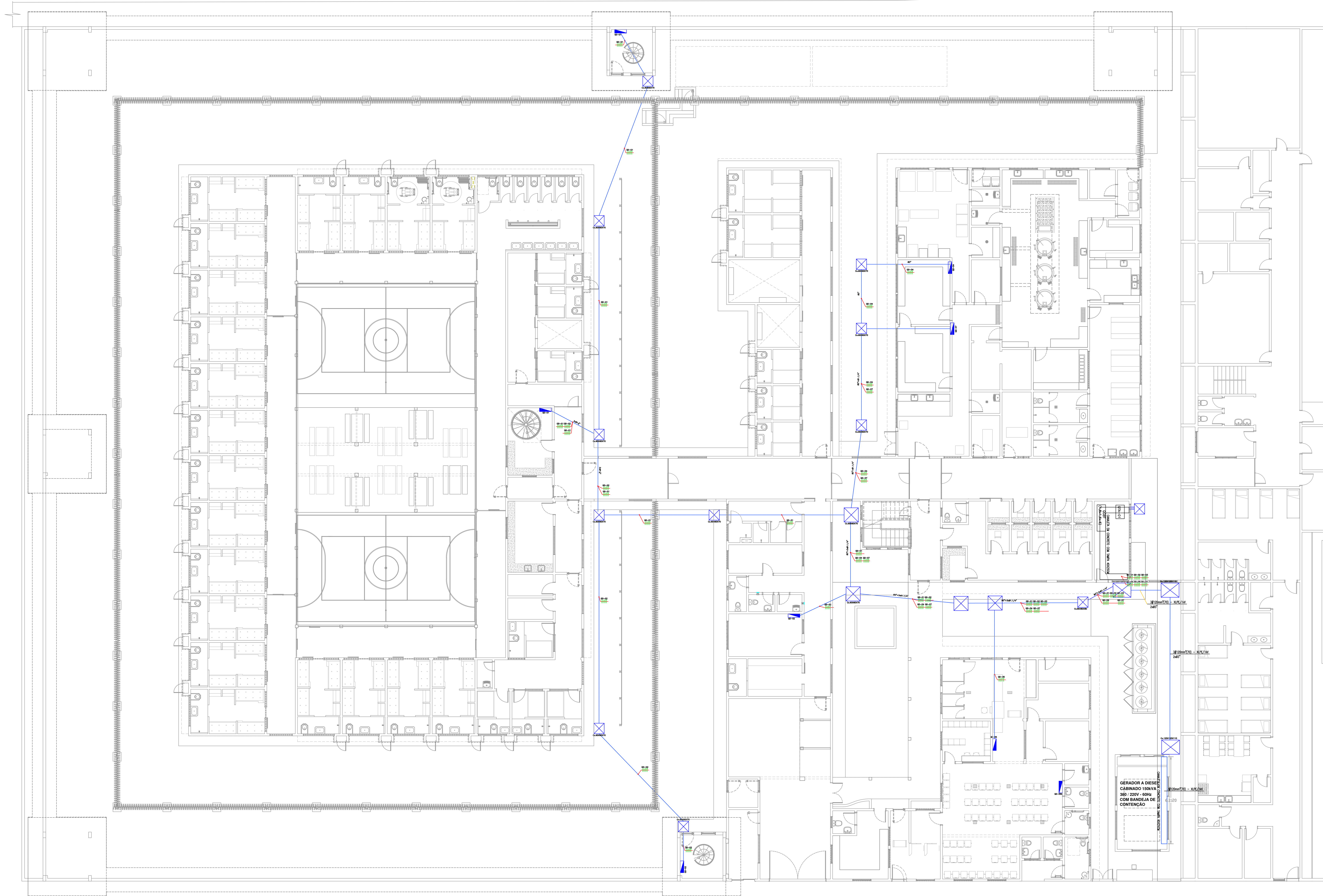
PLANTA BAIXA - ALIMENTADORES ESCALA: 1:100
