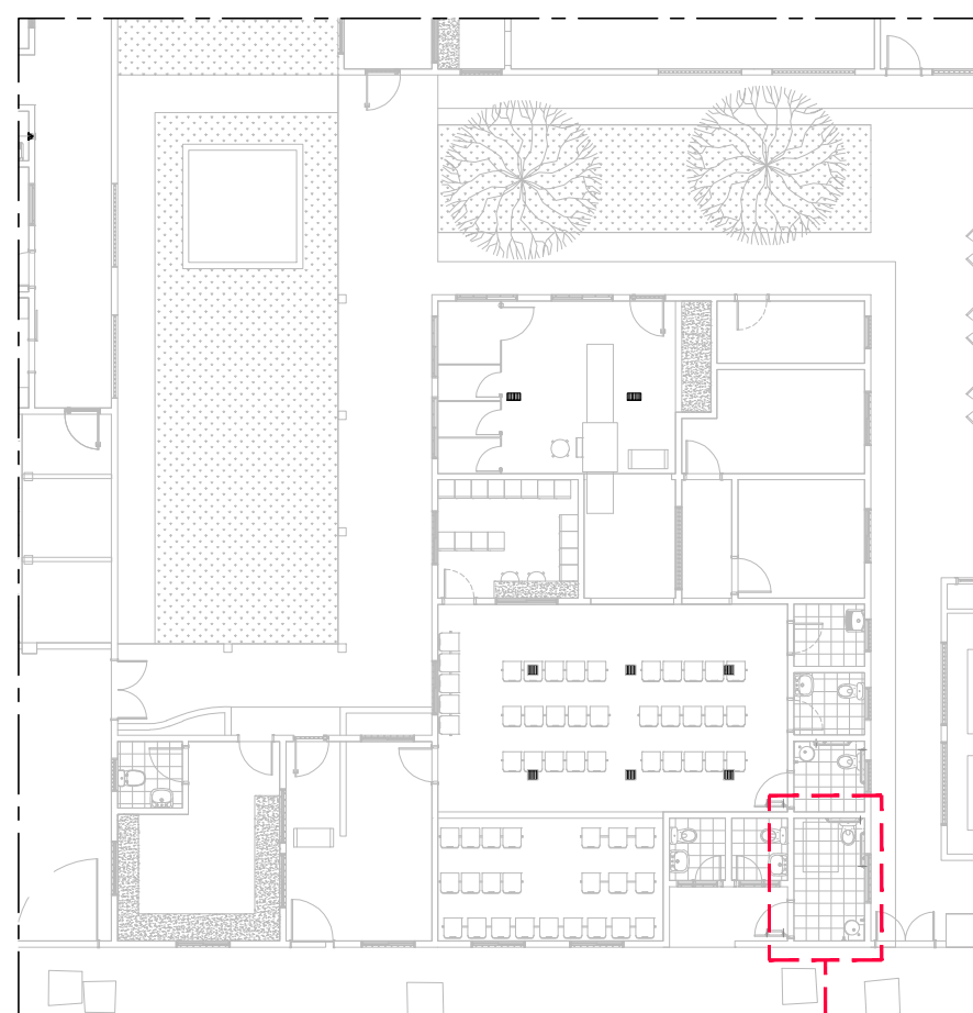
01 PLANTA DE LOCAÇÃO - PORTARIA ESCALA 1:200
