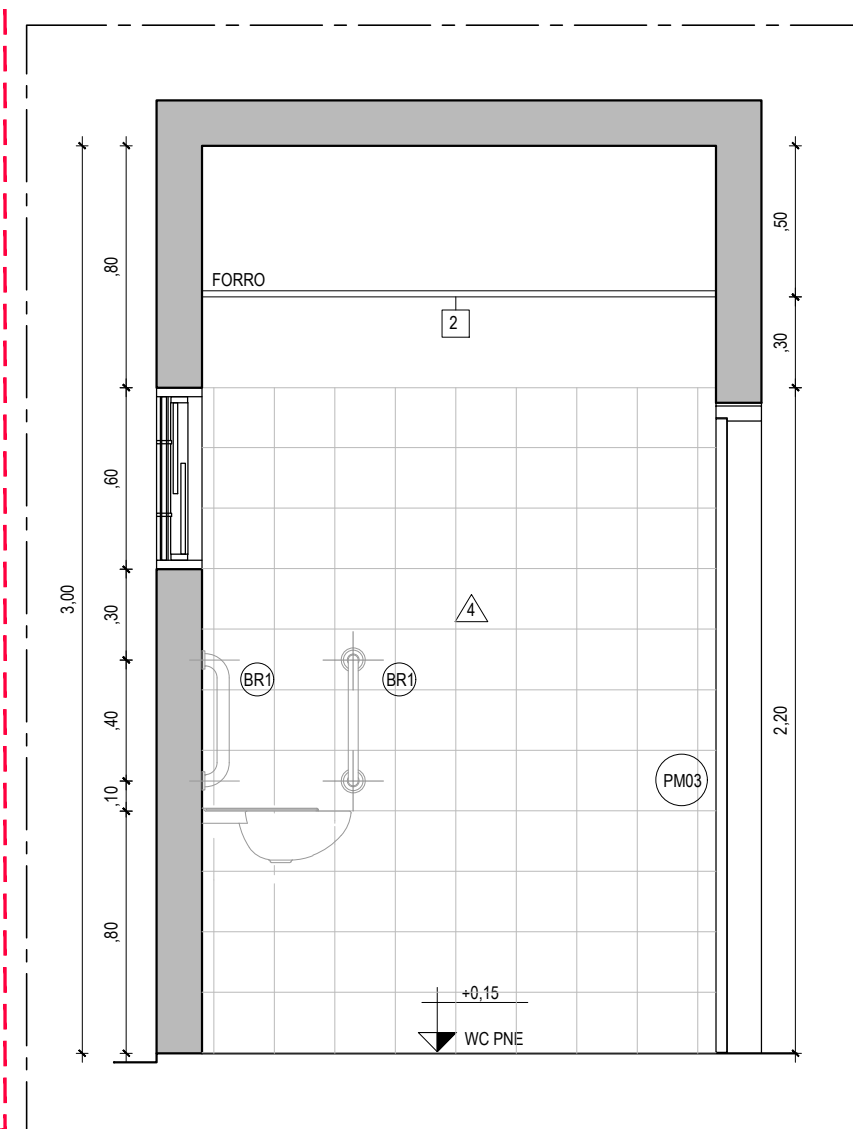
05 VISTA C - PNE ESCALA 1:25
