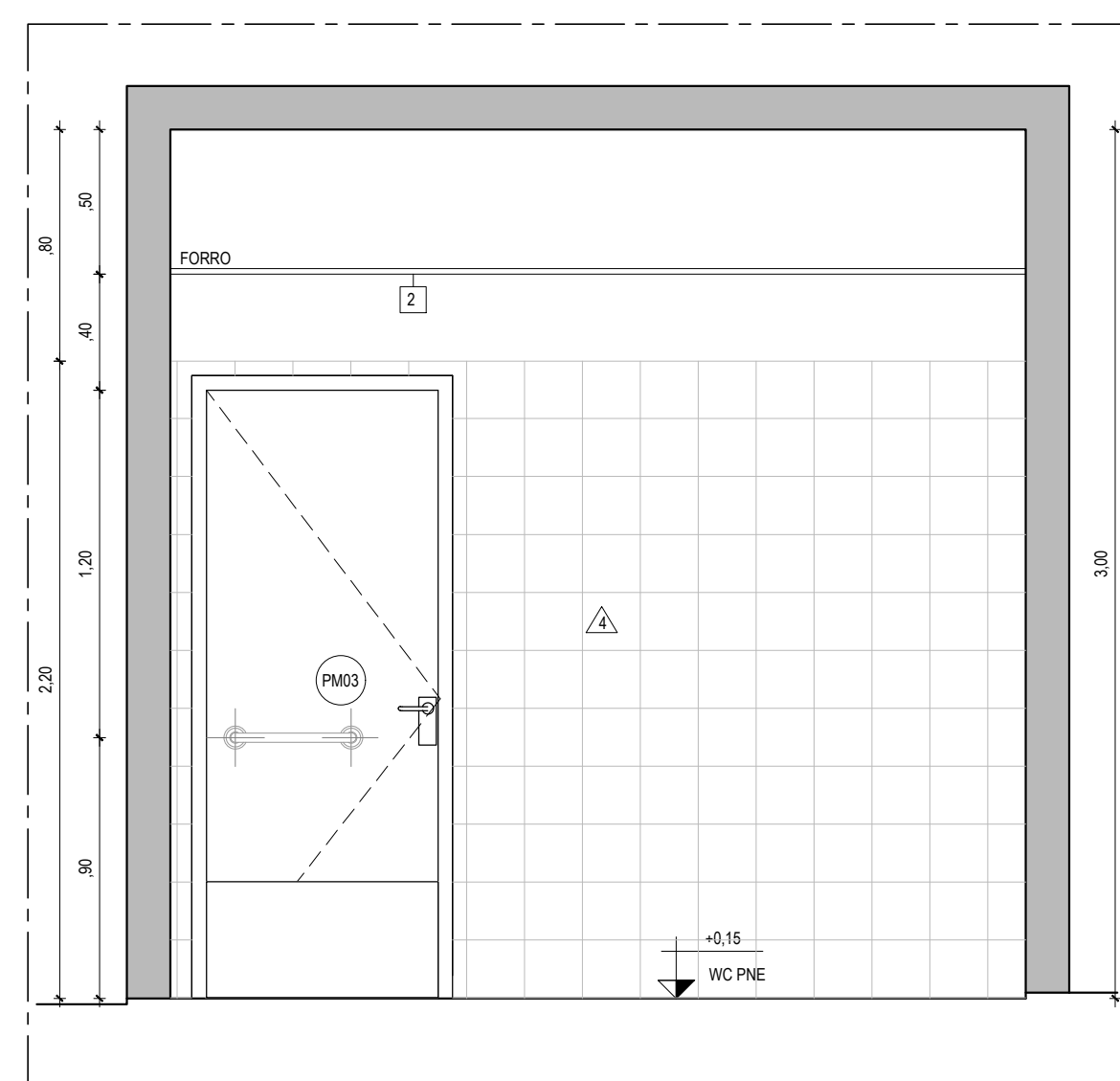
06 VISTA D - PNE ESCALA 1:25
