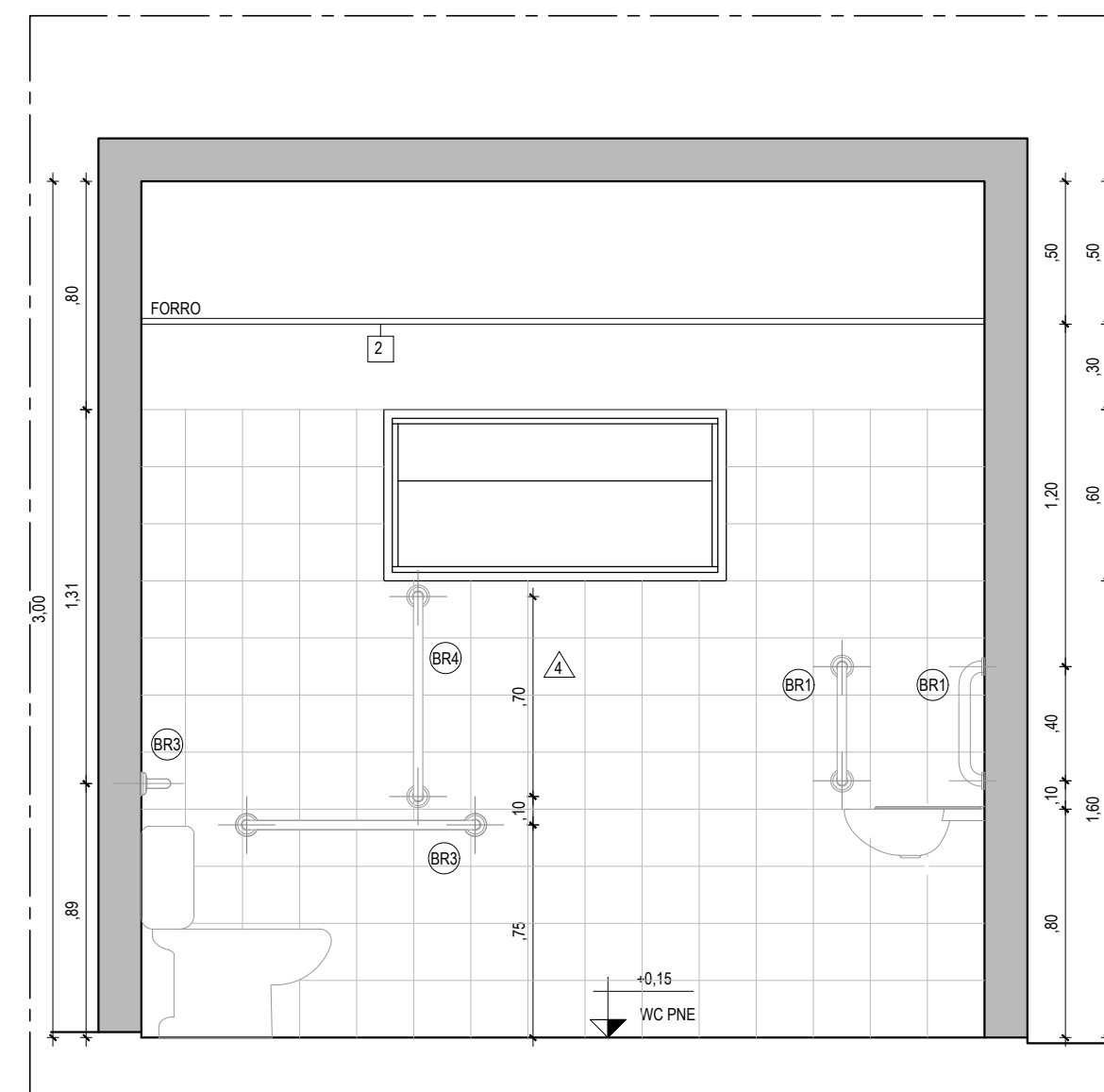
04 VISTA B - PNE ESCALA 1:25
