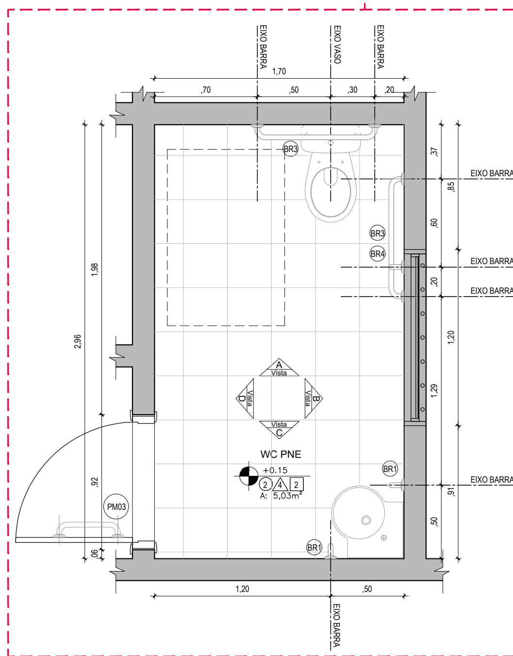
02 PLANA BAIXA ESCALA 1:25
