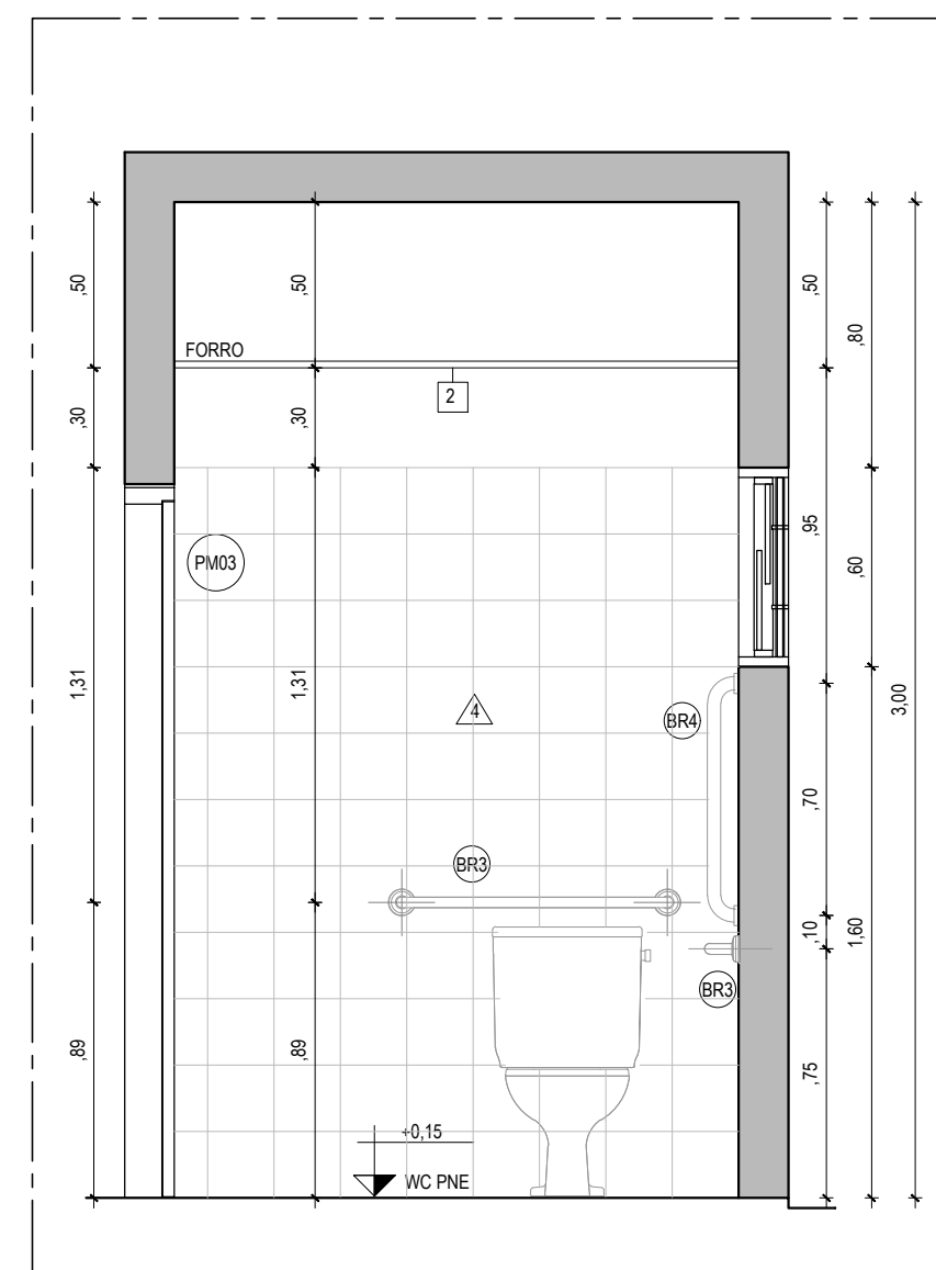
03 VISTA A - PNE ESCALA 1:25
