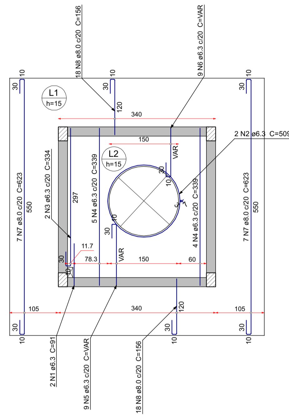
ARMAÇÃO POSITIVA DAS LAJES DO PAV. SUPERIOR (EIXO Y) ESCALA 1:50
