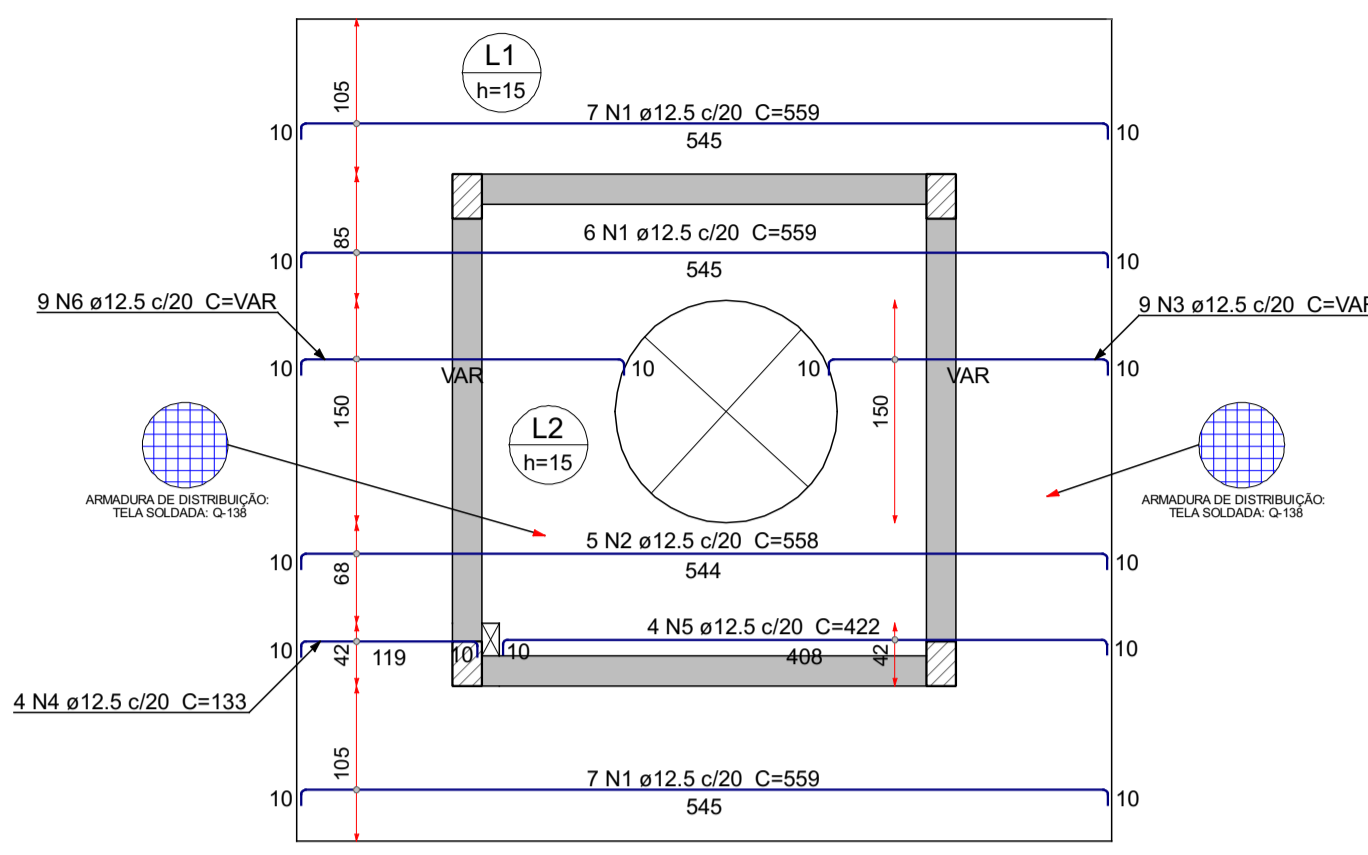
ARMAÇÃO NEGATIVA DAS LAJES DO PAV. SUPERIOR (EIXO X) ESCALA 1:50
