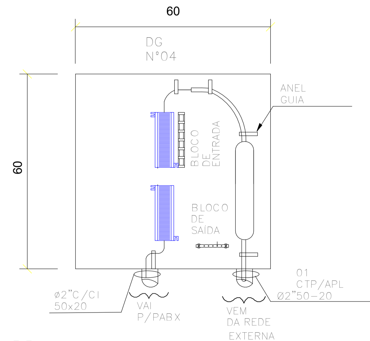
DG ESCALA: 1 : 50
