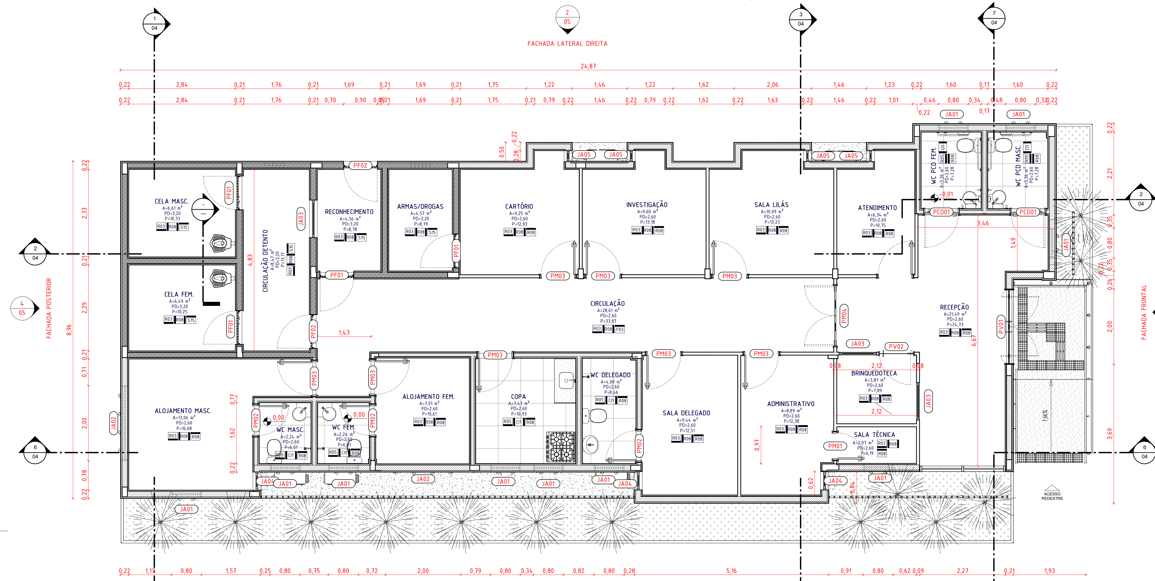
1 PLANTA BAIXA - TÉRREO 1 : 50
