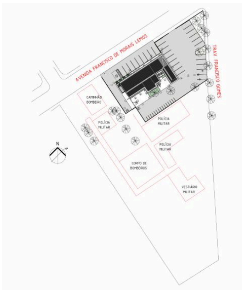
Bezerros: Planta de Situação – sem escala.
