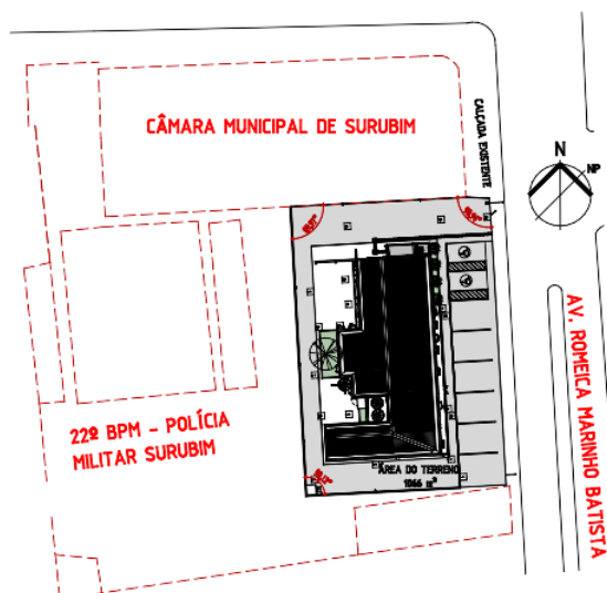
Surubim: Planta de Situação – sem escala.
