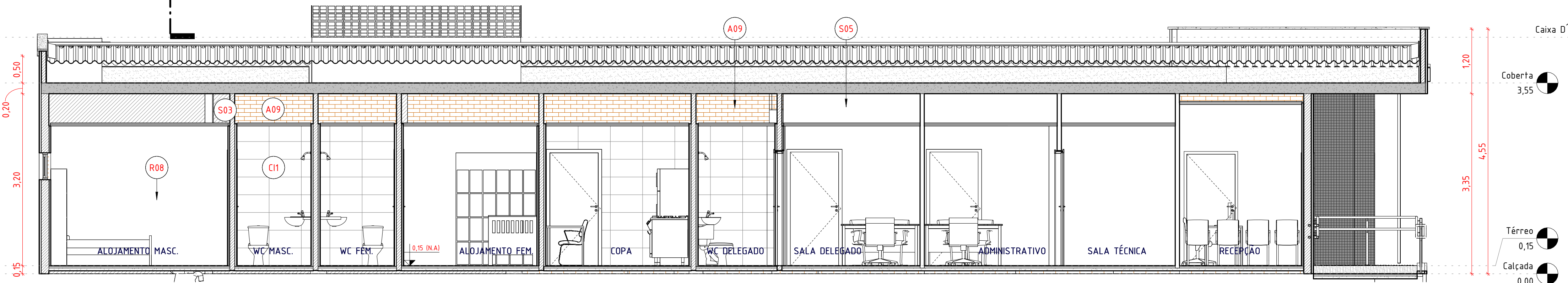
6 CORTE B 1 : 50
