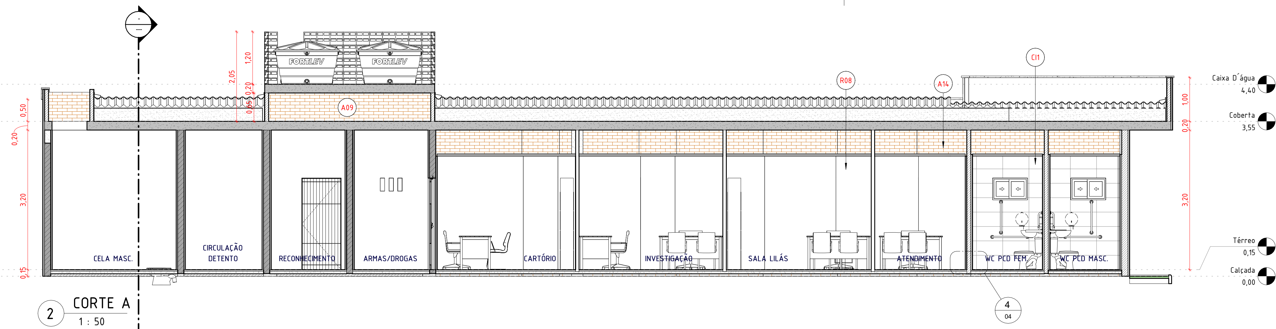
2 CORTE A 1 : 50
