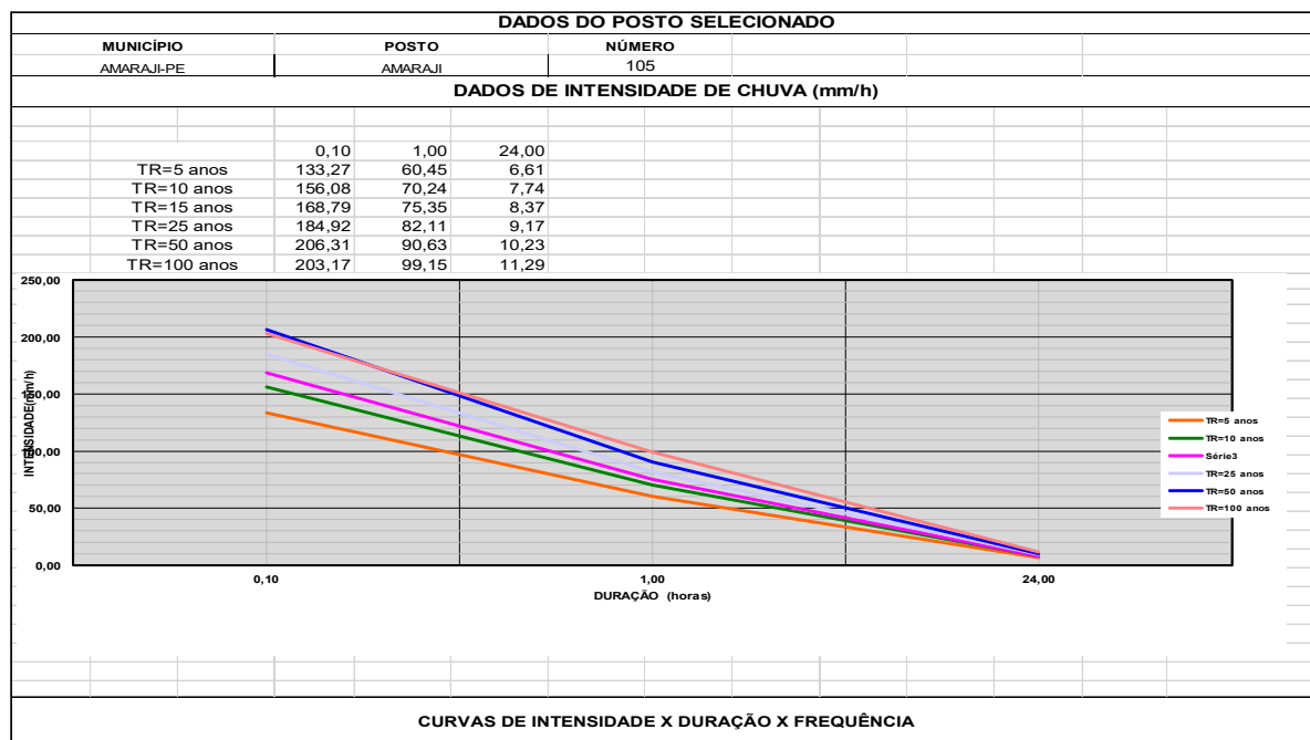
Figura EH-06: Curvas de Intensidade x Duração x Frequência
