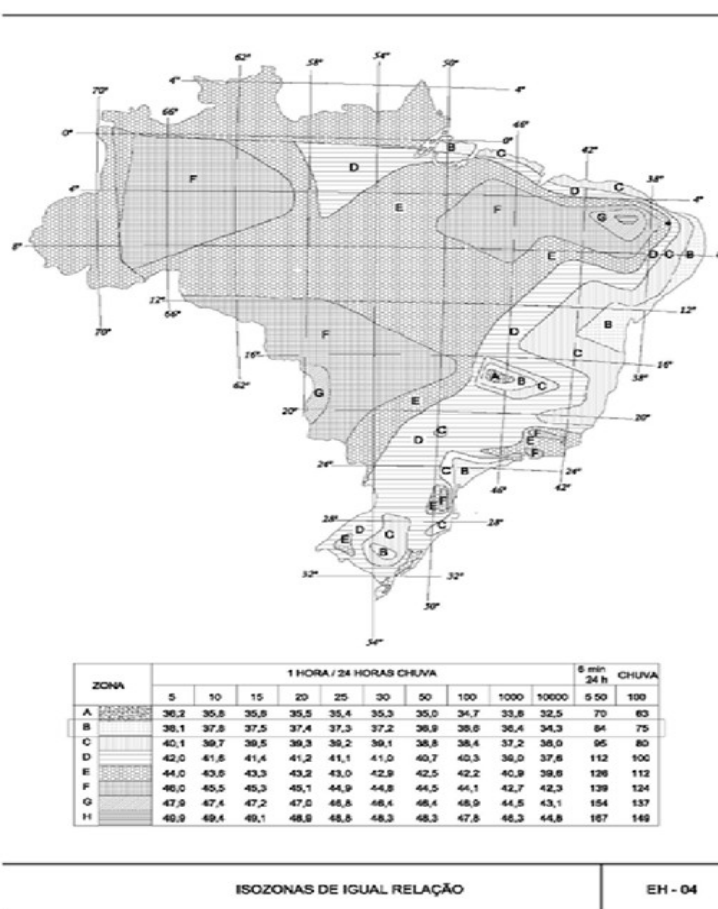
Figura EH-04: Mapa de Isozonas de Igual Relação
