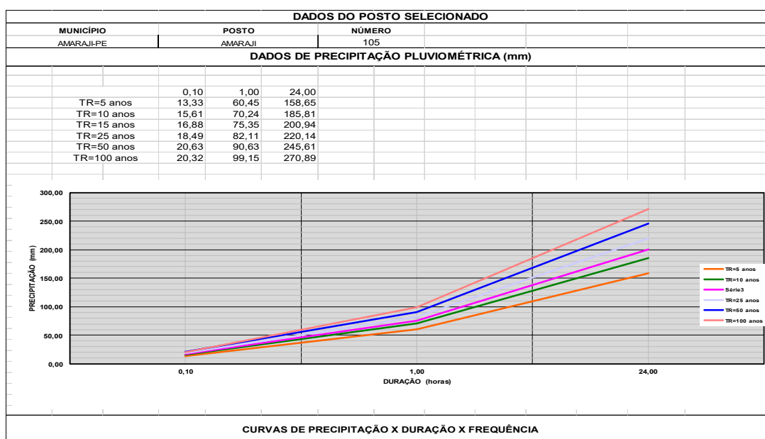
Figura EH-05: Curvas de Precipitação x Duração x Frequência
