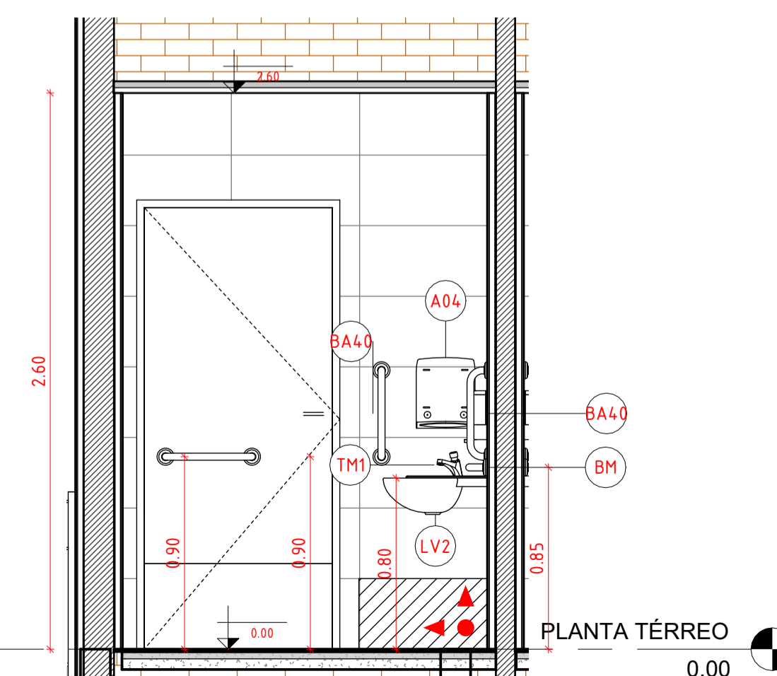
7 ELEVAÇÃO B - PCD FEM 1 : 25
