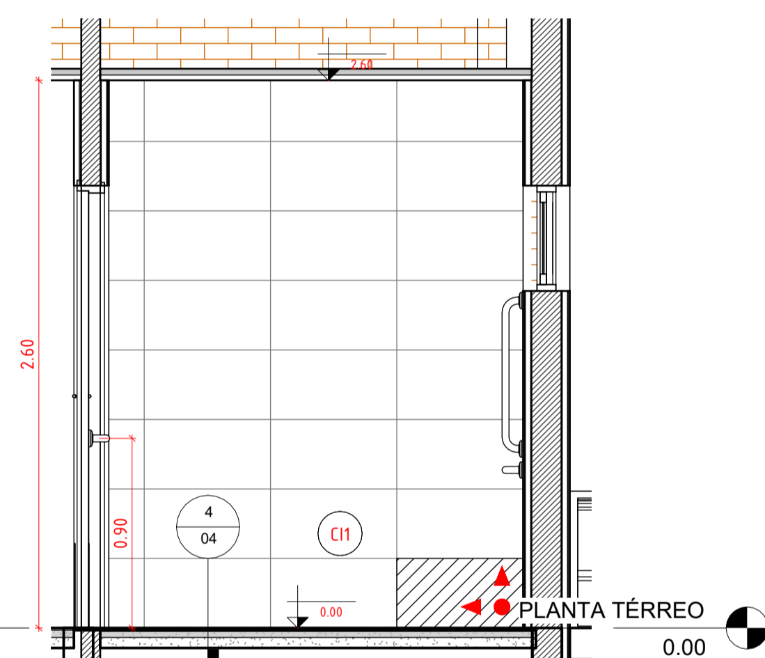
4 ELEVAÇÃO C - PCD MASC 1 : 25
