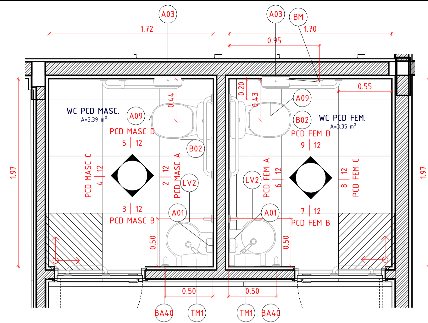
1 WC PCD MAS/FEM 1 : 25
