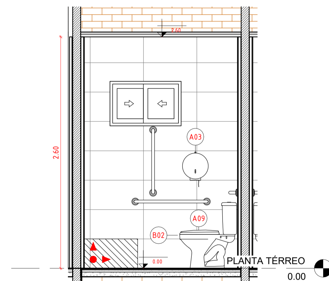
5 ELEVAÇÃO D - PCD MASC 1 : 25
