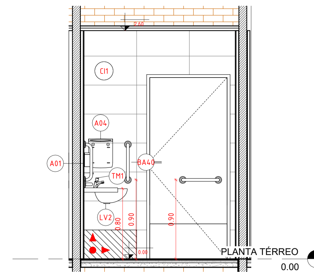
3 ELEVAÇÃO B - PCD MASC 1 : 25
