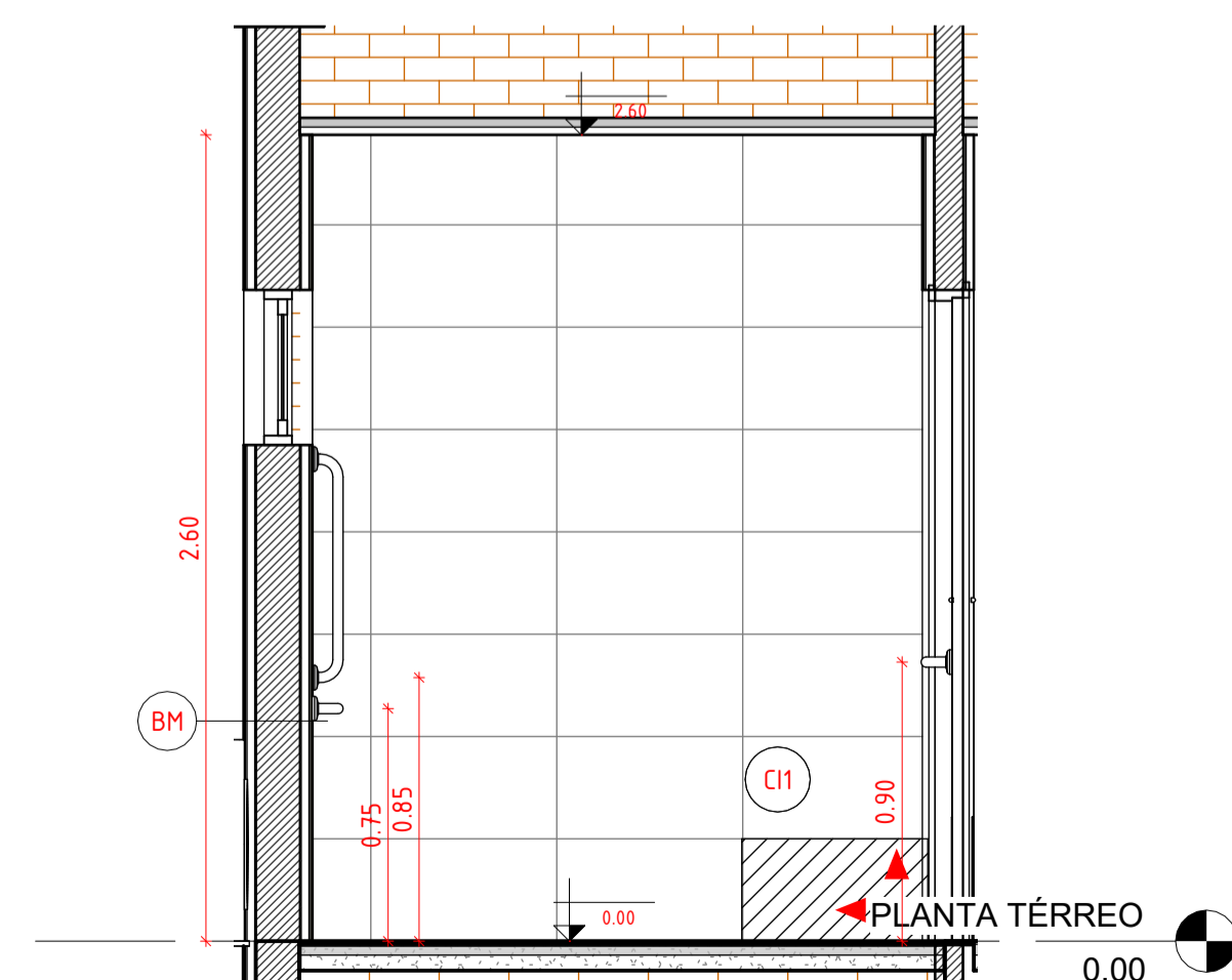
8 ELEVAÇÃO C - PCD FEM 1 : 25
