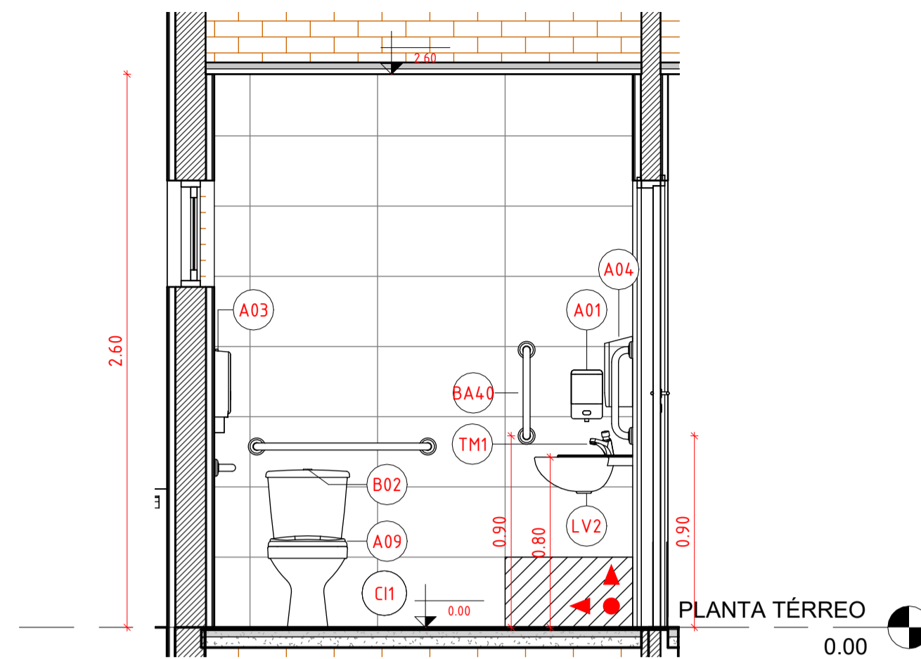
2 ELEVAÇÃO A - PCD MASC 1 : 25
