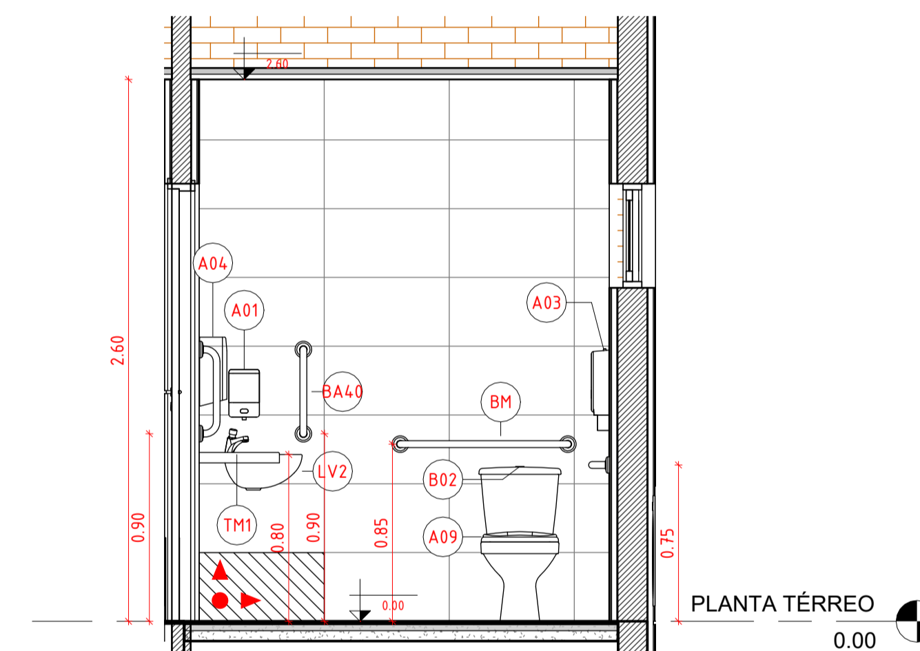
6 ELEVAÇÃO A - PCD FEM 1 : 25
