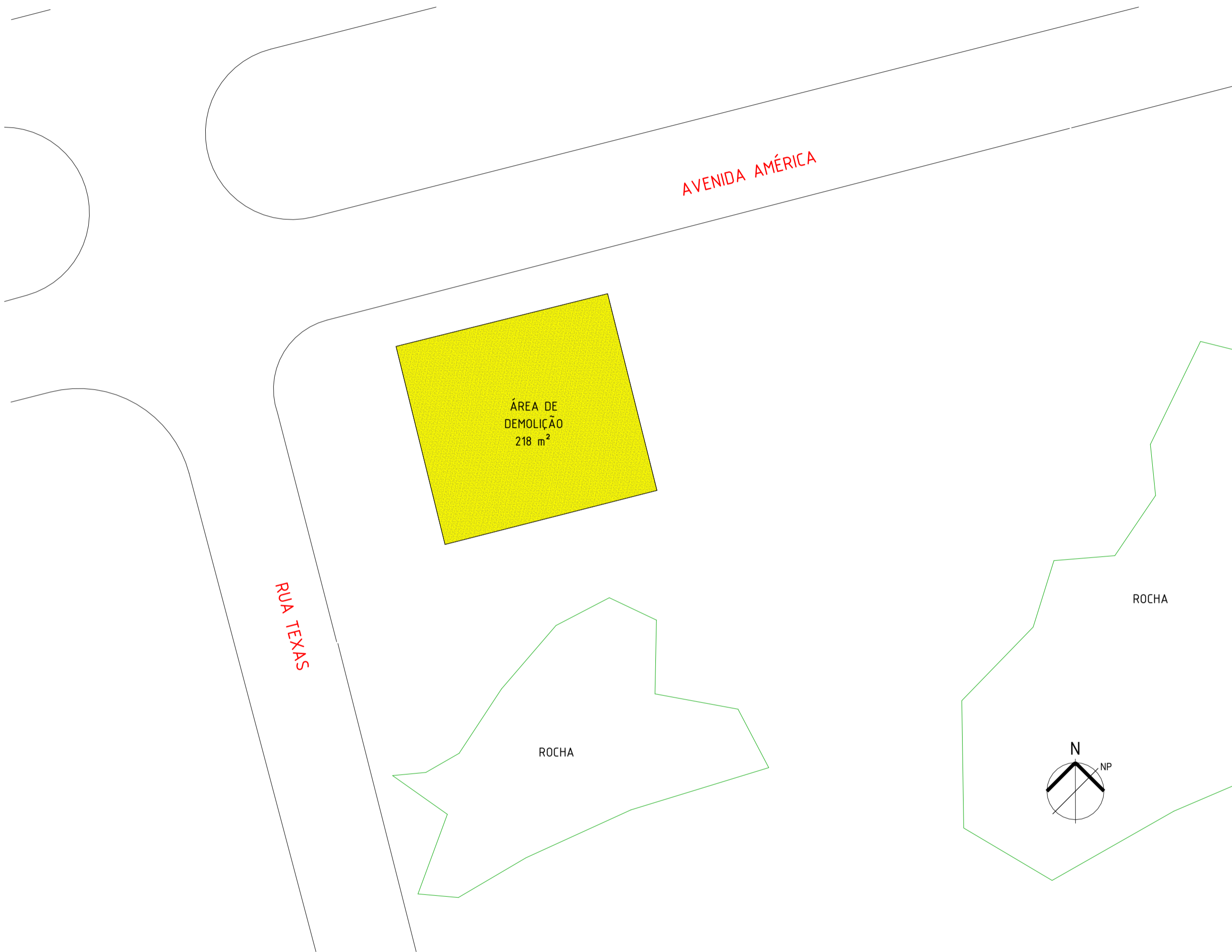
1 PLANTA DE DEMOLIÇÃO 1 : 250
