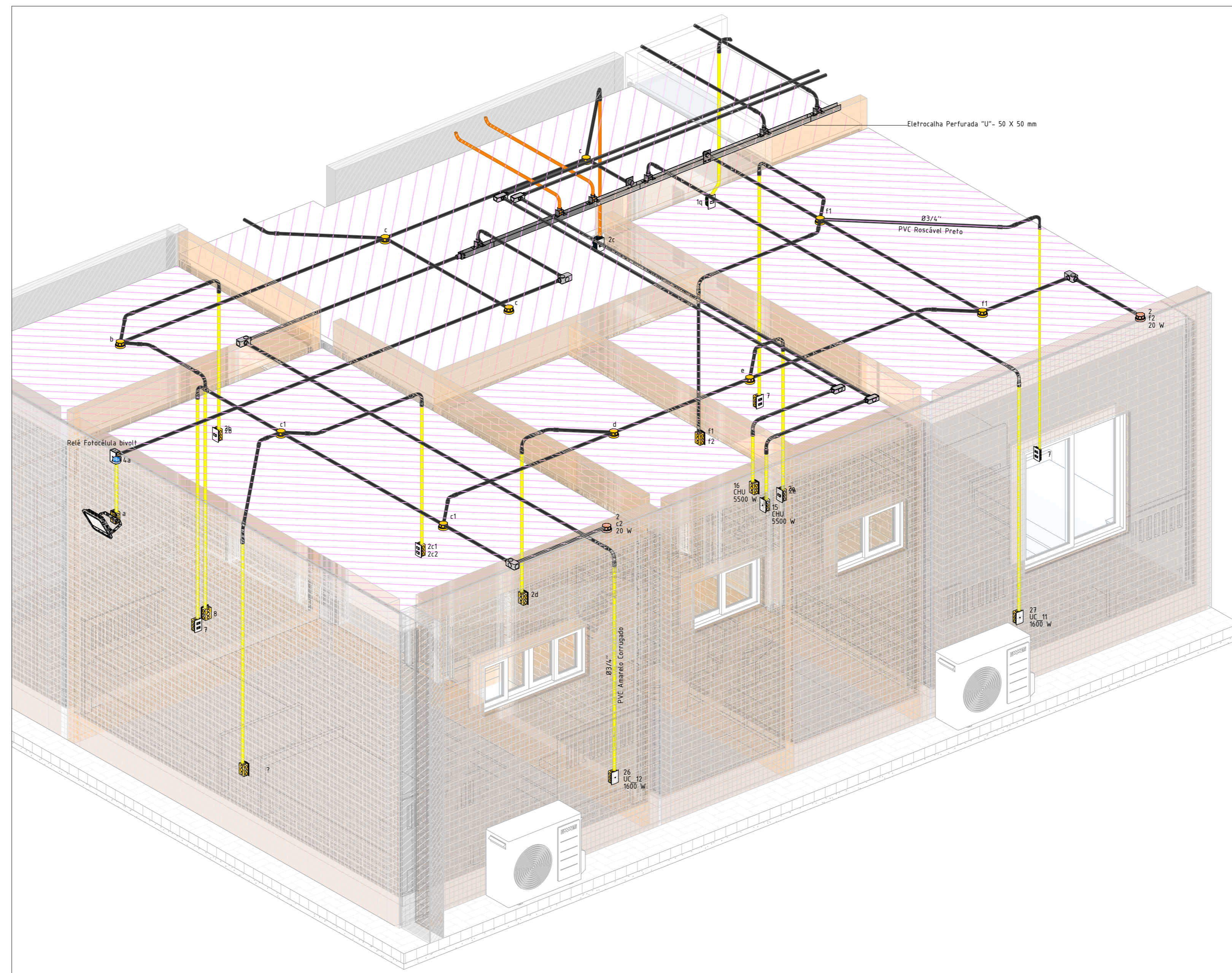
ISOMÉTRICO 04 ESCALA:
