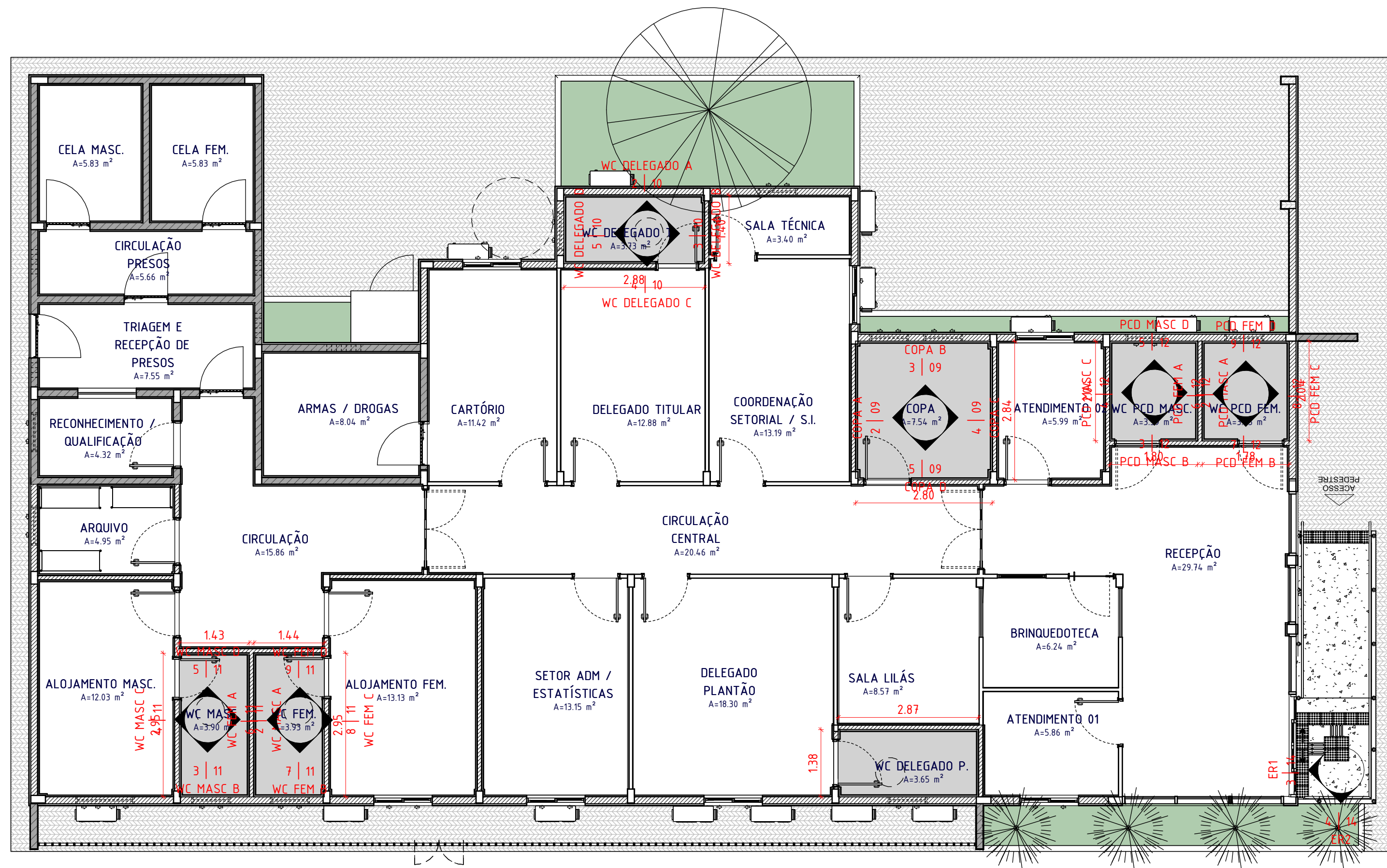
1 IMPERMEABILIZAÇÃO 1 : 75
