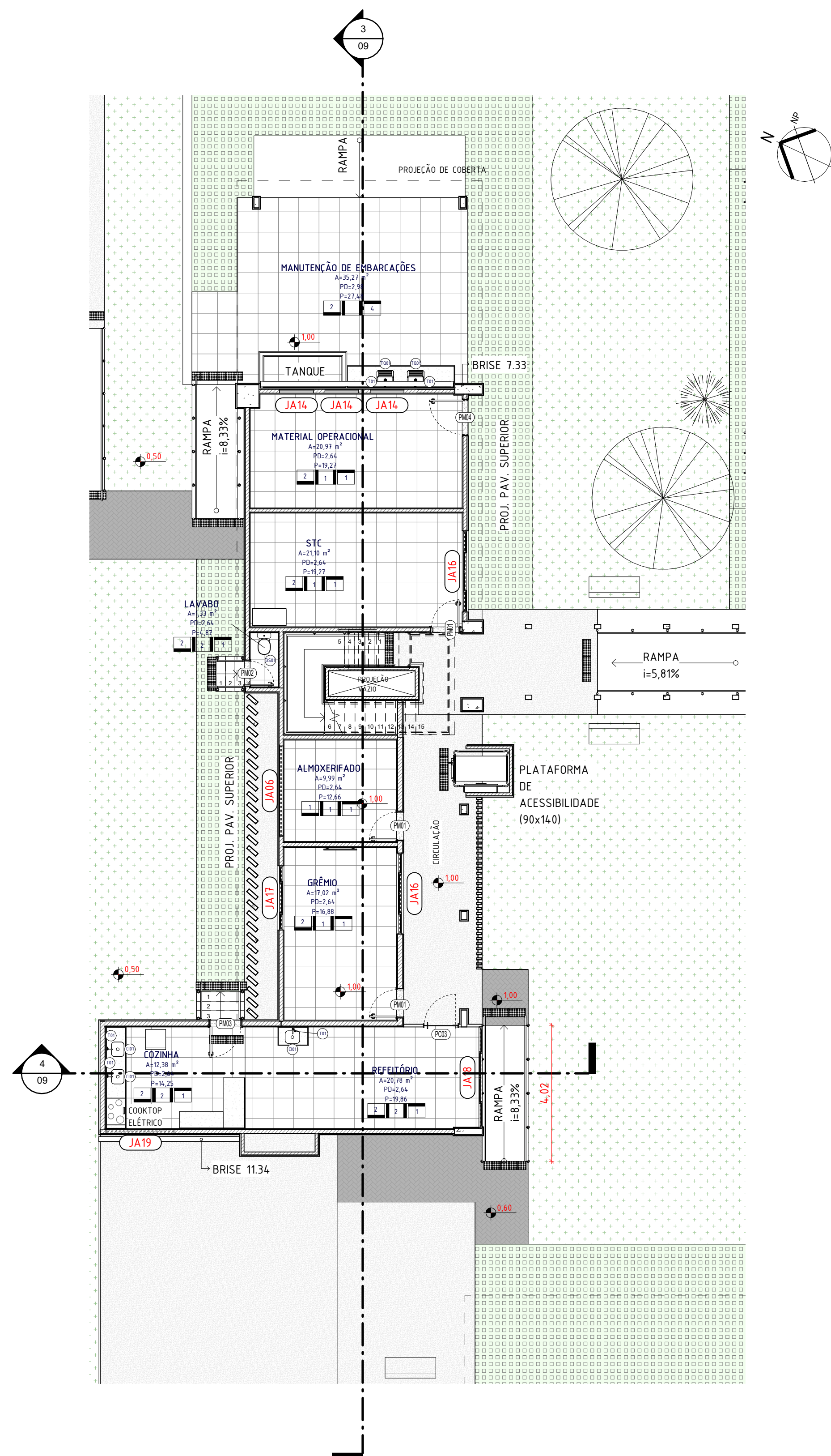
1 TÉRREO CASA 02 1 : 100
