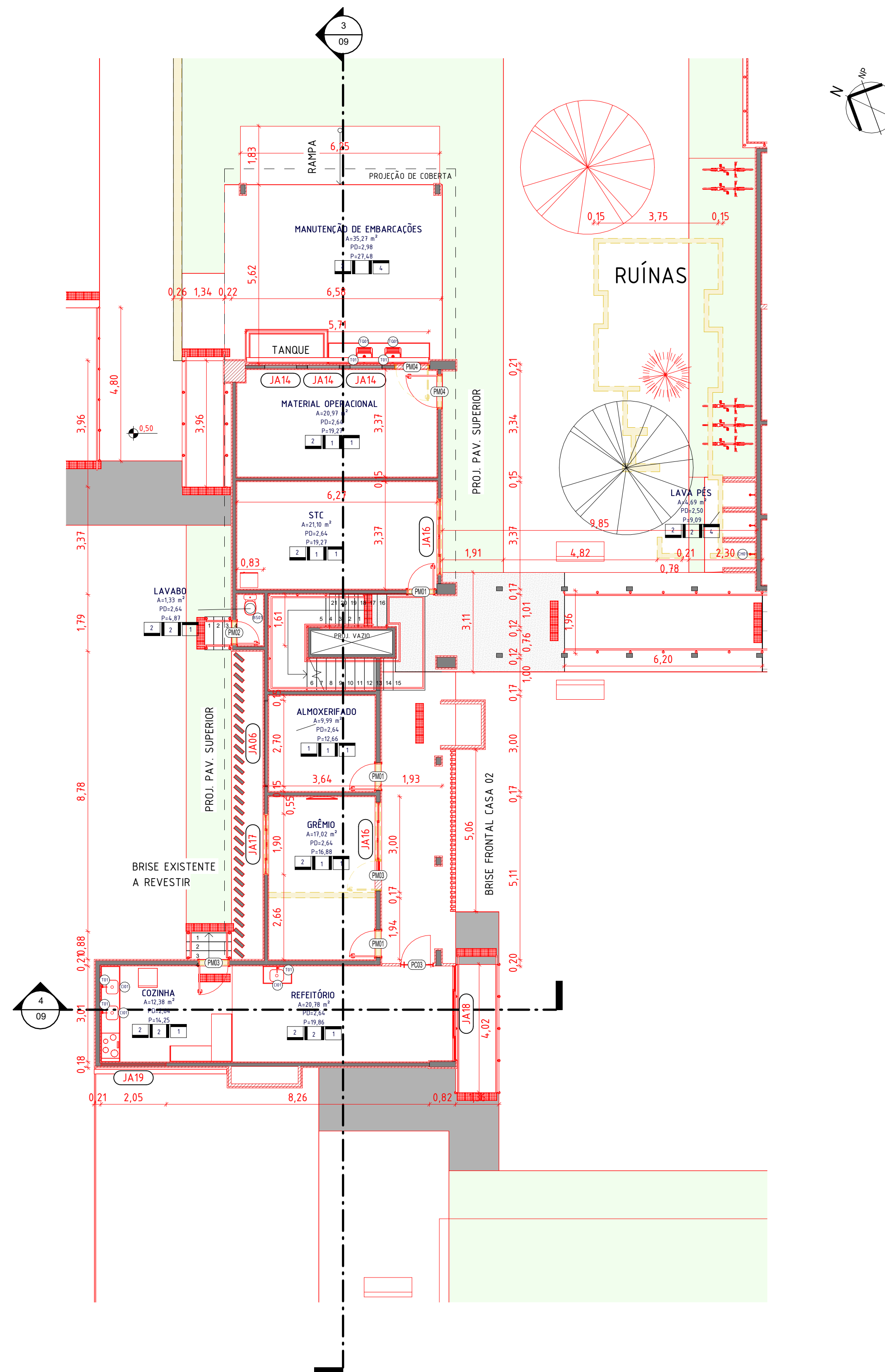
2 TÉRREO CASA 02 DEMOLIR E CONSTRUIR 1 : 100
