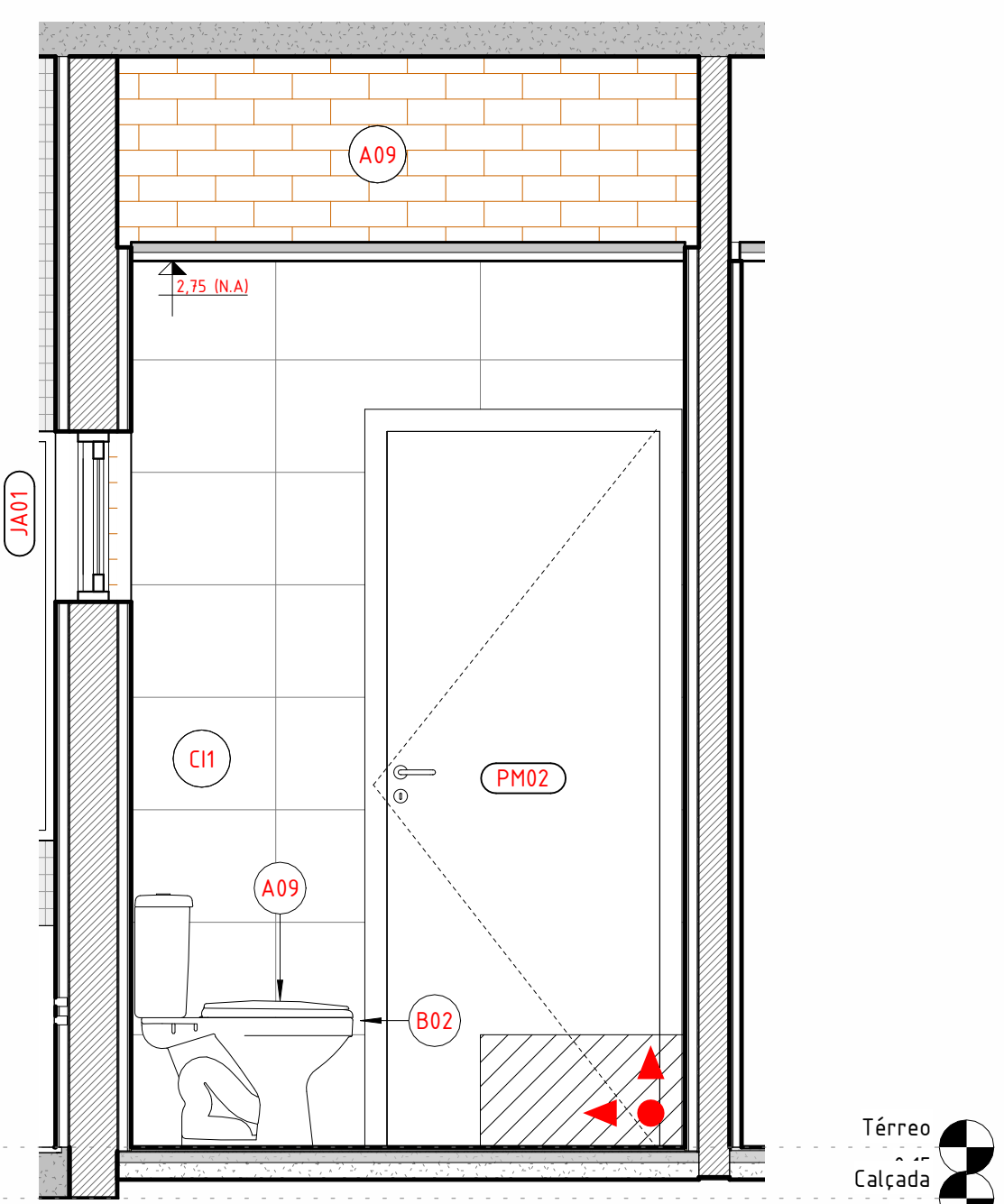
4 ELEV. ALOJ. MASC. C 1 : 20
