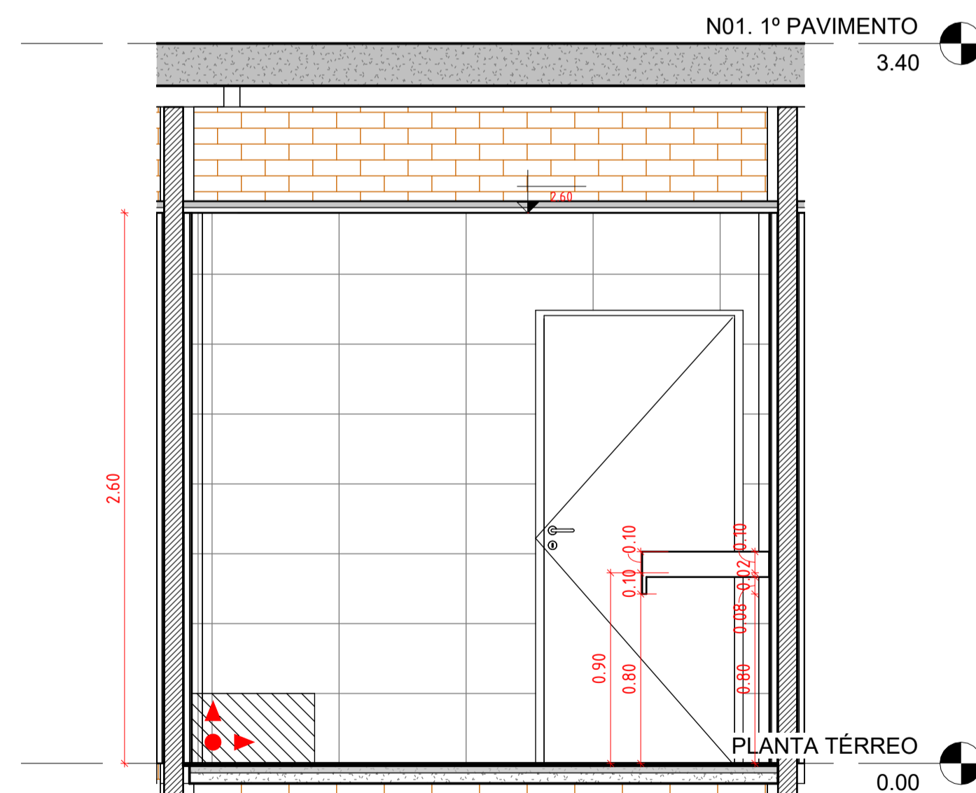
5 ELEVAÇÃO D - COPA 1 : 25
