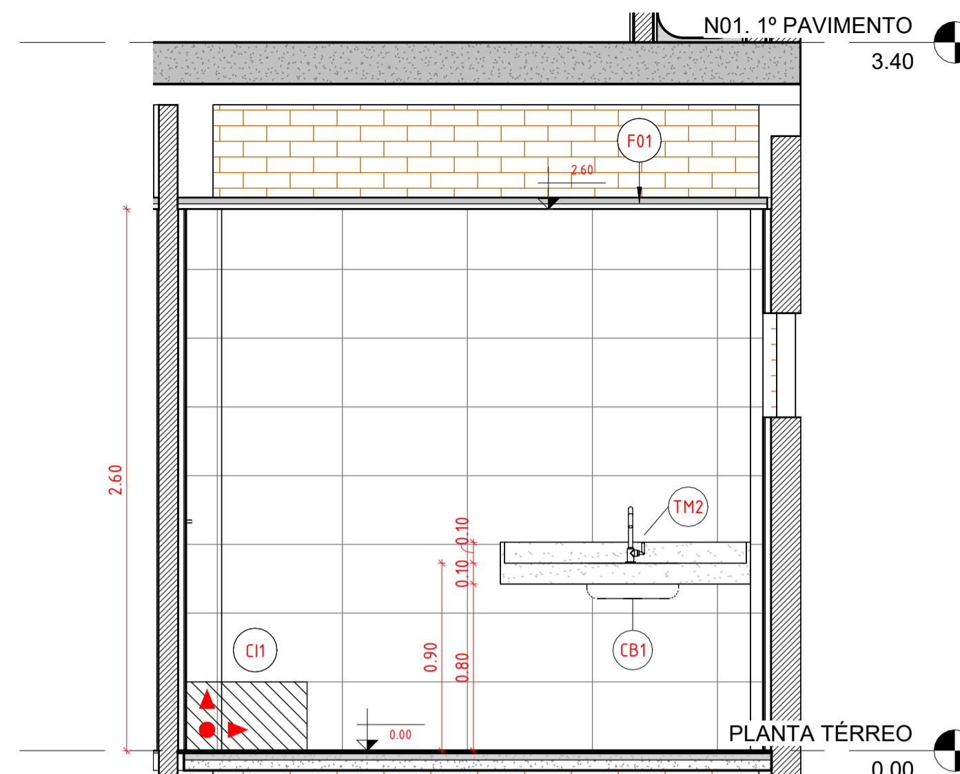
2 ELEVAÇÃO A - COPA 1 : 25
