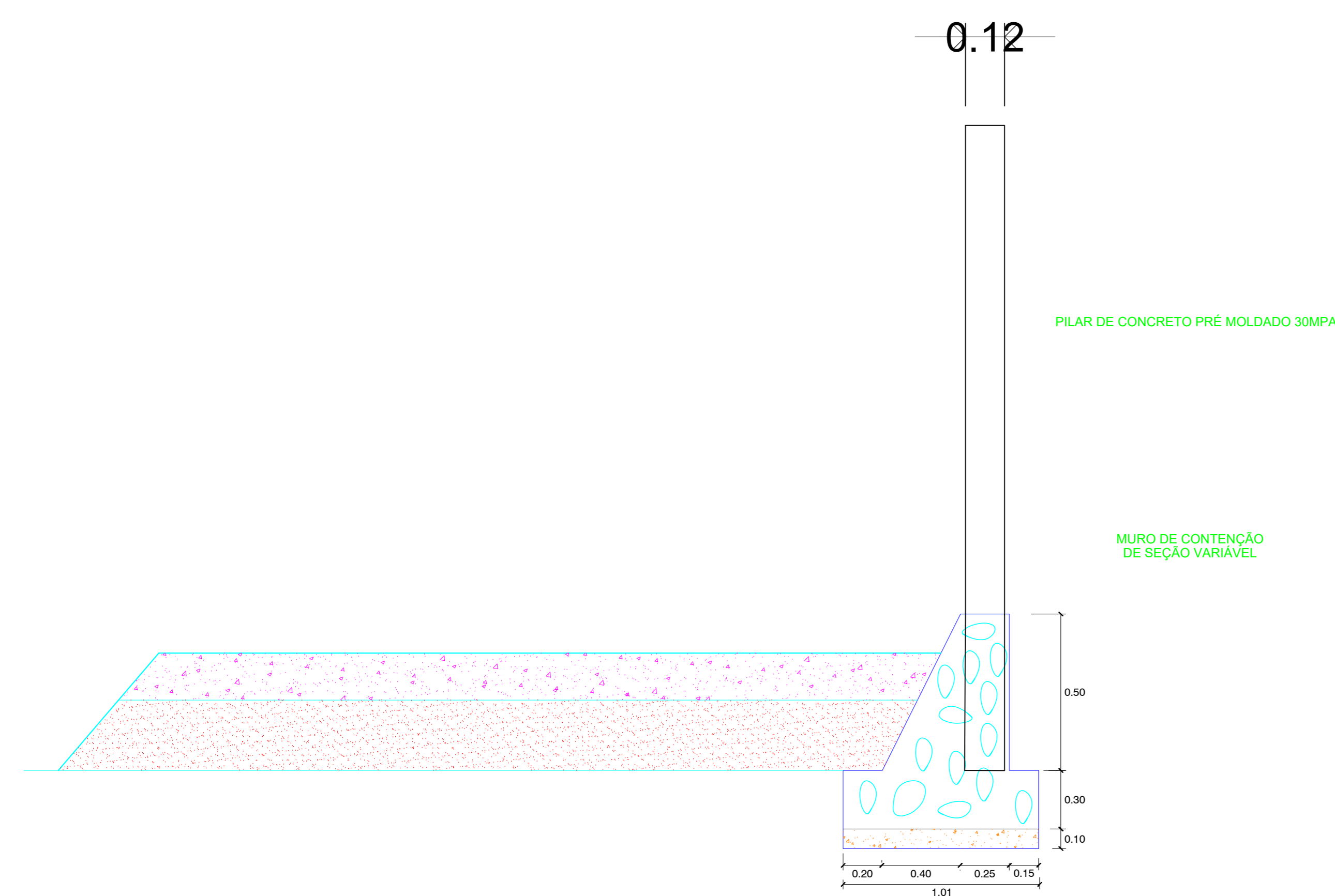
DETALLE MURO DE CONTEÇÃO
