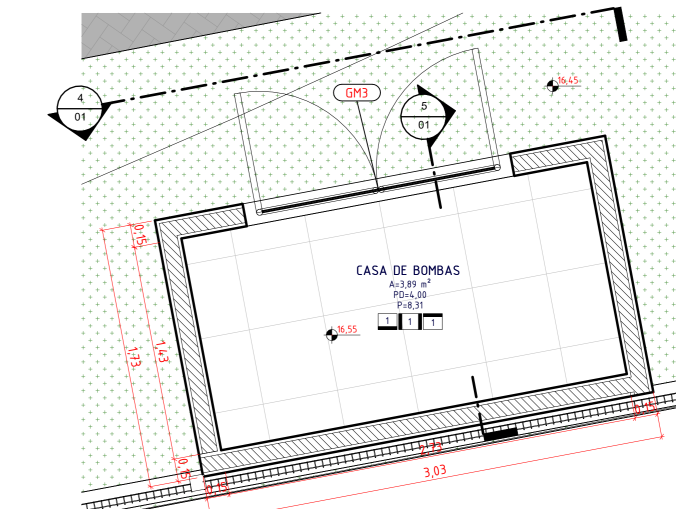
3 CASA DE BOMBAS 1 : 25
