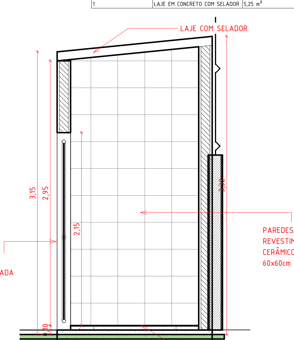
5 CORTE 2 - CASA DE BOMBAS 1 : 25
