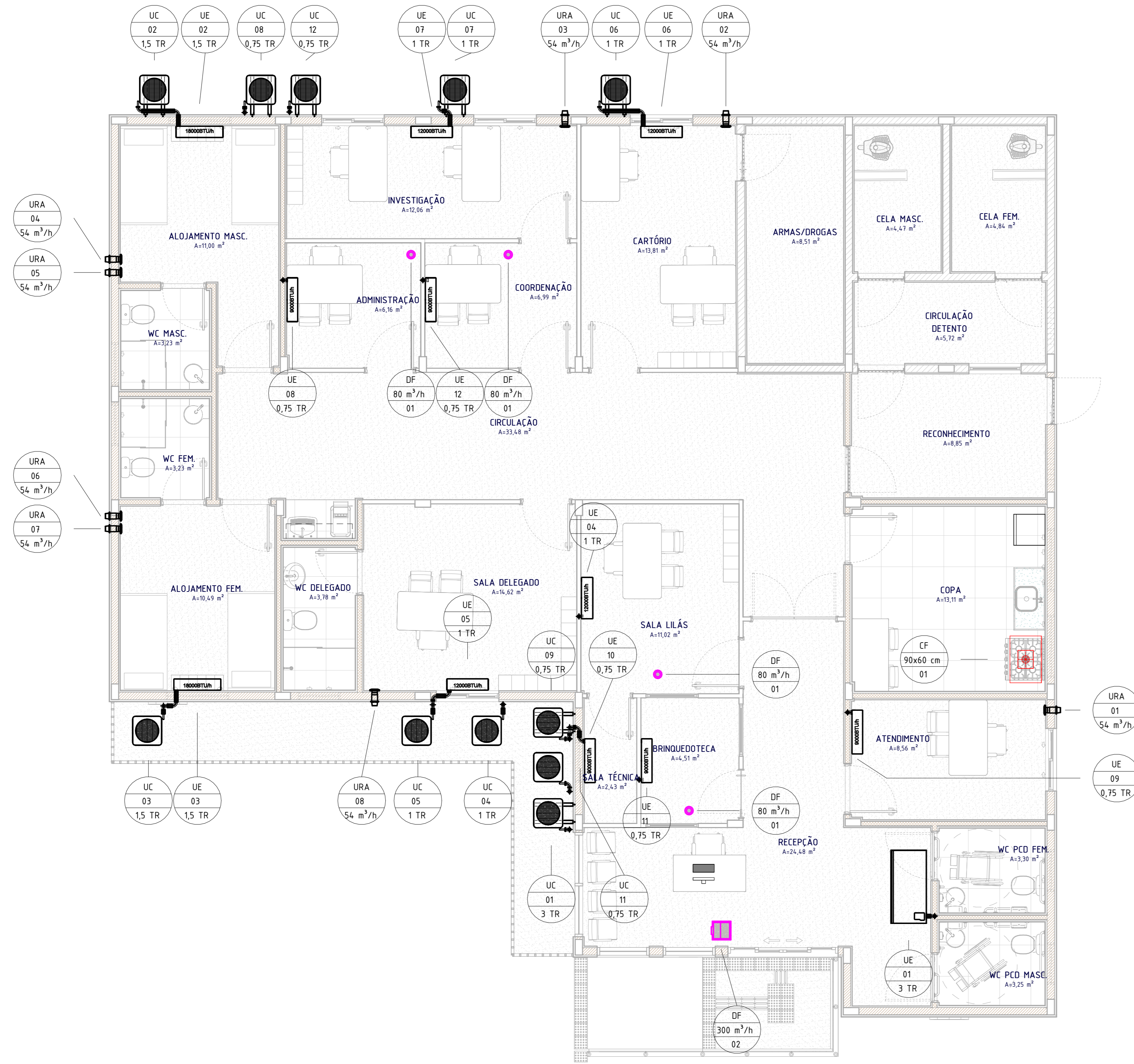
1 PLANTA BAIXA - TÉRREO 1 : 50
