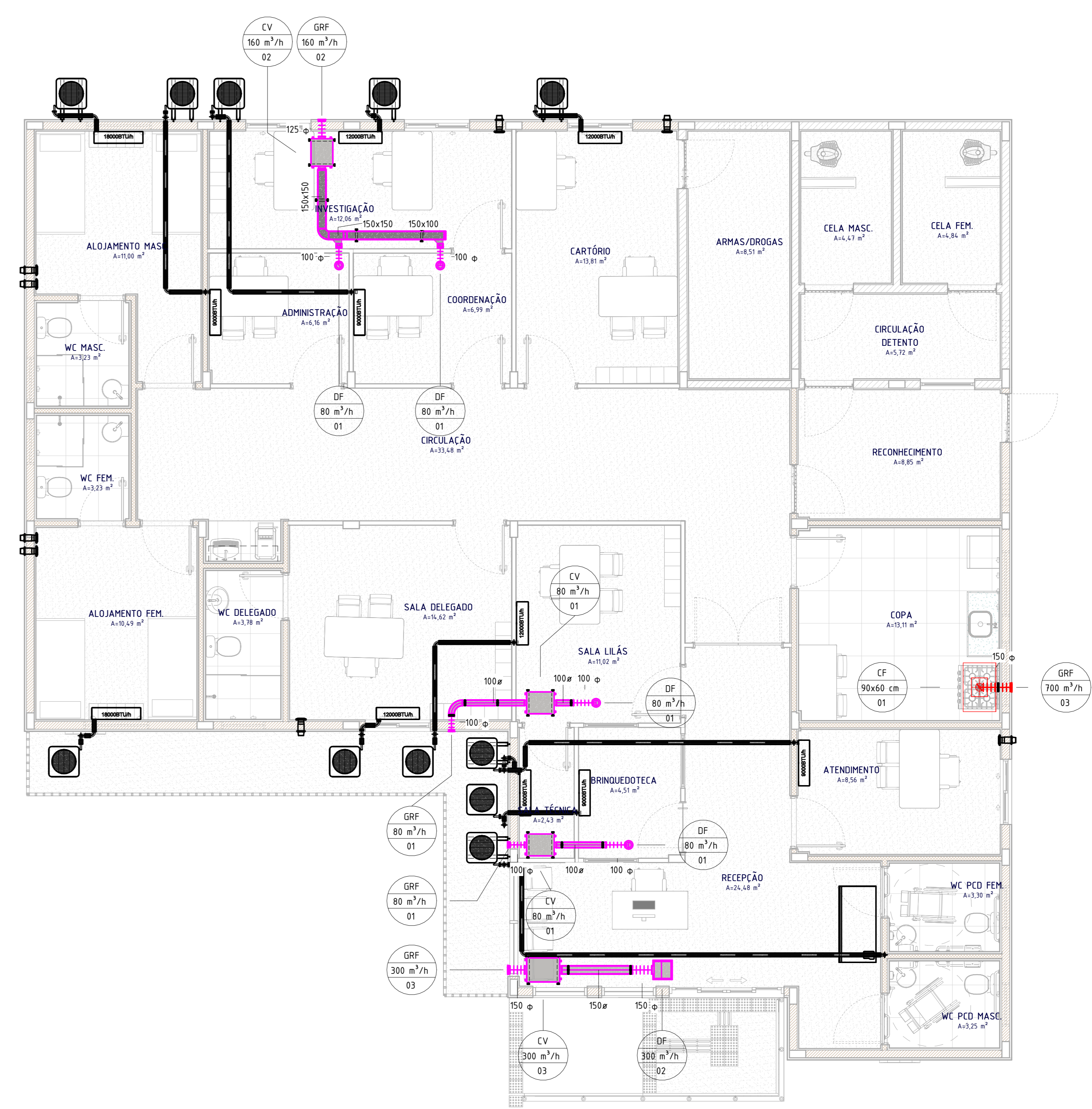
2 PLANTA BAIXA - TÉRREO - ENTREFORRO 1 : 50
