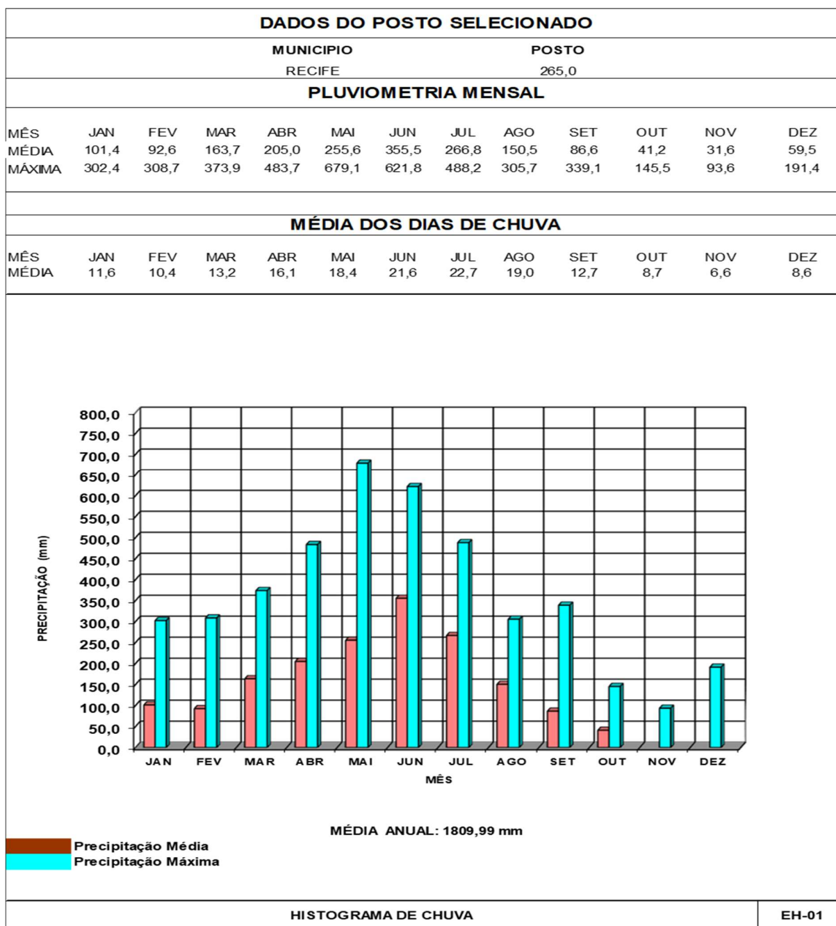
Figura EH-01: Histograma de chuva
