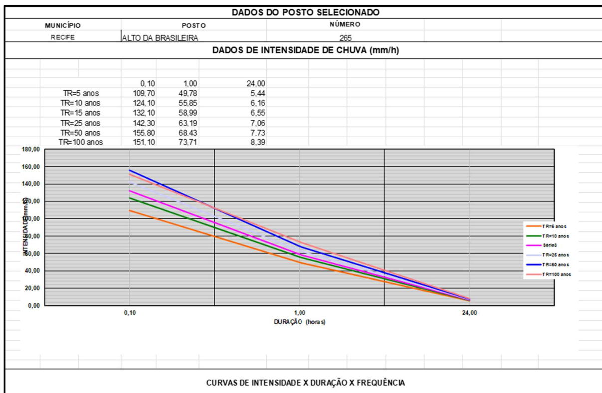
Figura EH-06: Curvas de Intensidade x Duração x Frequência
