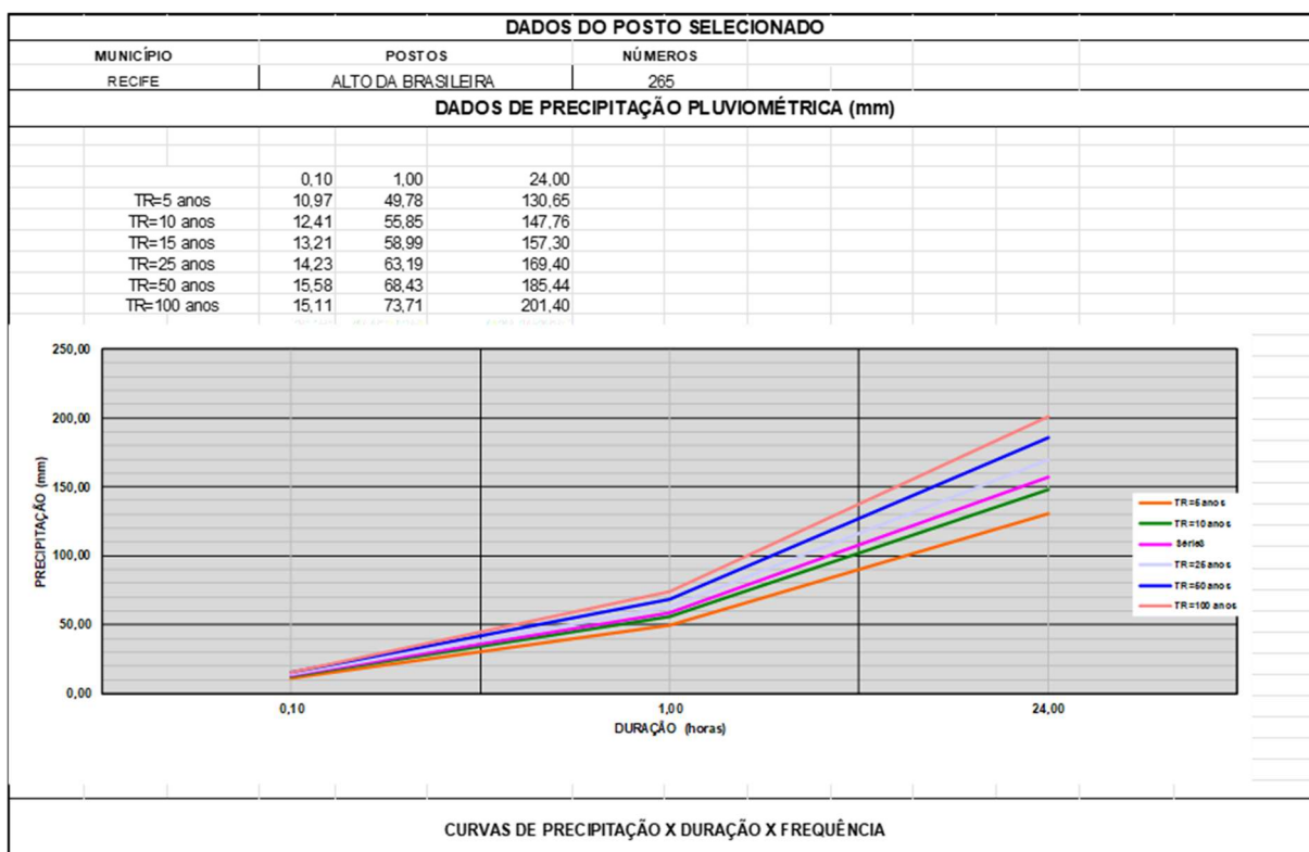
Figura ÉH-05: Curvas de Precipitação x Duração x Frequência
