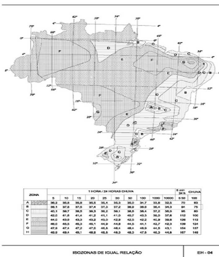
Figura: EH-04: Mapa de Isozonas de Igual Relação
