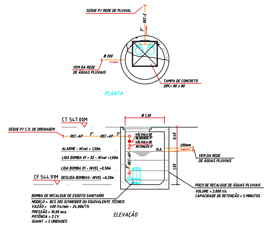
DET. POÇO DE RECALQUE ÁGUAS PLUVIAIS ESC. 1:150
