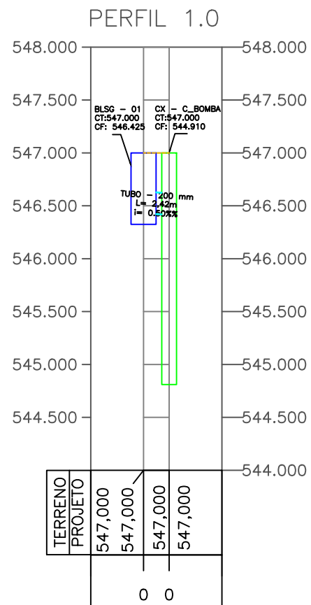
DET. PERFIL ESC. 1:500
