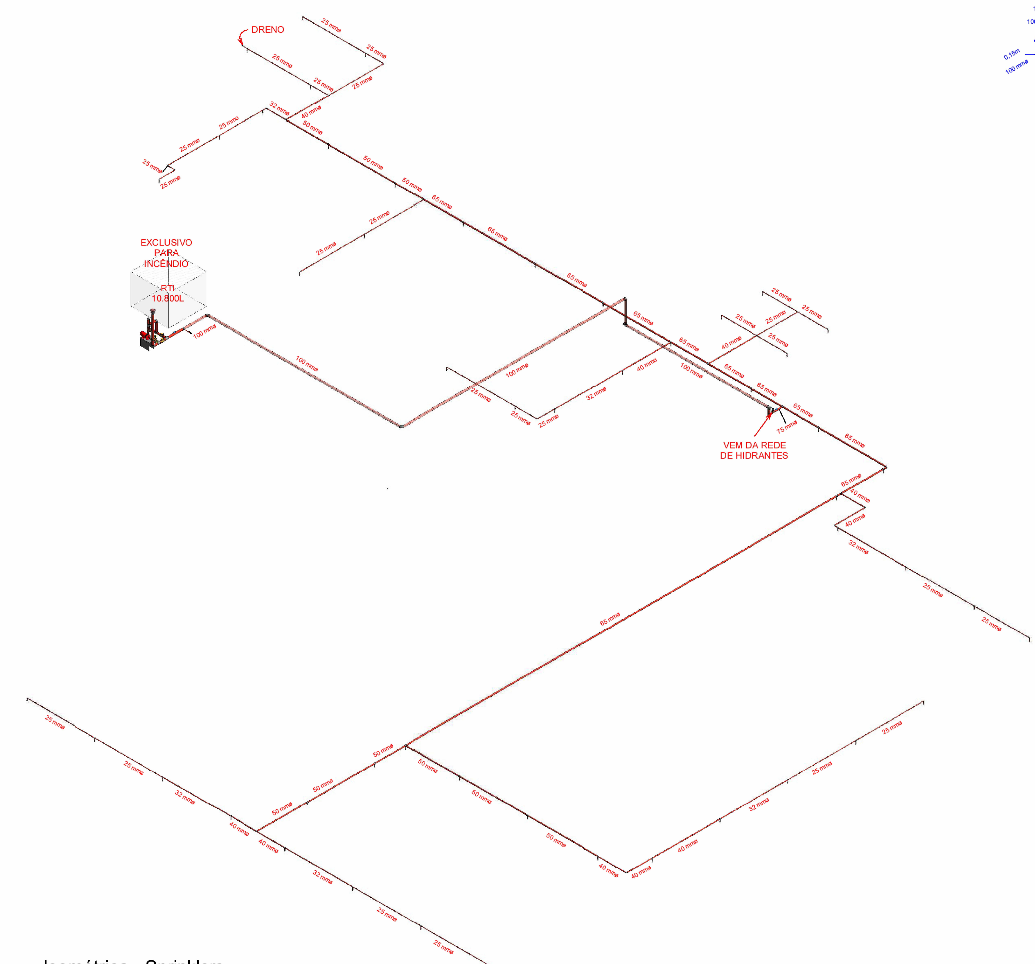
2 Isométrica - Sprinklers
