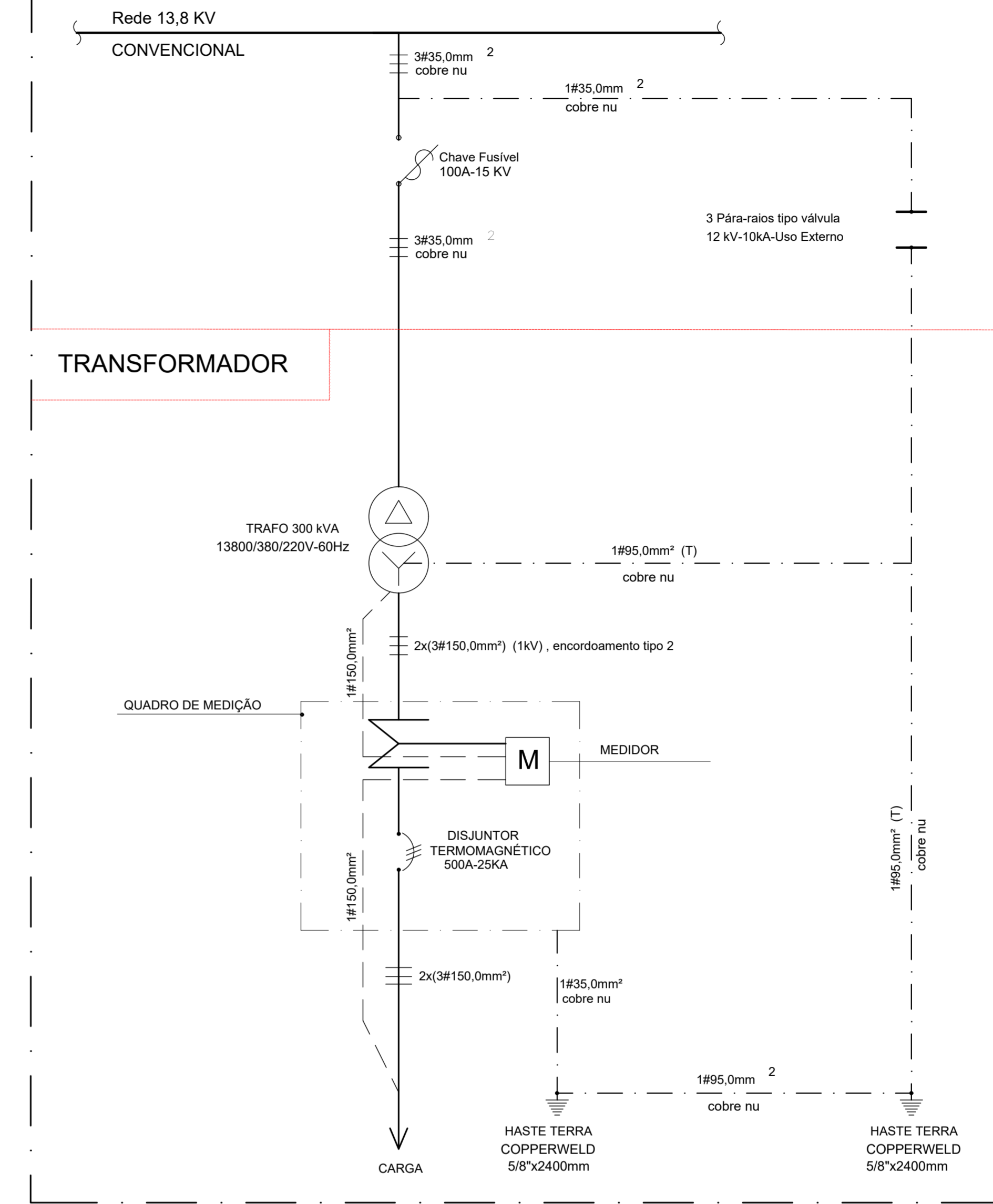
03 SUBESTAÇÃO AÉREA 13,8 kV - 300 kVA DIAGRAMA UNIFILAR GERAL ESCALA: SEM ESCALA
