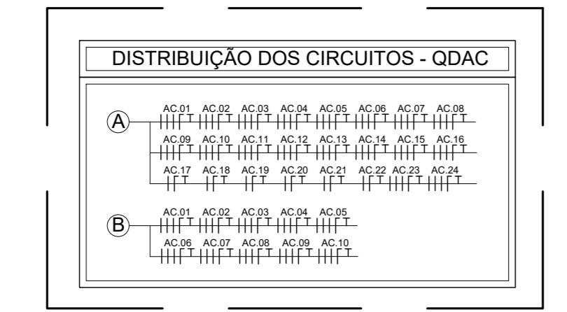
02 ENERGIA ELÉTRICA PARA AR CONDICIONADO DISTRIBUIÇÃO DOS CIRCUITOS QDAC ESCALA: 1/75
