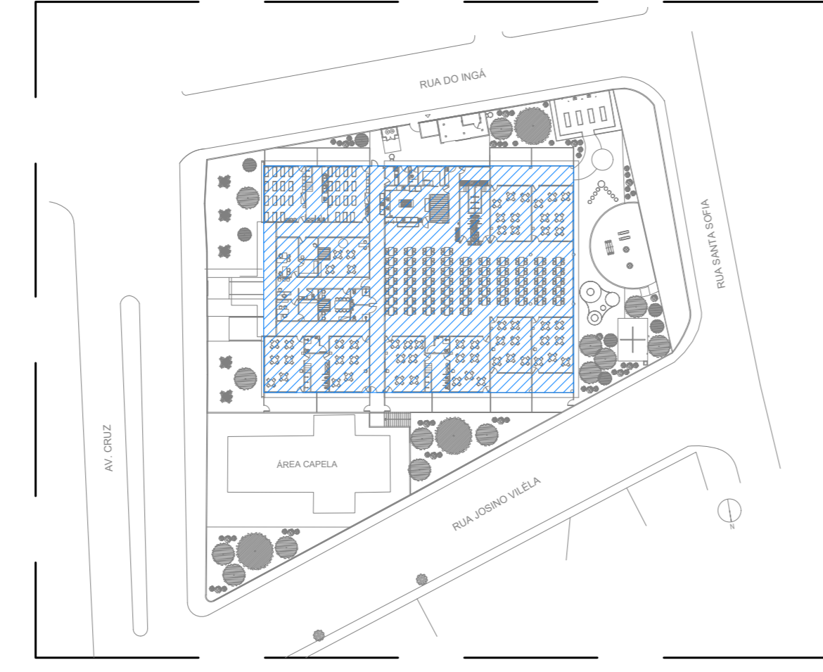
03 ENERGIA COMERCIAL - AR CONDICIONADO PLANTA BAIXA DE LOCAÇÃO ESCALA: 1/75
