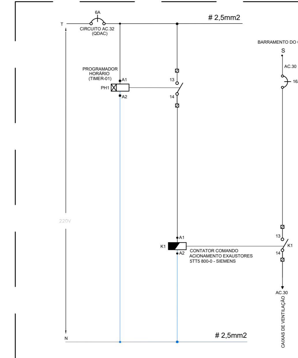
04 ENERGIA ELÉTRICA PARA AR CONDICIONADO DIAGRAMAS DE COMANDO QUADRO QDAC ESCALA: SEM ESCALA
