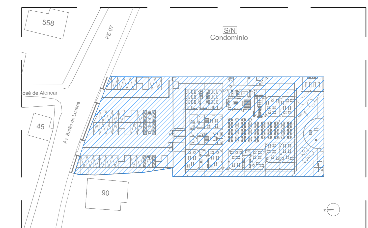
ENERGIA COMERCIAL - ILUMINAÇÃO 02 PLANTA BAIXA DE LOCAÇÃO ESCALA: 1/750
