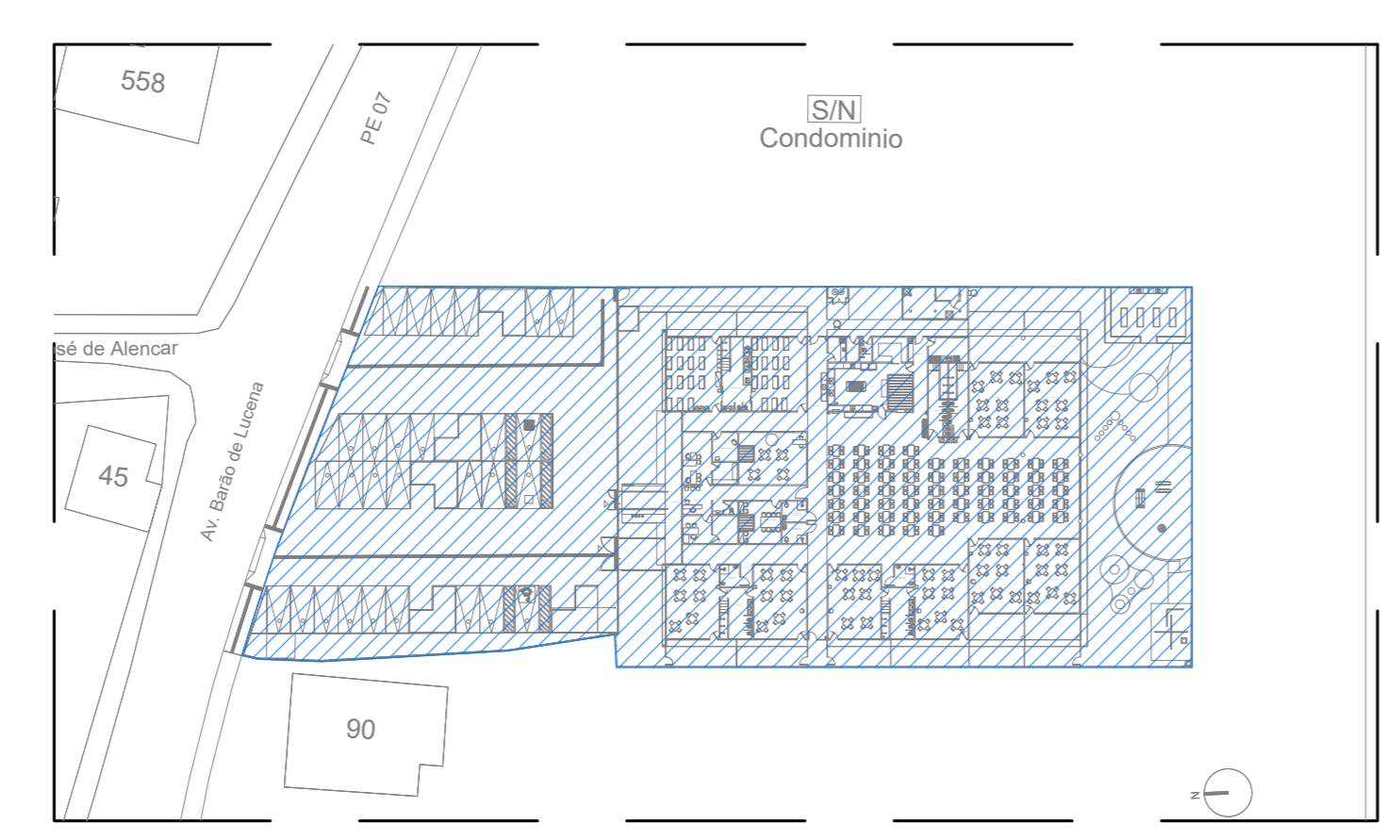
03 ENERGIA COMERCIAL - AR CONDICIONADO PLANTA BAIXA DE LOCAÇÃO ESCALA: 1/75
