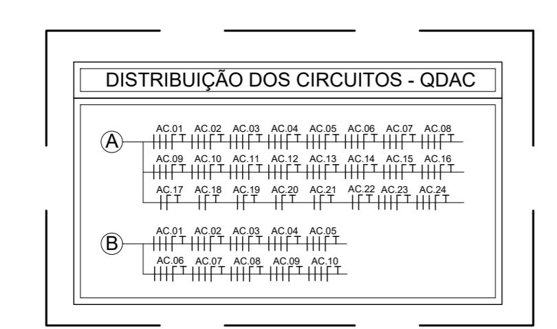
02 ENERGIA ELÉTRICA PARA AR CONDICIONADO DISTRIBUIÇÃO DOS CIRCUITOS QDAC ESCALA: 1/75
